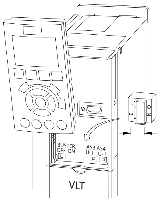
图 4.10 端子 53 和 54 的开关位置
