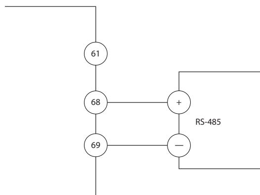
图 4.11 串行通讯接线图
