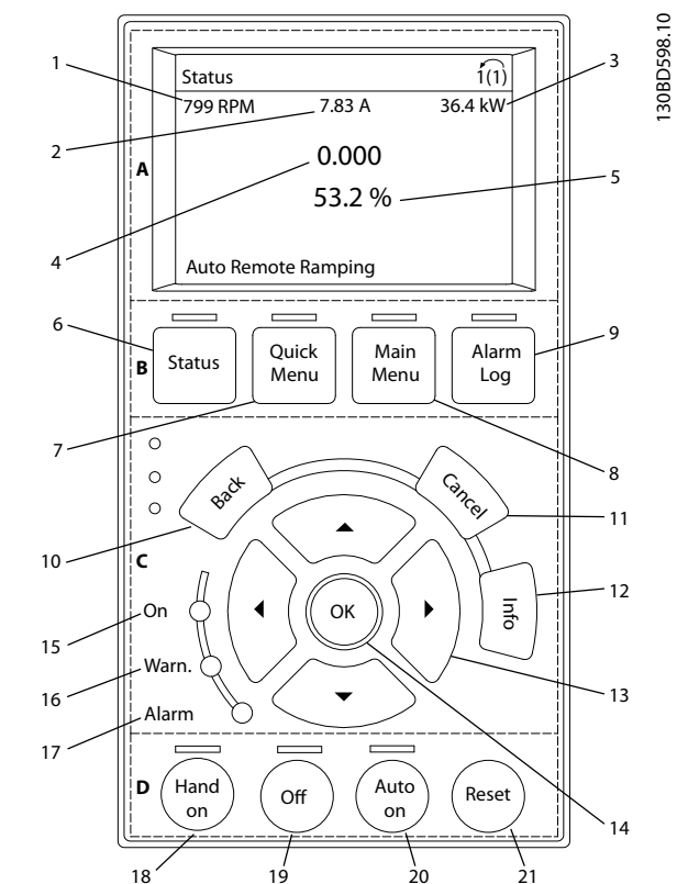
图 5.1 图形化本地控制面板 (GLCP)
