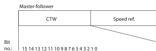
Ilustração 3.55 Control Word
