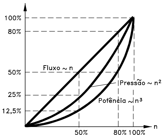
Ilustração 2.2 Leis de afinidade para bombas centrífugas
