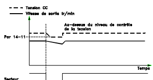
Illustration 3.41 Sauvegarde cinétique, brève panne de secteur. Fonctionnement tant que l'énergie du système le permet
