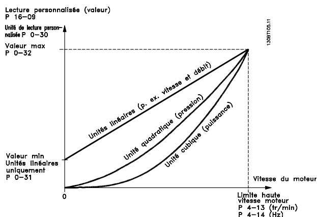
Illustration 3.3 Lect.paramétr.
