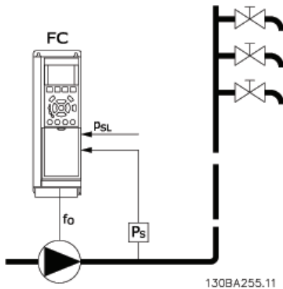
Illustration 3.57 Légende : FC = variateur de fréquence ; fo = sortie fréquence ; Ps=P système ; PsL=P consigne
