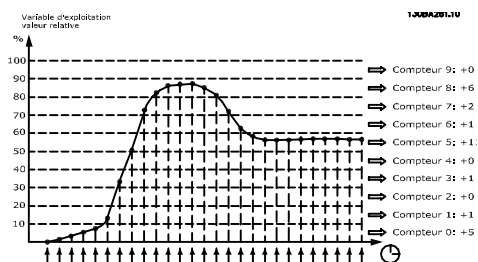
Illustration 3.69 Heure et valeurs relatives
