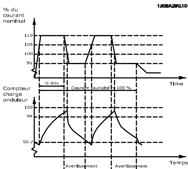
Illustration 3.44 Courant de sortie en condition de surcharge
