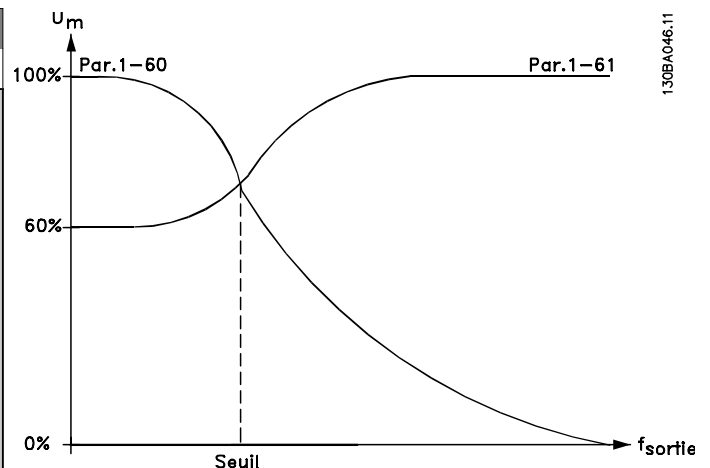
Illustration 3.10 Comp.charge à vit.basse
