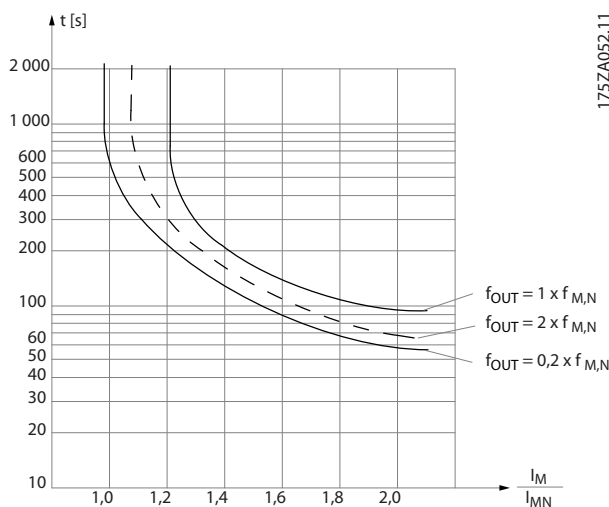
Illustration 3.12 Protection du moteur contre la surcharge
