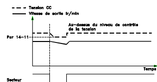
Illustration 3.47 Sauvegarde cinétique, brève panne de secteur. Fonctionnement tant que l'énergie du système le permet
