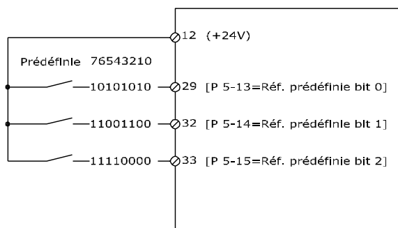
Illustration 3.14 Schéma de références prédéfinies
