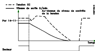
Illustration 3.40 Rampe de décélération ctrlée, défaut secteur plus long. Décélération tant que l'énergie du système le permet, puis mise en roue libre du moteur
