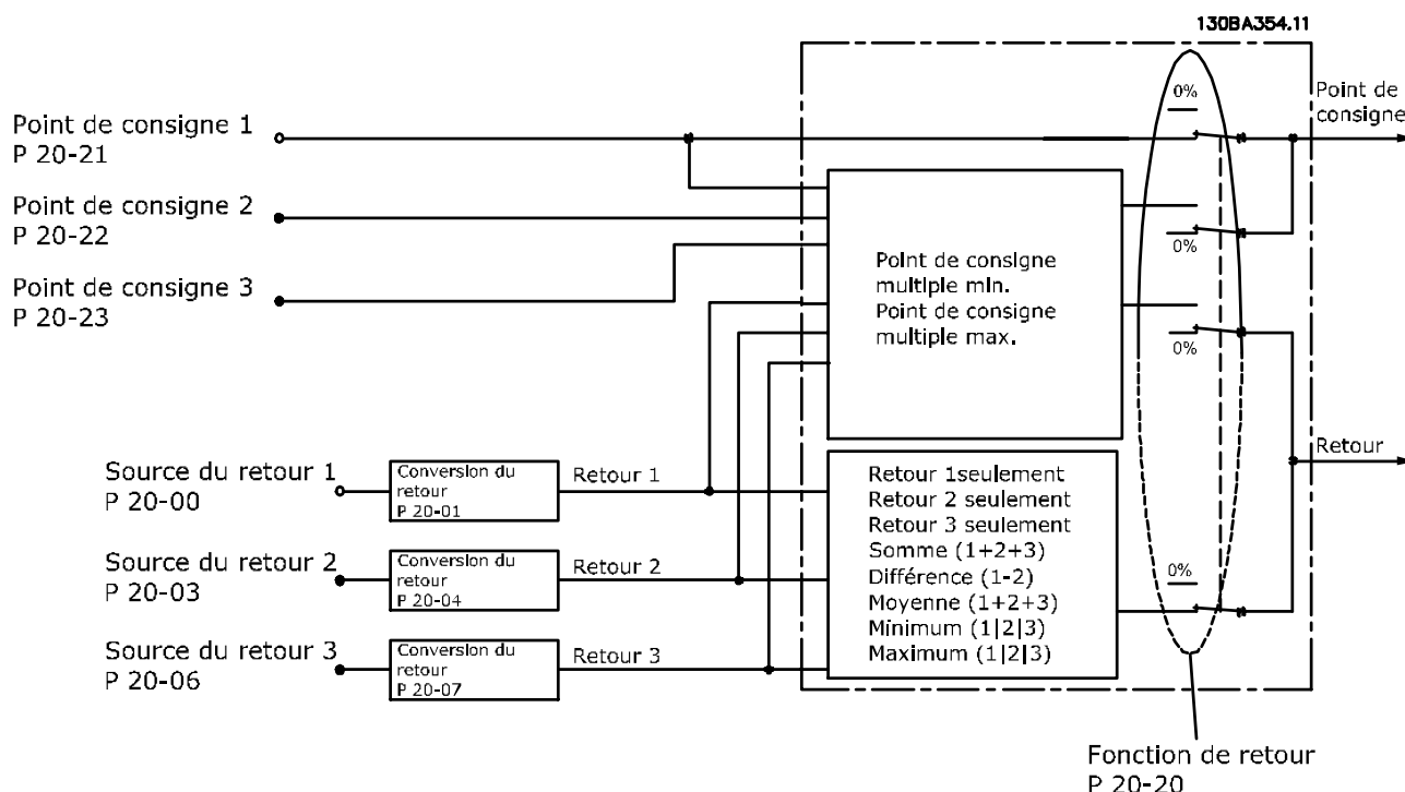
Illustration 3.51 Signal d'entrée du contrôleur PID en boucle fermée
