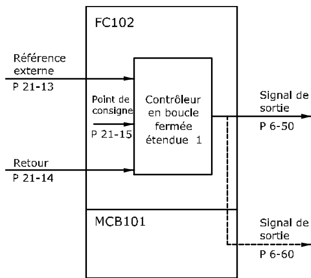
Illustration 3.53 Réf/ret PID ét. 1
