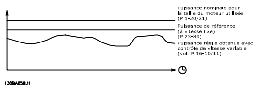
Illustration 3.70 Comparaison entre la puissance de référence et la puissance réelle
