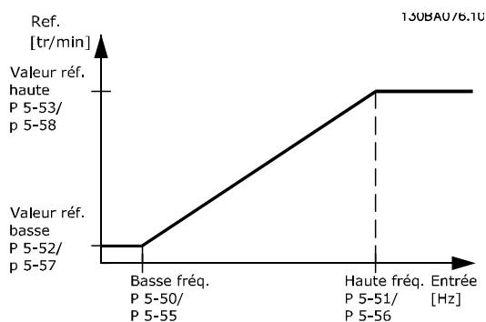
Illustration 3.27 Entrée impulsions
