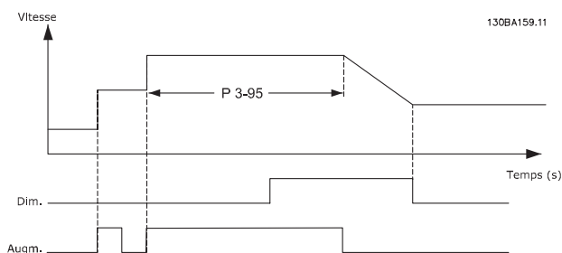
Illustration 3.22 Cas n° 2 de retard de rampe
