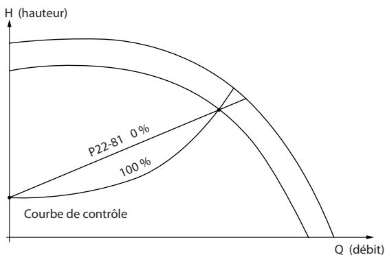
Illustration 3.62 Approx. courbe linéaire-quadratique
