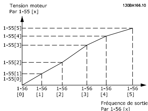
Illustration 3.9 Caractéristique U/f
