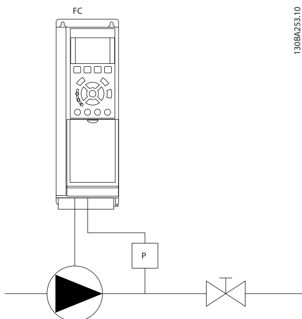
Illustration 3.55 Schéma de Détection d'absence de débit
