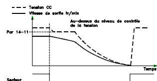
Illustration 3.48 Sauvegarde cinétique, panne secteur plus longue. Le moteur est en roue libre dès que l'énergie du système est trop basse
