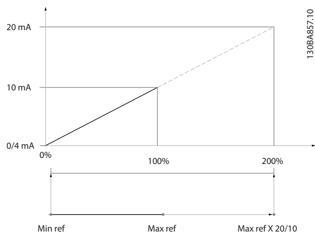
Illustration 3.35 Exemple 3
