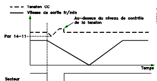
Illustration 3.39 Rampe de décélération ctrlée - Bref défaut secteur. Décélération jusqu'à l'arrêt, puis accélération jusqu'à la référence
