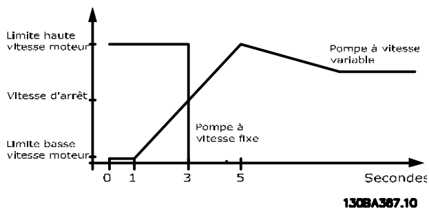
Illustration 3.83 Seuil d'arrêt
