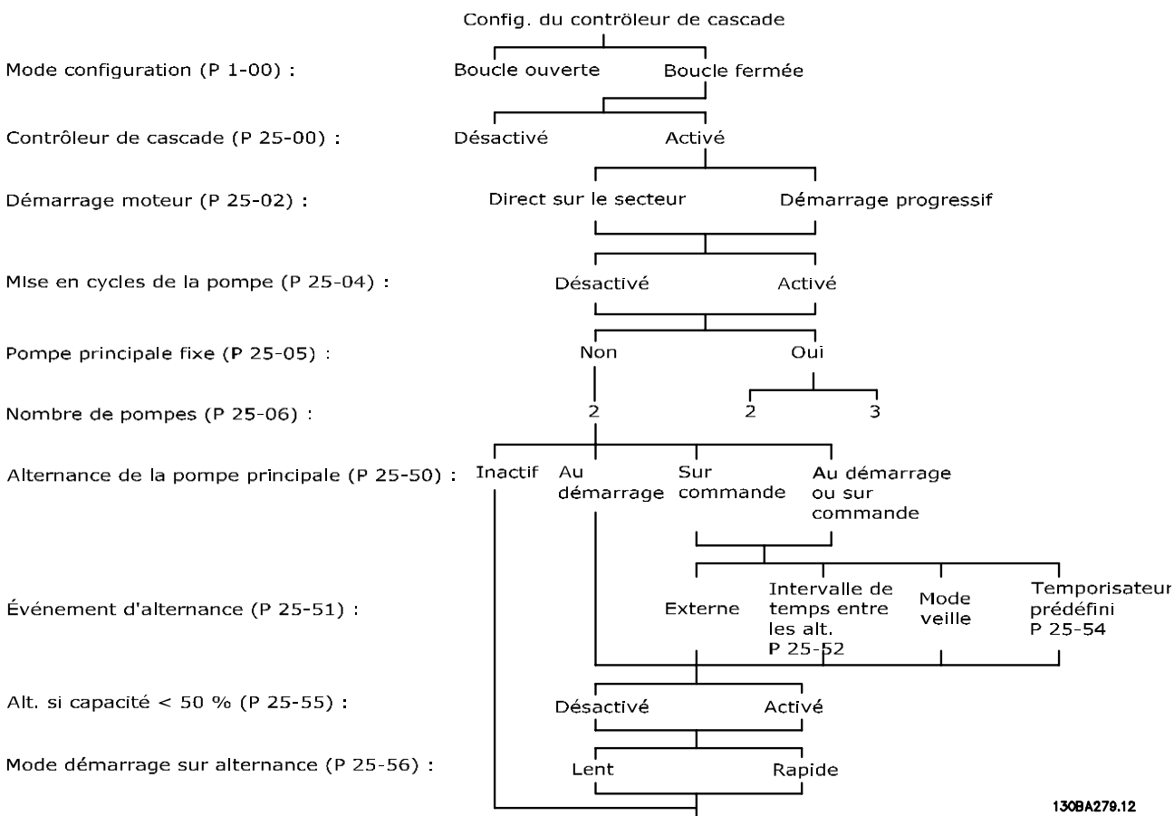
Illustration 3.71 Process de configuration du contrôleur de cascade
