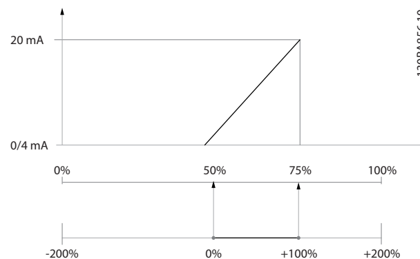
Illustration 3.34 Exemple 2
