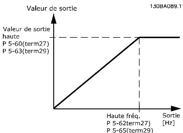
Illustration 3.28 Sortie impulsions
