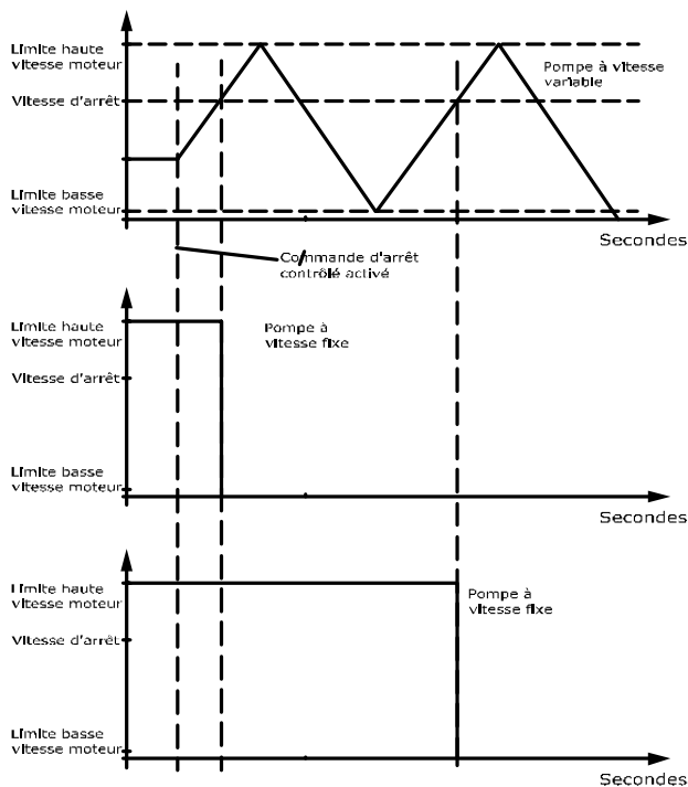
Illustration 3.84 Vitesse d'arrêt
