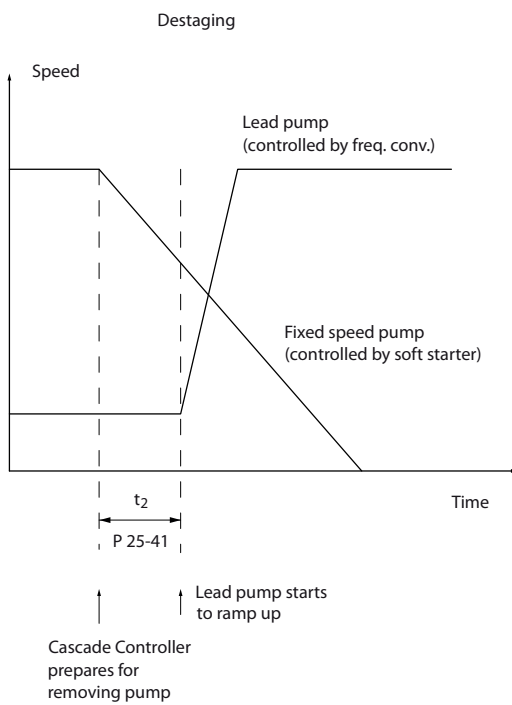
Illustration 3.81 Arrêt
