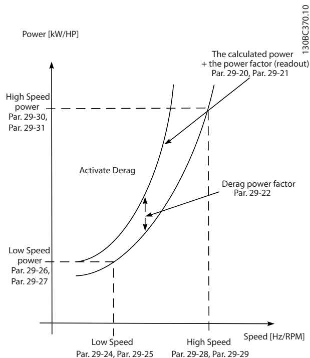
Illustration 3.90 Régl.puiss. décolmatage
