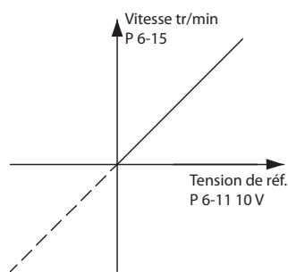
Illustration 1.9 Référence potentiomètre
