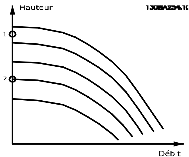
Illustration 3.56 Graphique de Détection d'absence de débit
