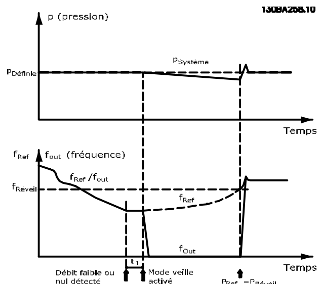
Illustration 3.60 Système de suralimentation sans retour de la pression
