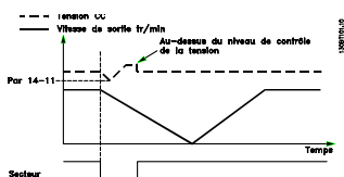
Illustration 3.45 Rampe de décélération ctrlée - Bref défaut secteur. Décélération jusqu'à l'arrêt, puis accélération jusqu'à la référence
