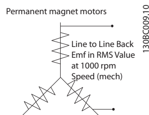
Illustration 3.7 Définitions des paramètres machine du FCEM des moteurs à aimant permanent
