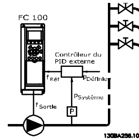
Illustration 3.59 Système avec retour de la pression
