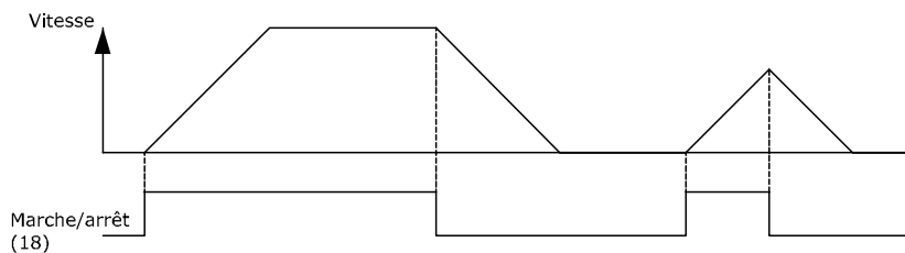
Illustration 1.6 Marche/arrêt
