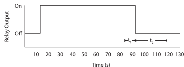
Illustration 3.29 Exemple de fonction de sortie
