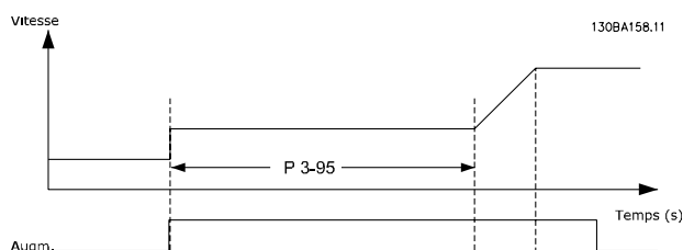
Illustration 3.21 Cas n° 1 de retard de rampe
