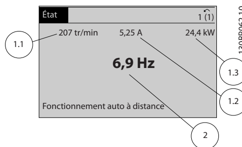
Illustration 2.11 Écran d'état II
