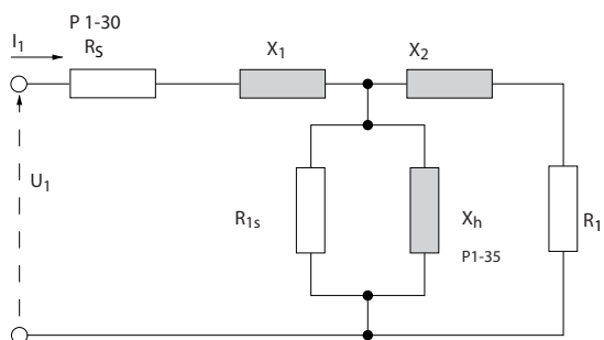
Illustration 3.4 Diagramme d'équivalence moteur pour un moteur asynchrone
