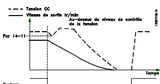
Illustration 3.46 Rampe de décélération ctrlée, défaut secteur plus long. Décélération tant que l'énergie du système le permet, puis mise en roue libre du moteur
