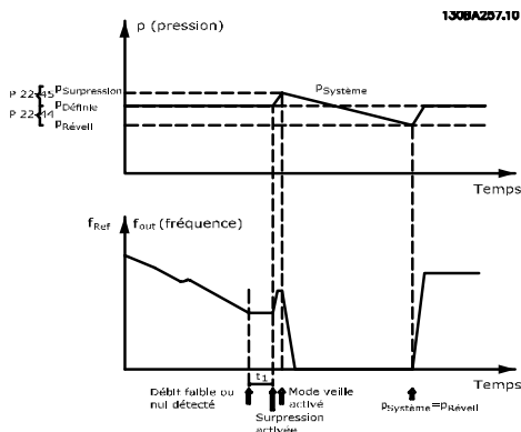
Illustration 3.58 Système d'appoint avec retour de pression
