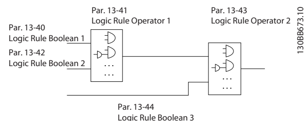
Illustration 3.38 Règles de Logique
