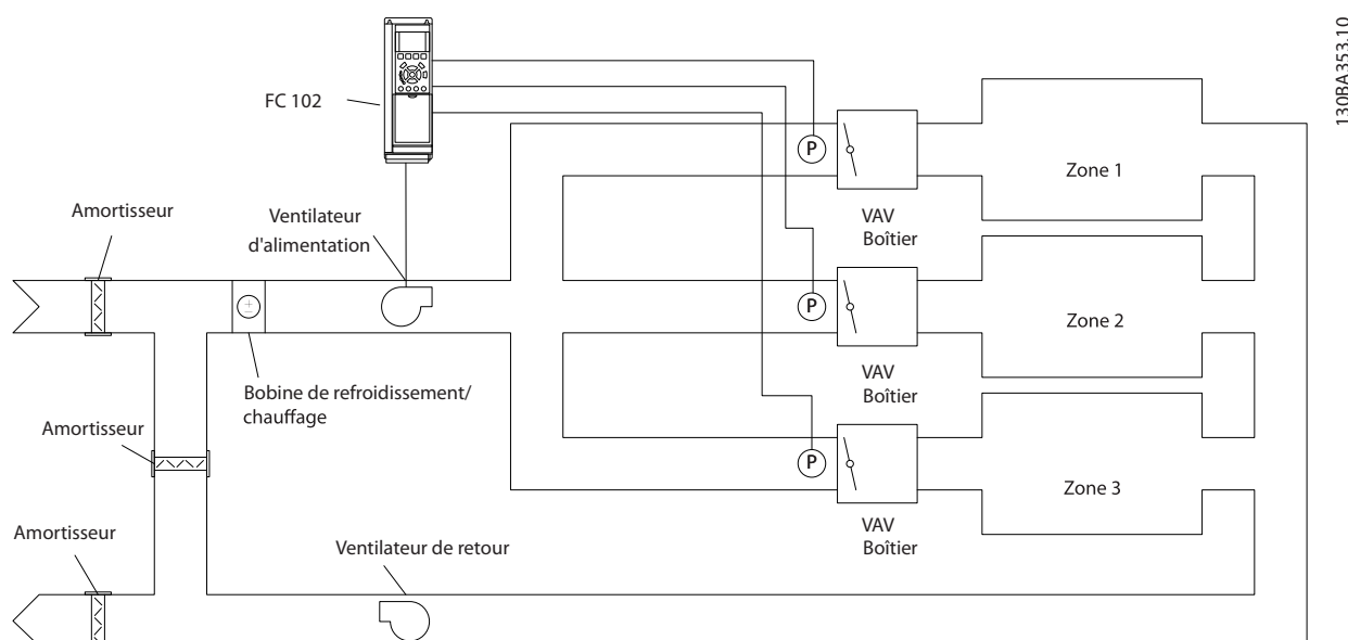
Illustration 3.52 Schéma d'application multizones
