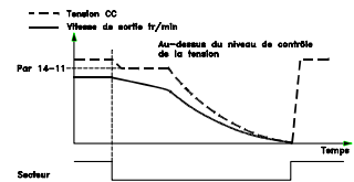
Illustration 3.42 Sauvegarde cinétique, panne secteur plus longue. Le moteur est en roue libre dès que l'énergie du système est trop basse
