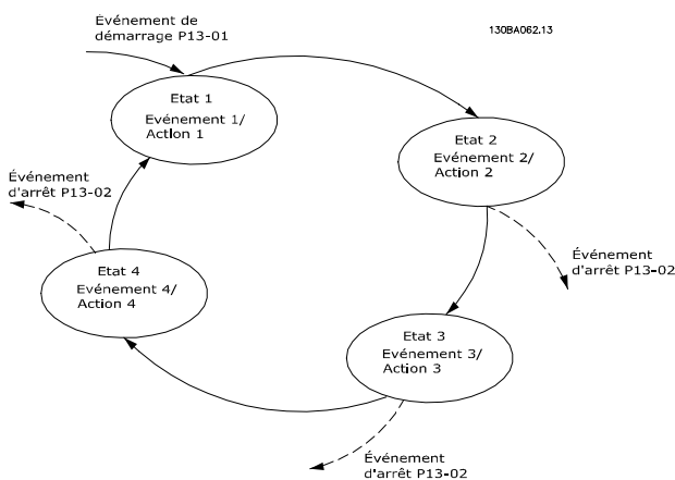
Illustration 3.36 Actions Événement logique avancé
