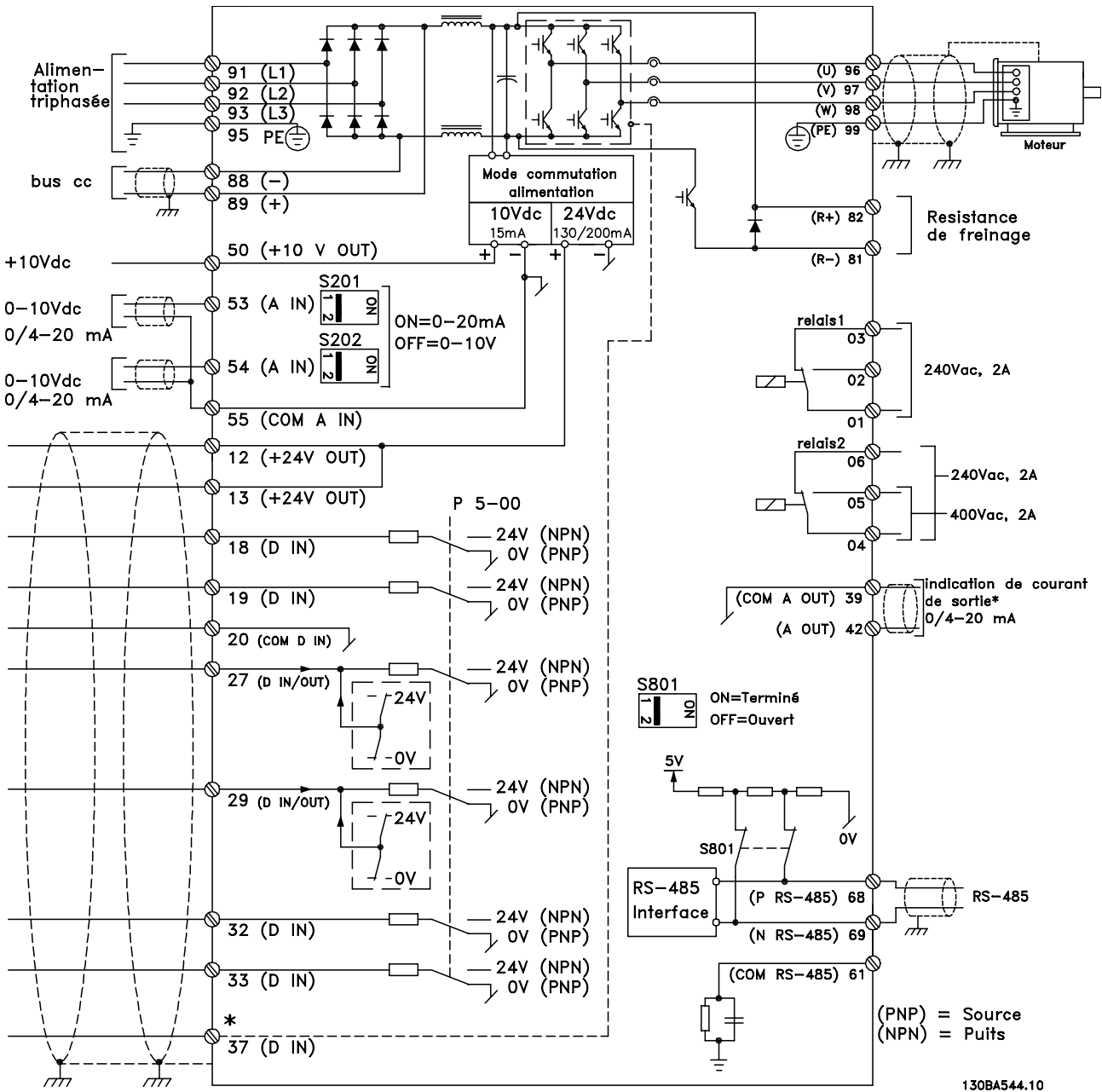
Illustration 1.2 Dessin schématique du câblage de base
