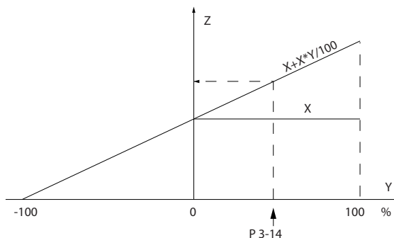
Illustration 3.16 Référence réelle
