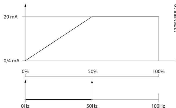
Illustration 3.33 Exemple 1
