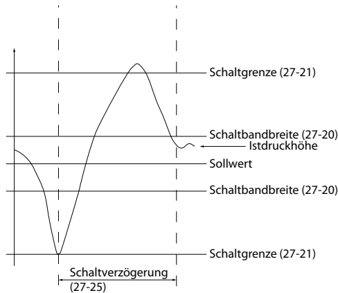
Abbildung 3.75 Schaltverzögerung
