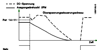
Abbildung 3.42 Geregelte Rampe ab, längerer Netzausfall. Rampe ab, solange die Energie im System dies zulässt; anschließend schaltet der Frequenzumrichter den Motor in den Freilauf.
