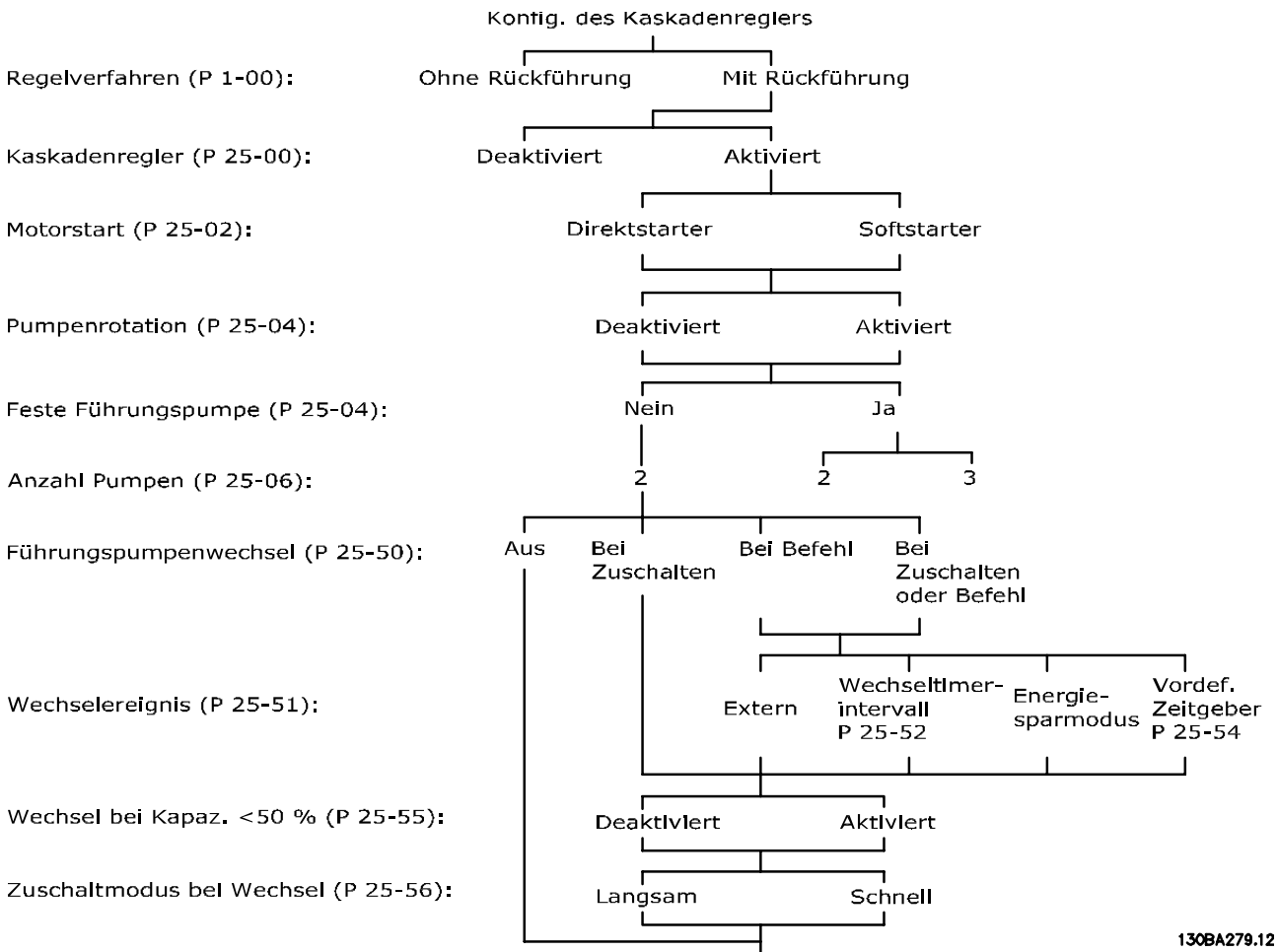
Abbildung 3.68 Kaskadenregler – Beispielkonfiguration
