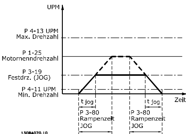
Abbildung 3.18 Rampenzeit JOG
