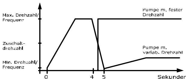
Abbildung 3.79 Zuschaltsschwelle
