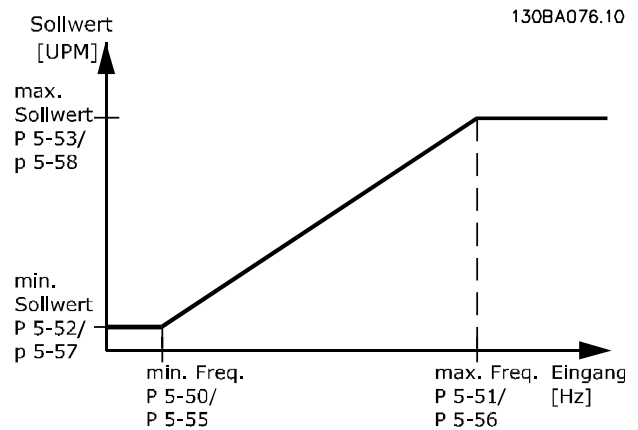
Abbildung 3.27 Pulseingänge
