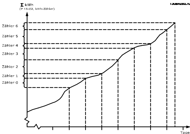
Abbildung 3.64 Energieprotokoll-Diagramm
