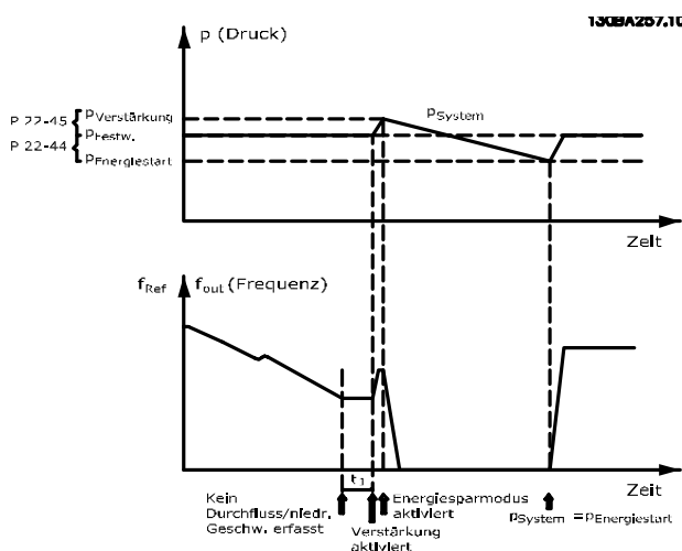
Abbildung 3.56 Boost-System mit Druck-Istwert
