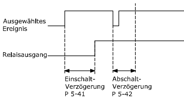
Abbildung 3.26 Aus Verzög., Relais
