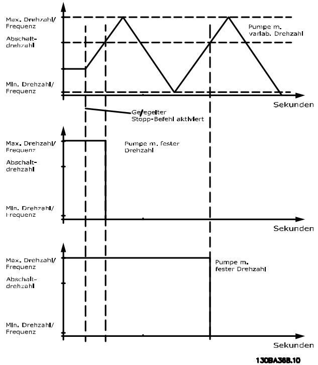
Abbildung 3.81 Abschalt-drehzahl
