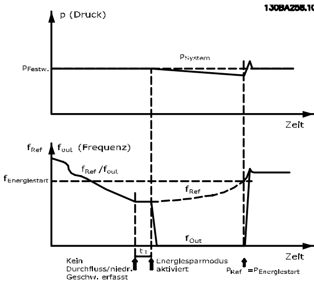
Abbildung 3.58 Boost-System ohne Druck-Istwert
