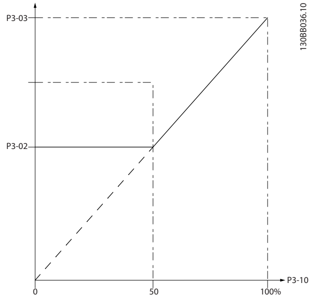
Abbildung 3.13 Festsollwert
