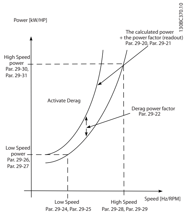
Abbildung 3.87 Rückspüleleistungsanpassung
