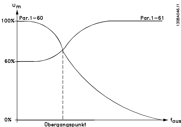
Abbildung 3.10 Lastausgleich tief
