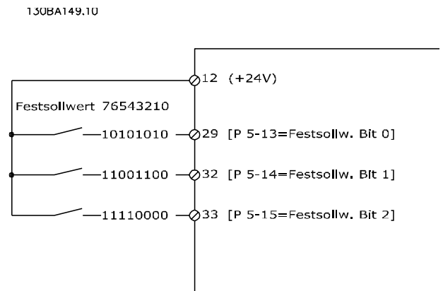
Abbildung 3.14 Festsollwertschema
