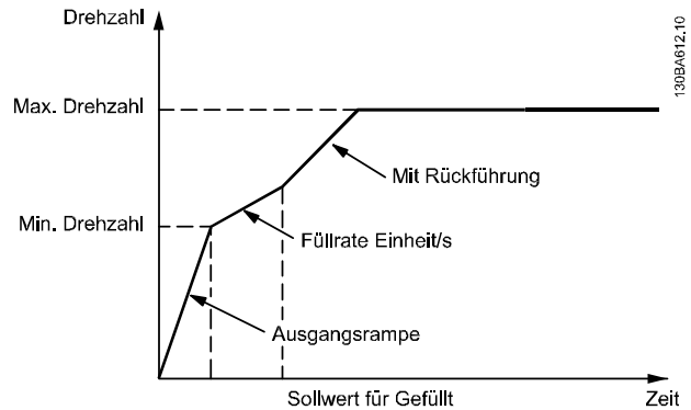
Abbildung 3.85 Vertikales Rohrsystem
