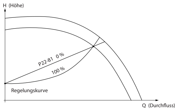
Abbildung 3.60 Quadratisch-lineare Kurvennäherung
