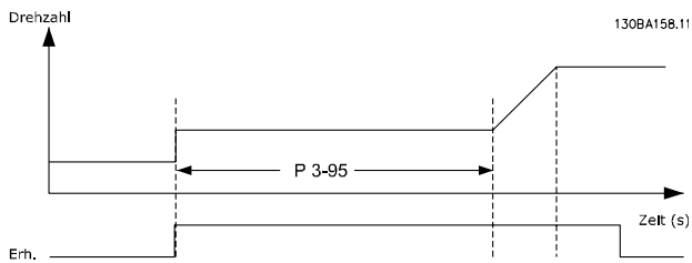
Abbildung 3.21 Rampenverzögerung Fall 1
