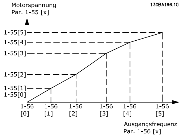
Abbildung 3.9 U/f-Kennlinie
