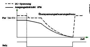
Abbildung 3.44 Kinetischer Speicher, längerer Netzausfall. Der Frequenzumrichter schaltet den Motor in den Freilauf, sobald die Energie im System zu gering ist.
