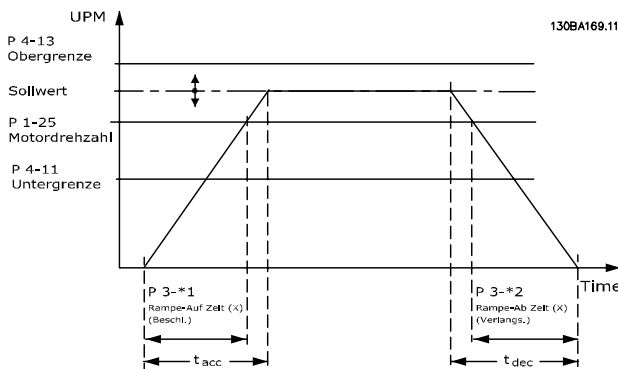
Abbildung 3.17 Rampe 1
