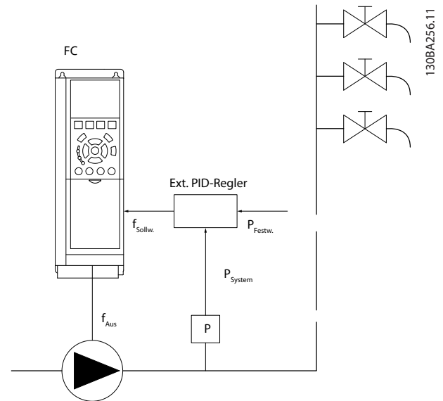
Abbildung 3.57 System mit Druck-Istwert
