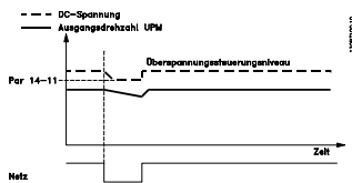
Abbildung 3.43 Kinetischer Speicher, kurzer Netzausfall. Weiterlaufen, solange die Energie im Systems dies zulässt.
