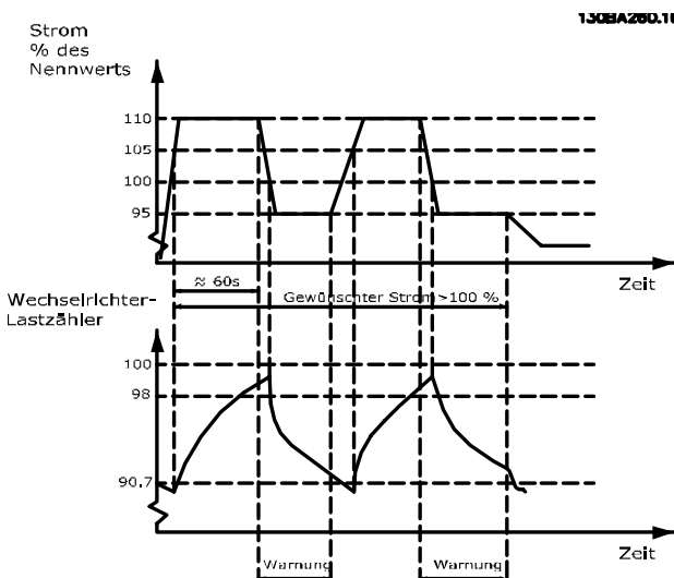
Abbildung 3.46 Ausgangsstrom bei Überlastbedingung
