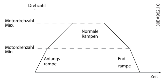
Abbildung 3.19 Ausgangs- und Endrampenzeit
