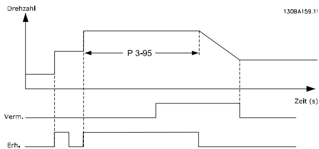
Abbildung 3.22 Rampenverzögerung Fall 2
