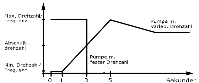
Abbildung 3.80 Abschaltsschwelle
