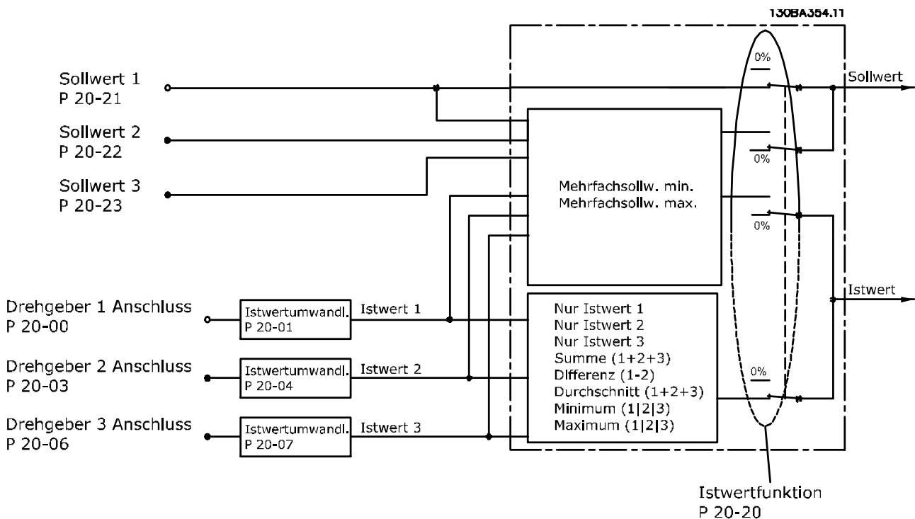
Abbildung 3.49 Eingangssignale des PID-Reglers mit Rückführung
