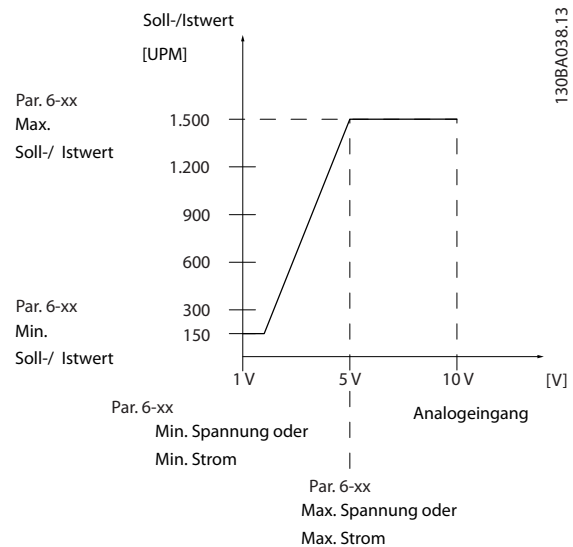
Abbildung 3.30 Signalausfallbedingungen
