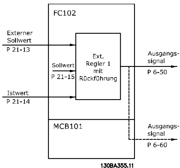
Abbildung 3.51 Erw. PID Soll-/Istw. 1
