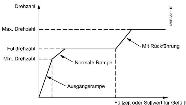
Abbildung 3.84 Horizontales Rohrsystem
