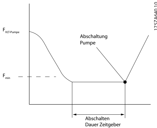
Abbildung 3.76 Abschaltfunktionszeit
