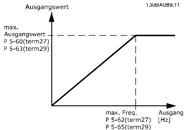
Abbildung 3.28 Pulsausgänge
