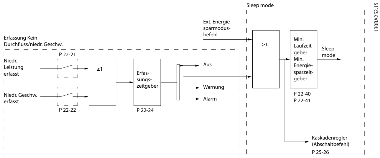
Abbildung 3.52 Signalflussdiagramm
