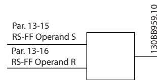
Abbildung 3.38 Reset/Set Flip Flops
