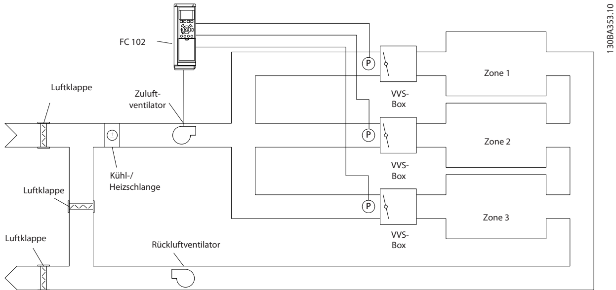
Abbildung 3.50 Anwendungsschema für mehrere Zonen
