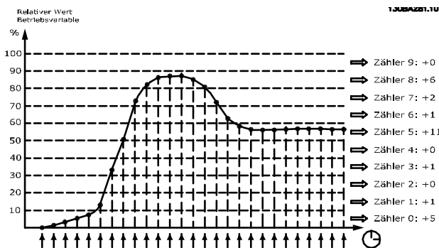
Abbildung 3.66 Zeit und Relativwerte
