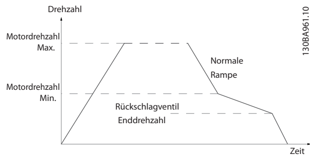
Abbildung 3.20 Rückschlagventil-Rampe
