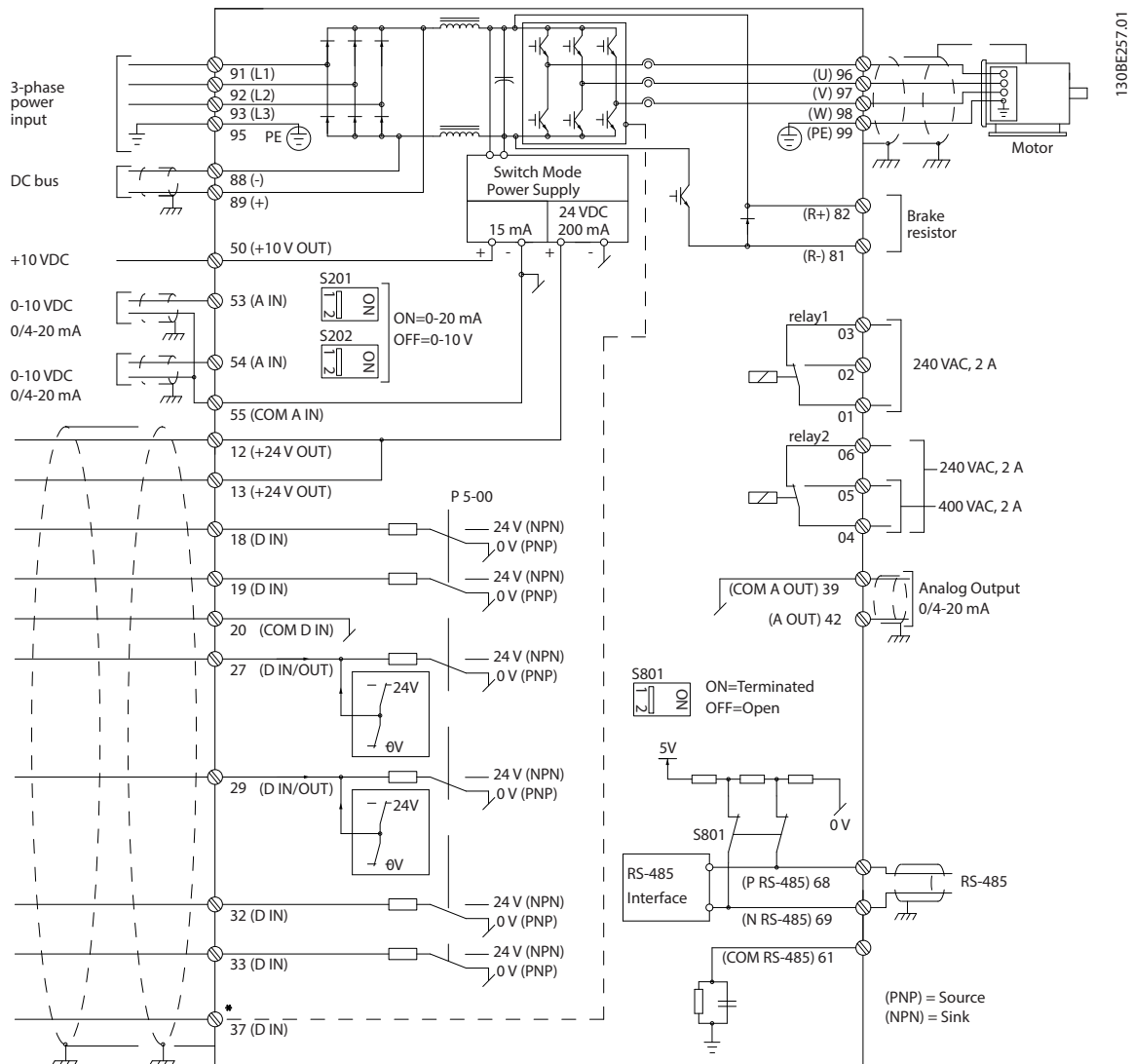
Abbildung 1.2 Anschlussdiagramm des Grundgeräts
