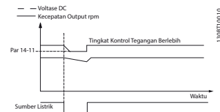
Ilustrasi 3.52 Cadangan Kinetik, Kegagalan Akibat Aliran Listrik Mati Singkat.
