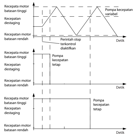
Ilustrasi 3.92 Kecepatan Destaging
