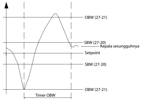
Ilustrasi 3.86 Waktu OBW
