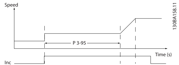
Ilustrasi 3.25 Penundaan Ramp Kasus 1
