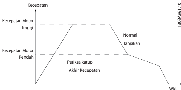
Ilustrasi 3.24 Periksa Ramp Katup
