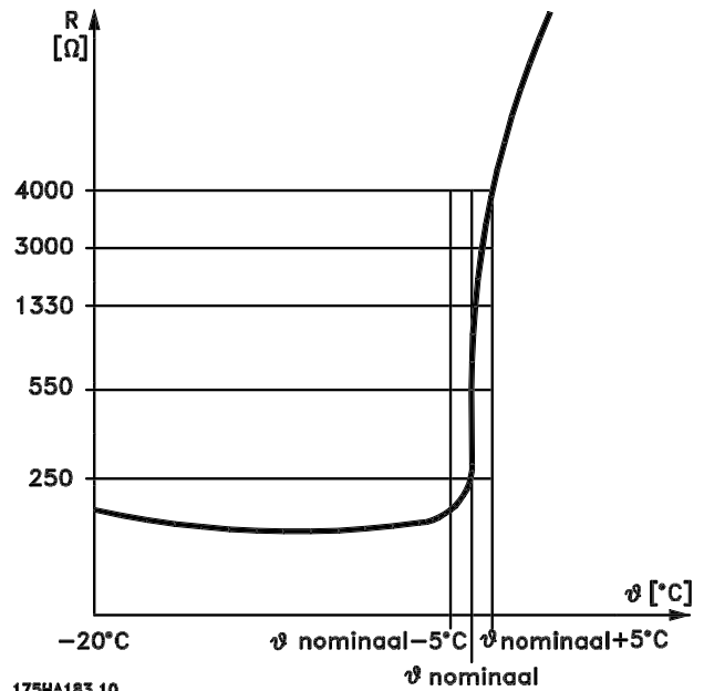
175HA183.10 Ilustrasi 3.12 Profil PTC
