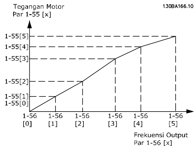
Ilustrasi 3.9 Karakteristik U/f
