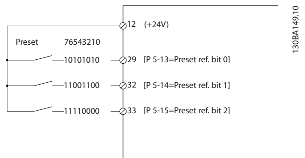
Ilustrasi 3.18 Skema Referensi Preset
