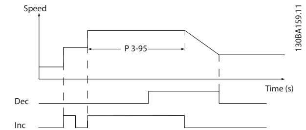
Ilustrasi 3.26 Penundaan Ramp Kasus 2
