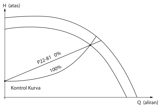
Ilustrasi 3.71 Perkiraan Kurva Linear-Kuadrat
