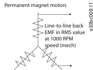
Ilustrasi 3.7 Batasan Parameter Mesin Back EMF Motor PM
