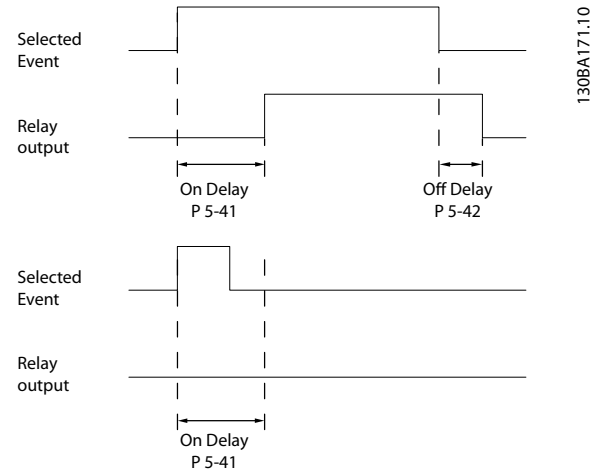
Ilustrasi 3.29 Tunda Aktif, Relai
