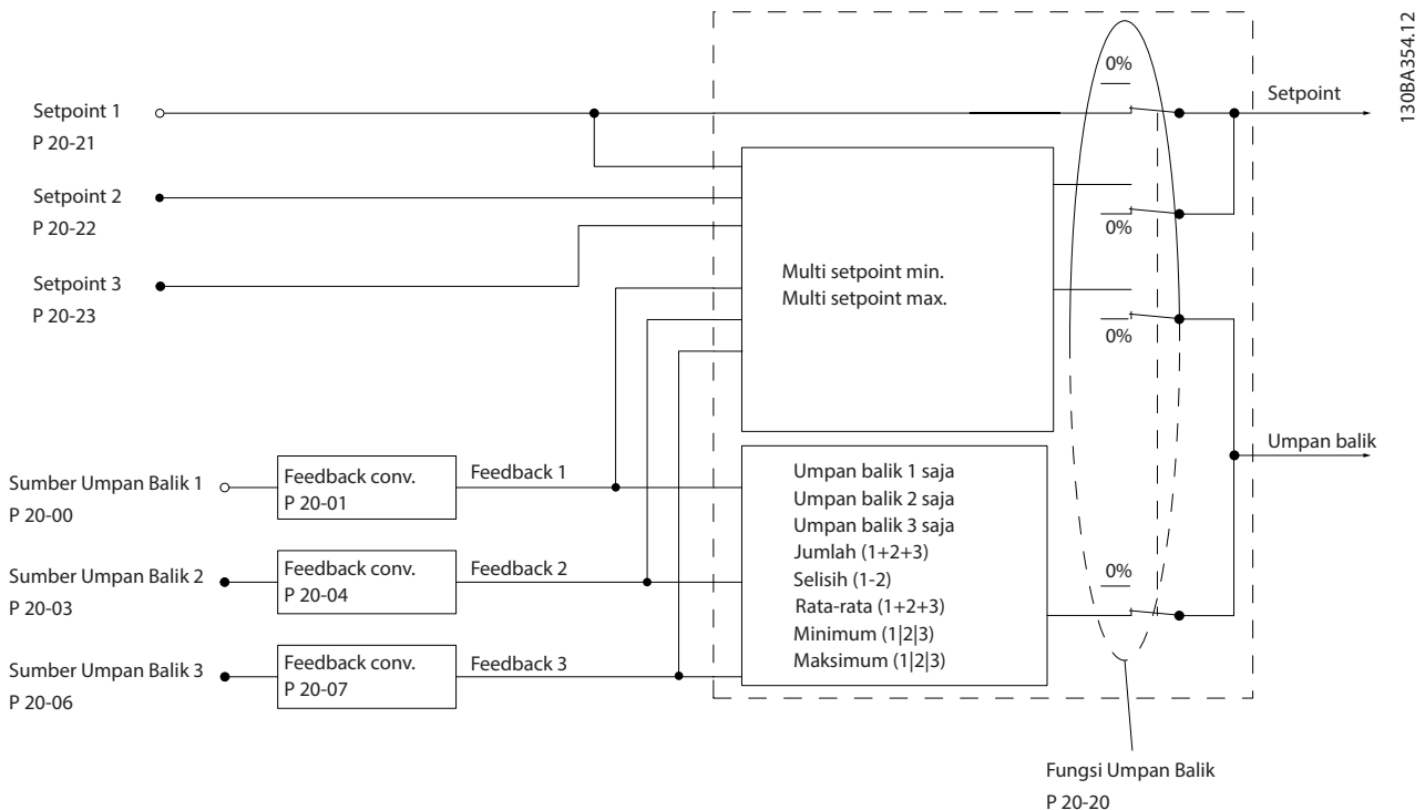
Ilustrasi 3.60 Sinyal Input dalam Kontroler PID Simpall tertutup
