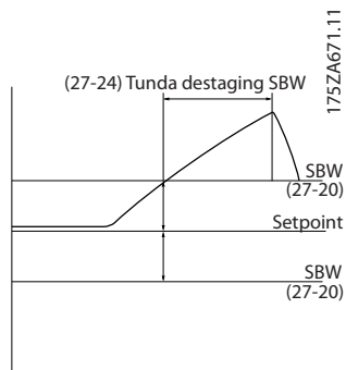
Ilustrasi 3.98 Tunda Destaging SBW
