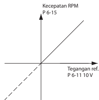
Ilustrasi 1.9 Referensi potensiometer
