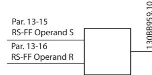
Ilustrasi 3.42 Flip Flop Reset/Set
