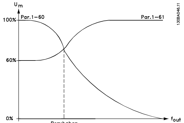
Ilustrasi 3.10 Kompensasi Beban Kecepatan Rendah
