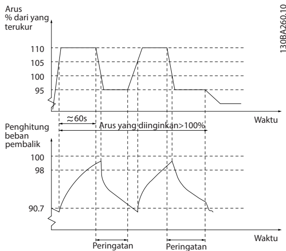
Ilustrasi 3.55 Arus Output dalam Kondisi Kelebihan Beban
