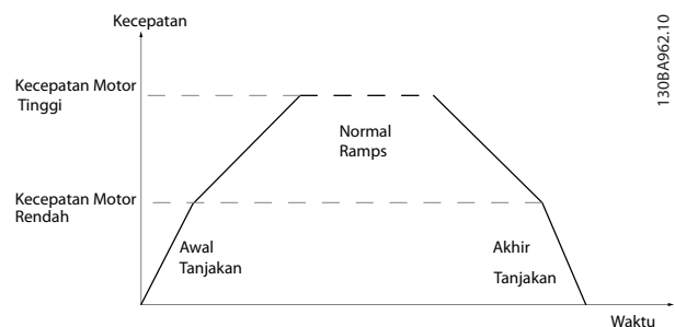
Ilustrasi 3.23 Waktu R Awal dan Final
