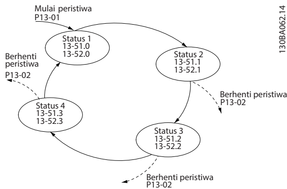
Ilustrasi 3.40 Tindakan Peristiwa Smart Logic
