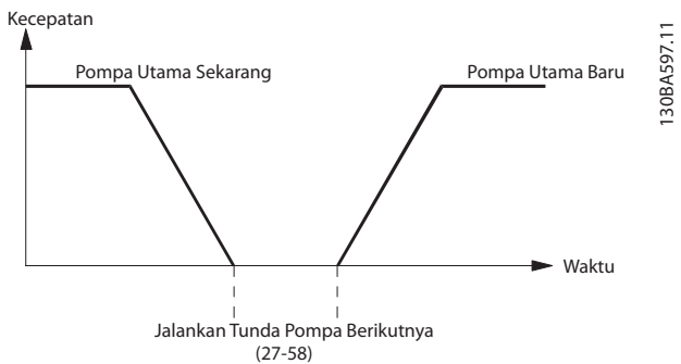
Ilustrasi 3.109 Tunda Pengoperasian Pompa Selanjutnya
