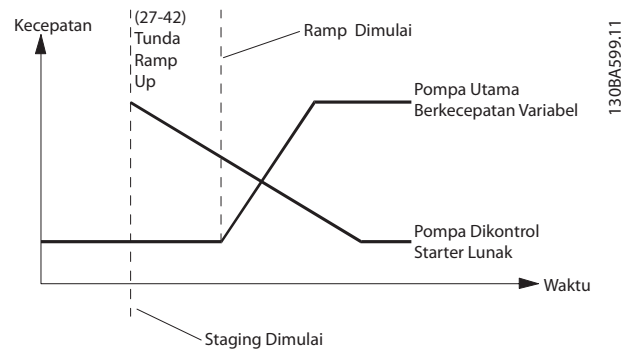
Ilustrasi 3.106 Tunda Akselerasi
