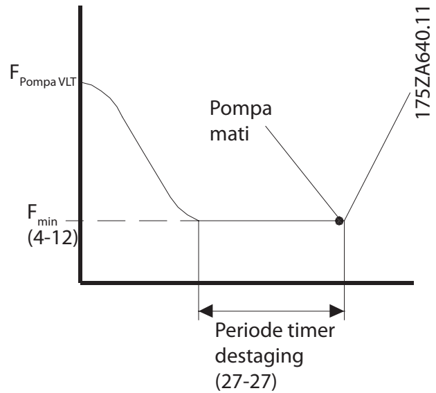
Ilustrasi 3.87 Waktu Fungsi Destaging
