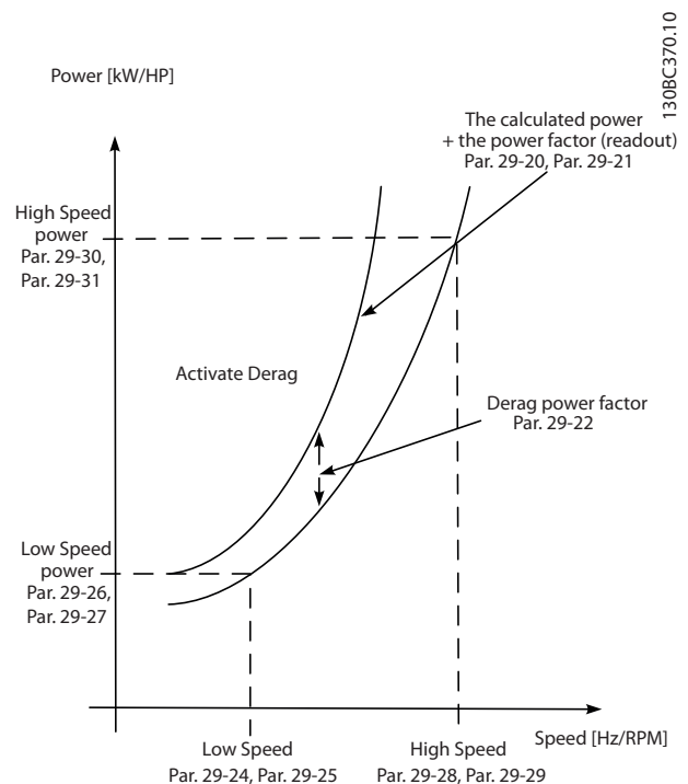
Ilustrasi 3.113 Penalaan Daya Derag
