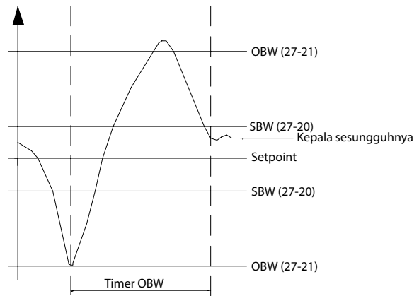
Ilustrasi 3.99 Waktu OBW
