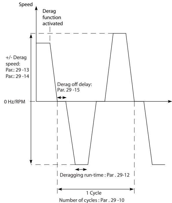
Ilustrasi 3.112 Fungsi Derag
