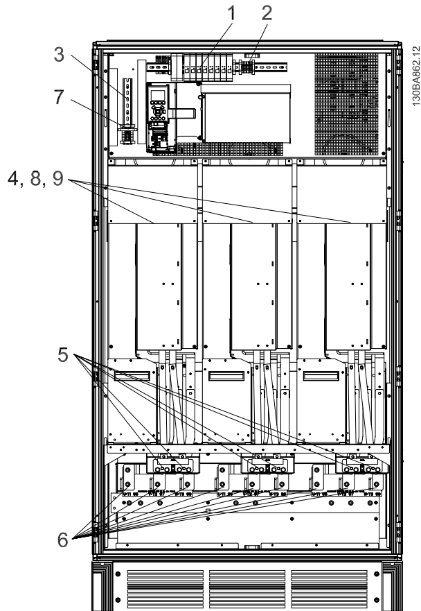
Disegno 3.47: Armadio inverter, telaio di taglia F2 e F4
