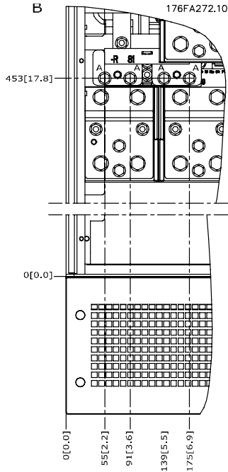
Ilustração 3.13: Posições das conexões de energia para os gabinetes metálicos IP21 (NEMA Tipo 1) e IP54 (NEMA Tipo 12) (detalhe B)
