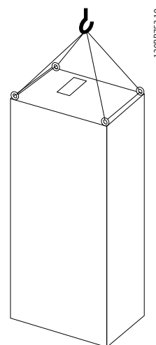
Bild 3.1 Rekommenderad lyftmetod, kapsling F8.
