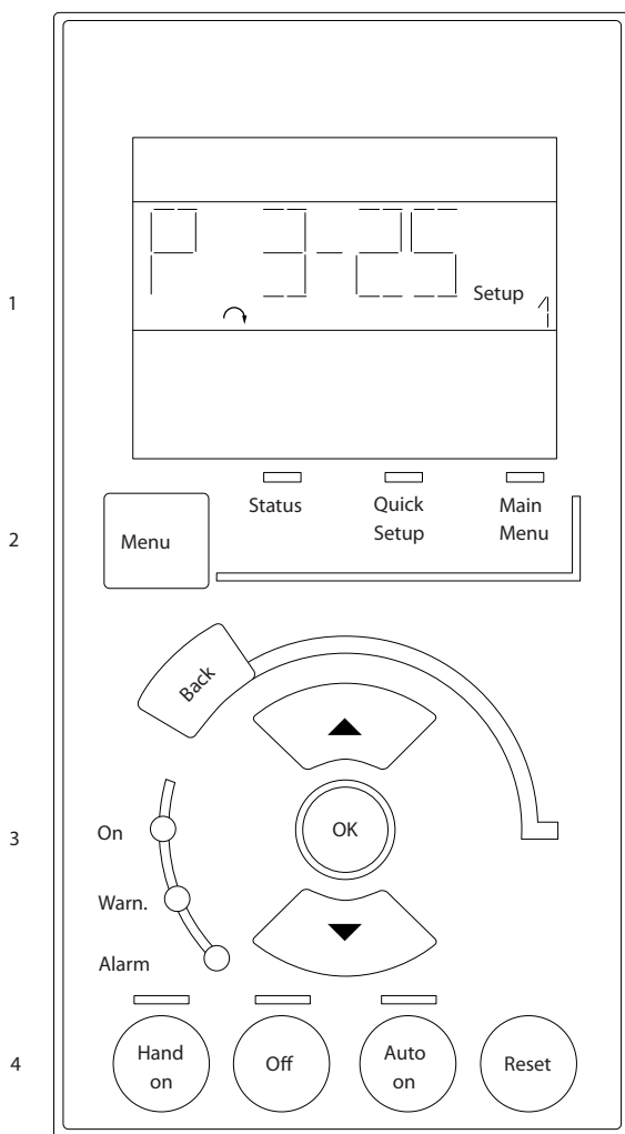
Ilustração 5.1 LCP Numérico (NLCP)
