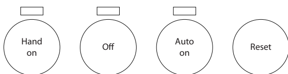
Ilustração 5.5 Teclas operacionais do LCP numérico (NLCP)
