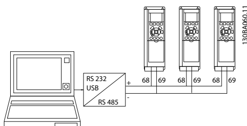
Ábra 5.9 Kapcsolási példa
