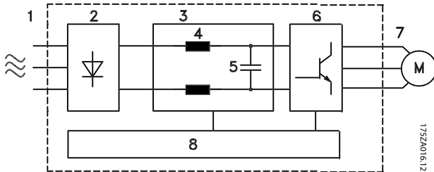
Afbeelding 1.4 Blokschema frequentieomvormer
