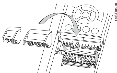
Afbeelding 2.30 Stuurklemmen verwijderen
