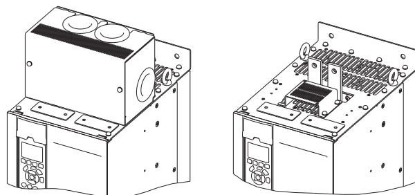
Εικόνα 2.32 Διαμοιρασμός φορτίου ή Ακροδέκτης αναδιανομής με κάλυμμα (Αρ.) και χωρίς κάλυμμα (Δεξ.)
