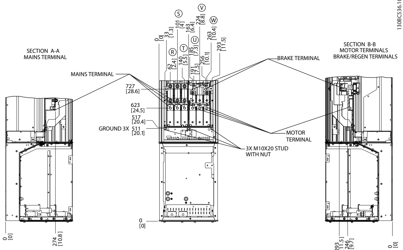
Εικόνα 2.14 Θέσεις ακροδεκτών, D5h με επιλογή πέδησης
