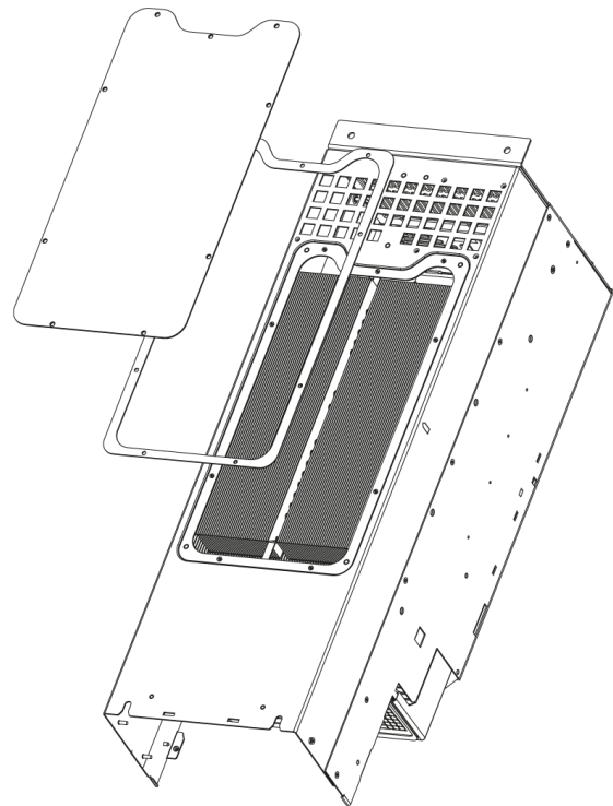
그림 7.1 방열판 액세스 패널
