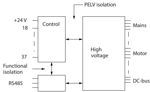
그림 8.1 PELV 절연
