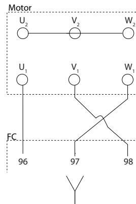
그림 5.5 모터 회전 변경을 위한 배선
