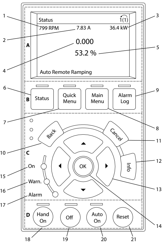
그림 5.1 현장 제어 패널(LCP)
