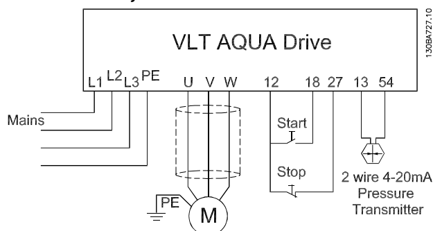
Slika 8.4 Ožičenje za primjene s potopnom pumpom
