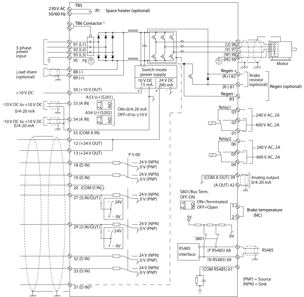
図 5.2 基本配線図
