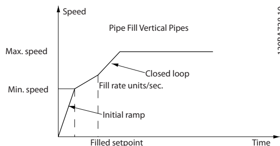
図 8.5 配管充填モードの性能曲線
