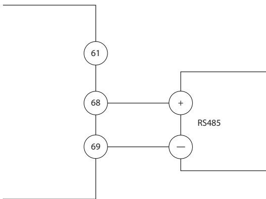
Illustration 5.21 Schéma de câblage de la communication série
