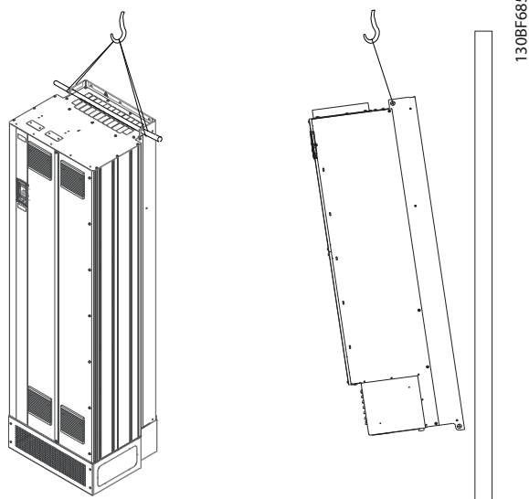
Illustration 4.2 Méthode de levage recommandée
