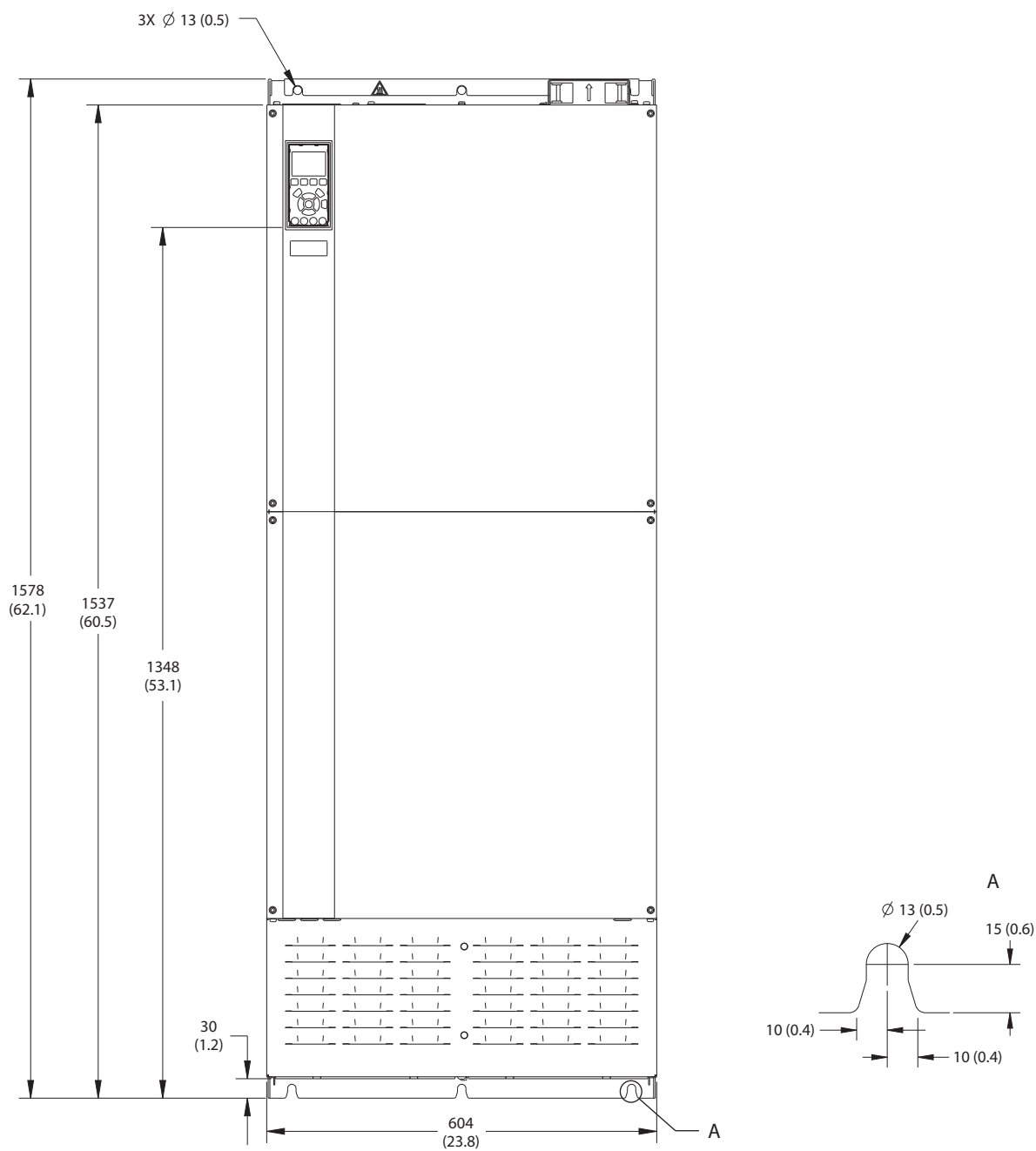
図 9.14 E4h の正面図
