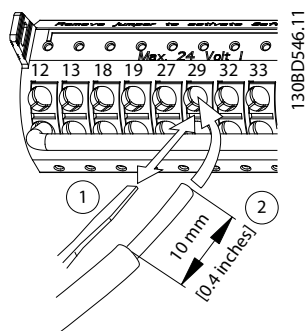
図 5.20 コントロール配線の接続
