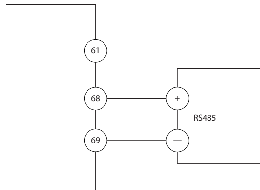
図 5.22 シリアル通信 配線図
