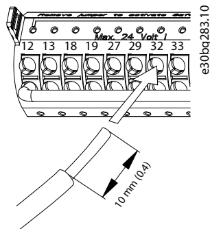
圖 5.20 連接實心的控制電線
