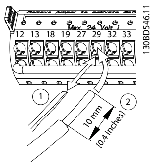
圖 5.21 連接軟型控制電線
