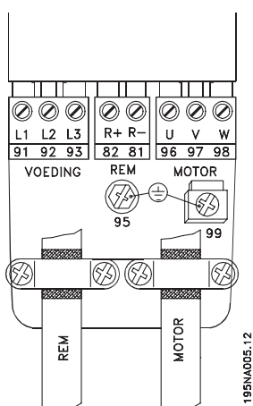
Afbeelding 4.1 Klemmen
