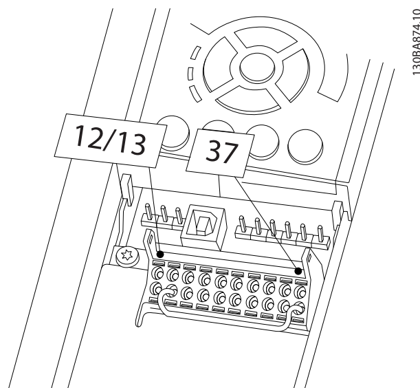
Disegno 2.19 Ponticello tra i morsetti 12/13 (24 V) e 37
