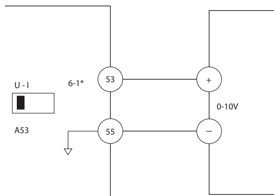
Disegno 5.8 Esempio di cablaggio per il dispositivo esterno che fornisce un segnale di controllo da 0-10 V (convertitore di frequenza a sinistra, dispositivo esterno a destra)
