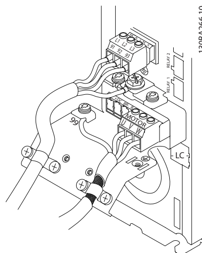
Disegno 2.7 Messa a terra con cavo schermato
