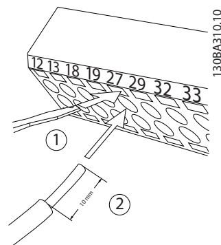
Disegno 2.13 Collegamento dei cavi di controllo
