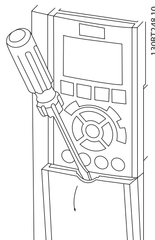
Disegno 2.9 Accesso ai cavi di controllo per le custodie A2, A3, B3, B4, C3 e C4
