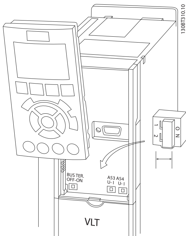
Disegno 2.18 Posizione dei morsetti 53 e 54 Interruttori e interruttore di terminazione bus
