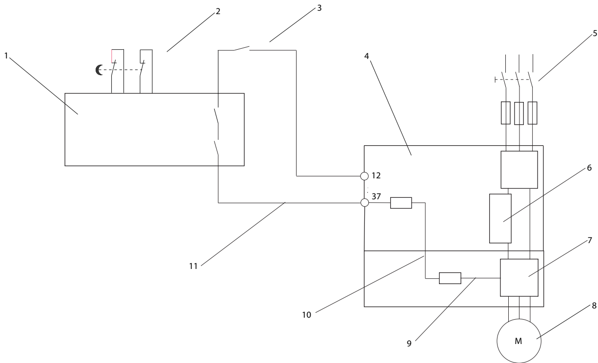
图 2.20 在安全类别 3 (EN 954-1) / PL “d” (ISO 13849-1) 基础上实现停止类别 0 (EN 60204-1)
