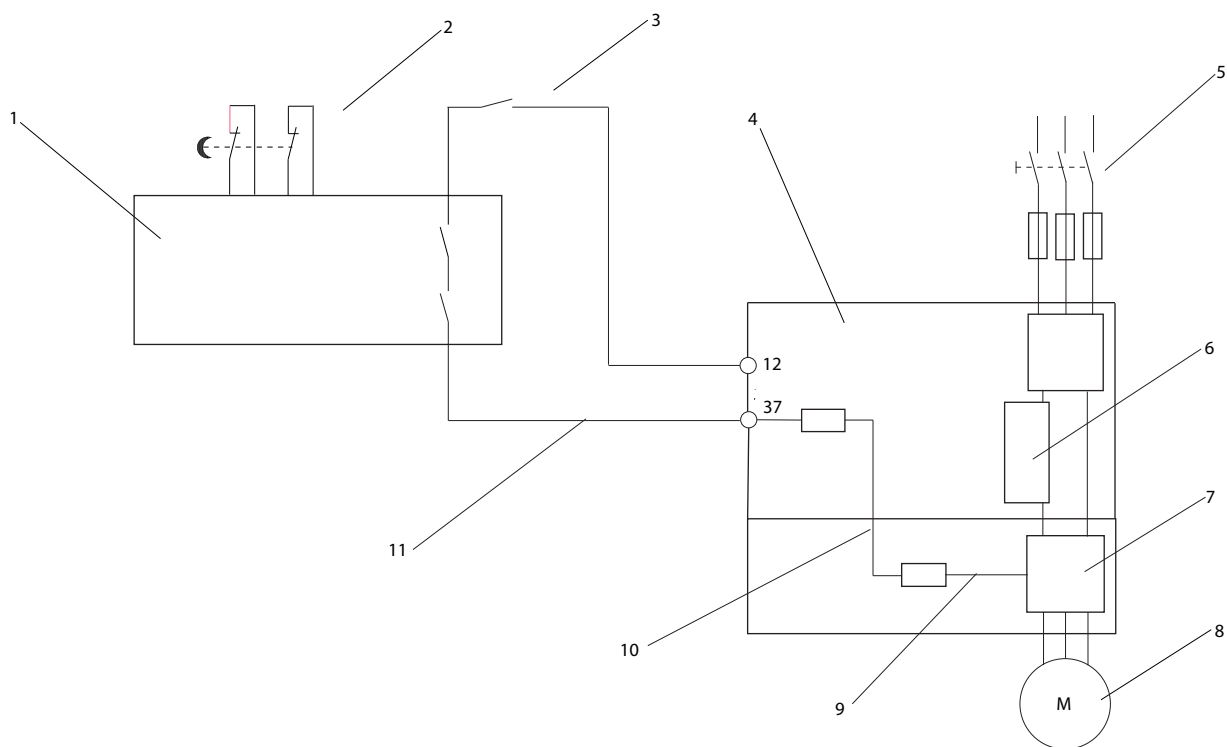
圖 2.20 符合安全類別 3 (EN 954-1) / PL “d” (ISO 13849-1) 和停止類別 0 (EN 60204-1) 的安裝
