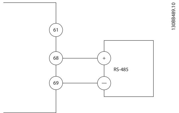
圖 2.22 串列通訊配線圖
