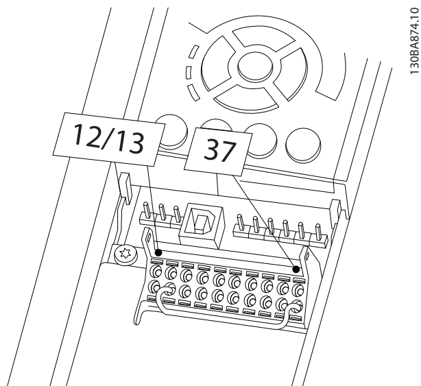
圖 2.19 端子 12/13 (24 V) 和 37 之間的跳線
