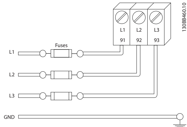
Slika 2.6 Osigurači frekventnog pretvarača
