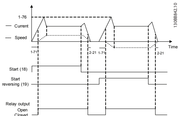
Εικόνα 6.1 Έλεγχος μηχανικής πέδης
