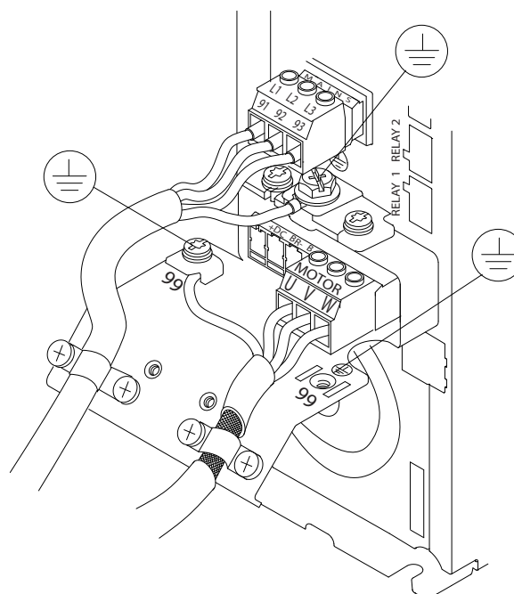
圖 4.5 馬達、主電源與接地線路的範例
