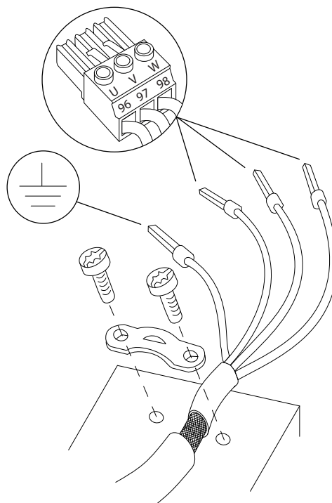
圖 4.4 馬達連接
