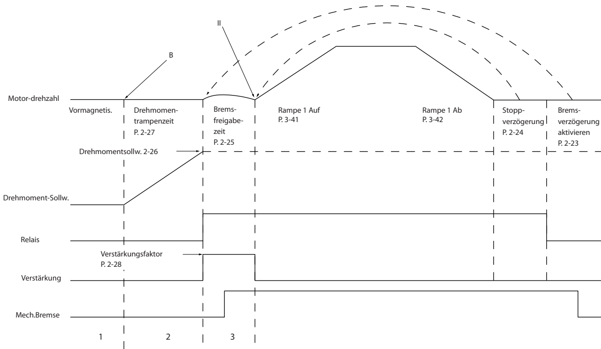
Abbildung 3.20 Ablauf beim Lüften der Bremse bei mechanischer Bremssteuerung in Hubanwendungen
