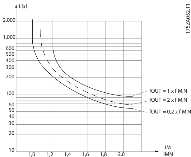
Abbildung 3.16 ETR-Profil
