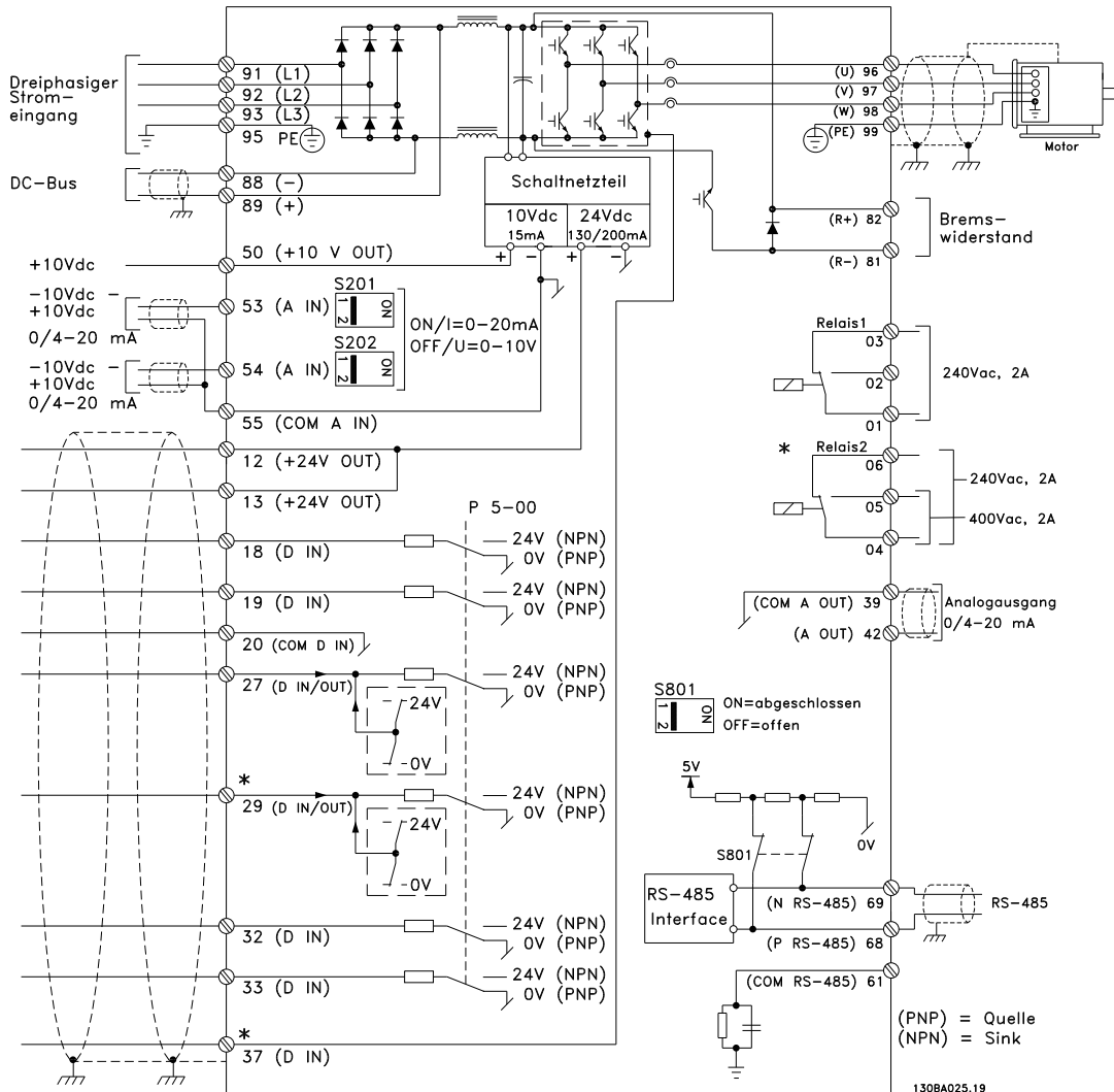
Abbildung 1.2 Schaltbild mit allen elektrischen Klemmen ohne Optionen.
