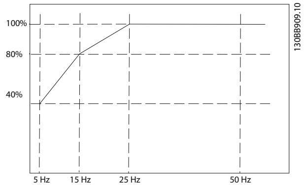
Abbildung 3.18 Beispiel einer thermischen Begrenzungskurve bei ATEX ETR.
