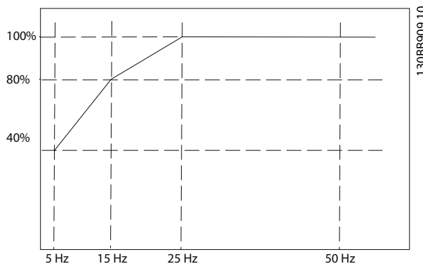
Ilustração 3.18 Exemplo de curva de limitação térmica TEX ETR. eixo x: f_m [Hz] eixo y: I_m/I_{m,n} \times 100 [%]
