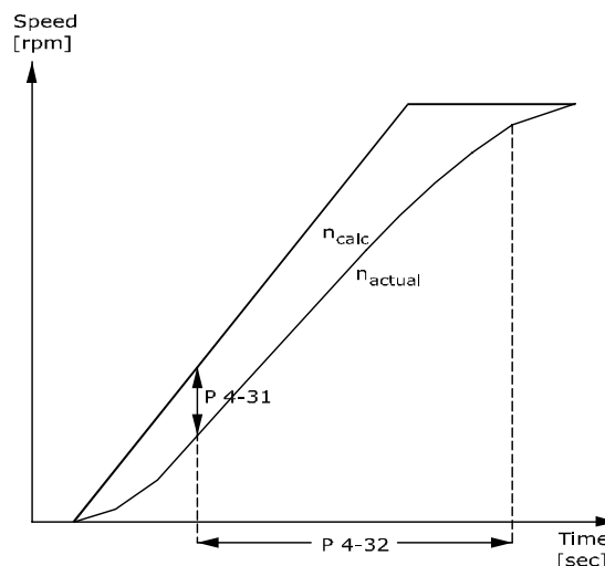
130BA221.10 Рисунок 3.31
