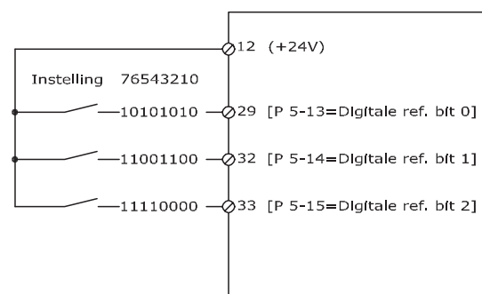
Afbeelding 3.21 Ingestelde ref.
