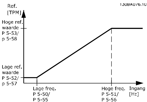
Afbeelding 3.37 Pulsingang
