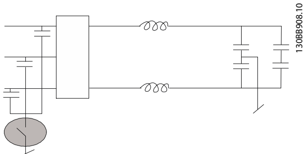
Afbeelding 3.60 RFI-filter
