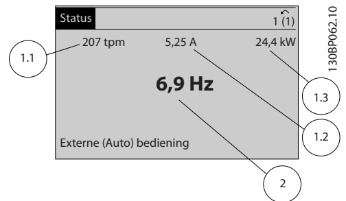
Afbeelding 2.11 Statusscherm II
