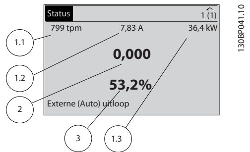
Afbeelding 2.10 Statusscherm I
