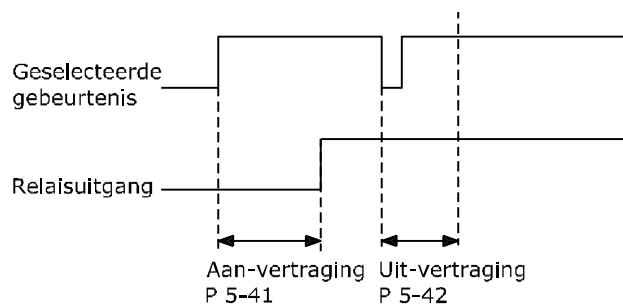
Afbeelding 3.36 Uit-vertr., relais
