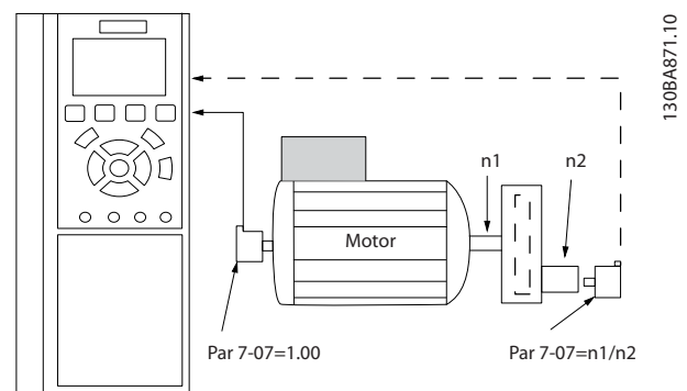
Afbeelding 3.46 Snelheids-PID, terugk overbr.verh.
