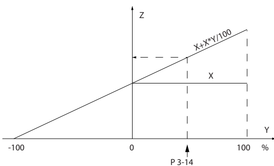
Afbeelding 3.23 Actuele referentie
