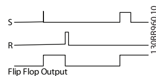
Afbeelding 3.52 Flip-flopuitgangen
