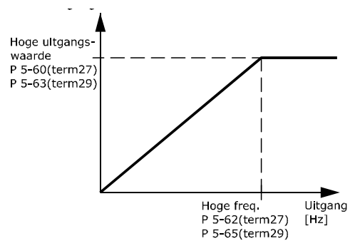
Afbeelding 3.38 Configuratie van pulsuitgangen
