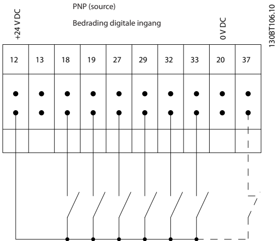
Afbeelding 1.3 PNP (source)
