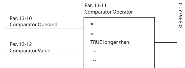
Afbeelding 3.50 Comparatoren
