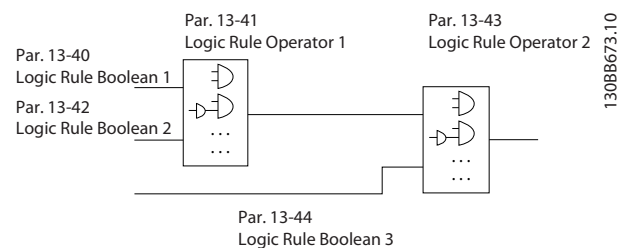
Afbeelding 3.53 Log. regels
