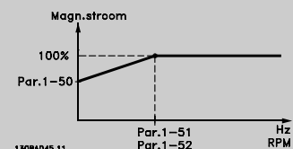
Afbeelding 3.7 Motormagnetisering
