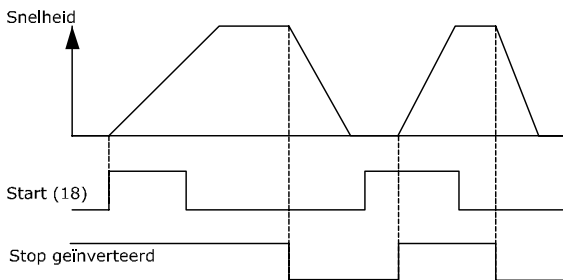
Afbeelding 1.7 Pulsstart/stop
