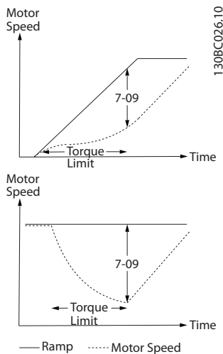
Afbeelding 3.47 Snelheidsfout tussen de ramp en het actuele toerental
