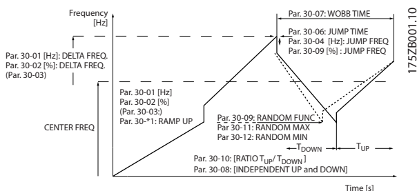
Afbeelding 3.64 Wobbelfunctie
