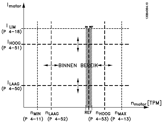
Afbeelding 3.32 Aanp. waarsch.
