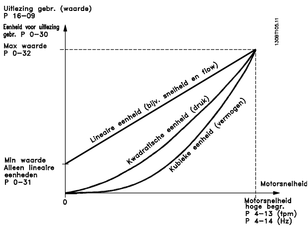
Afbeelding 3.4 Uitlezing gebruiker
