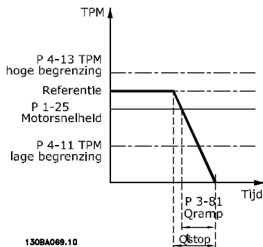
Afbeelding 3.28 Snelle stop ramp-tijd
