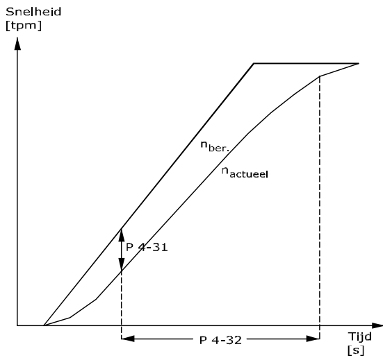
Afbeelding 3.31 Motorterugkoppelingssnelh. fout
