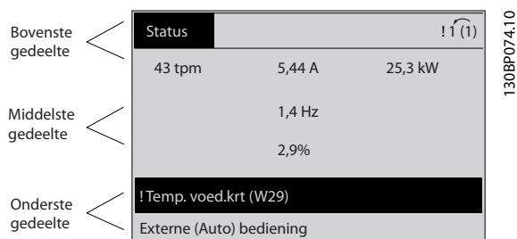
Afbeelding 2.2 Lcd-scherm
