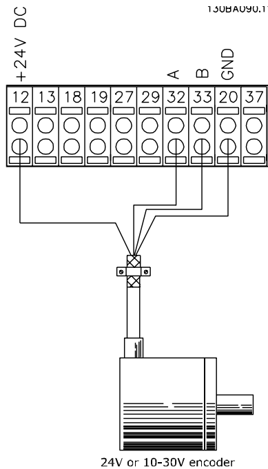
Afbeelding 3.39 Encoderaansluiting
