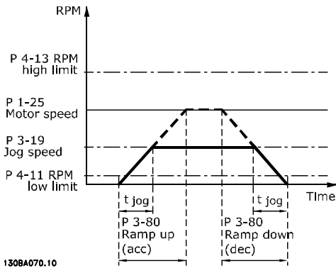
Afbeelding 3.27 Jog ramp-tijd
