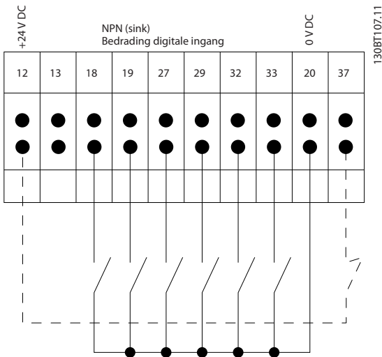
Afbeelding 1.4 NPN (sink)
