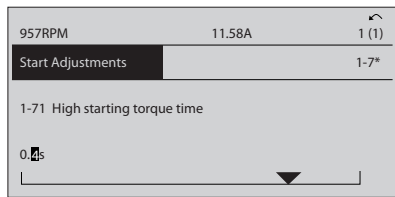
Afbeelding 2.20 Opslaan
