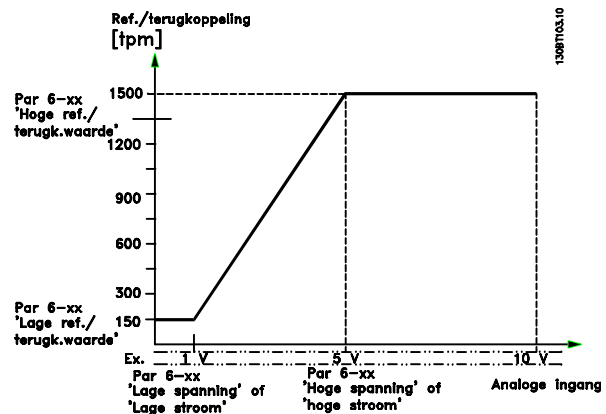
Afbeelding 3.41 Anal. ingang 1
