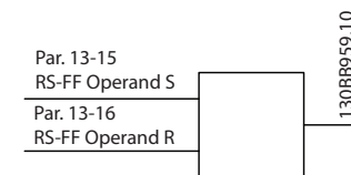
Afbeelding 3.51 Reset/Set-flipflops
