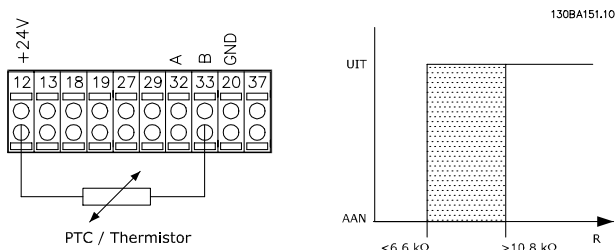
Afbeelding 3.17 Aansluiting thermistor
