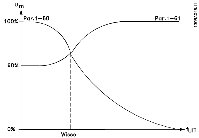
Afbeelding 3.11 Omschakeling
