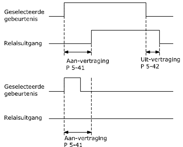
Afbeelding 3.35 Aan-vertr., relais
