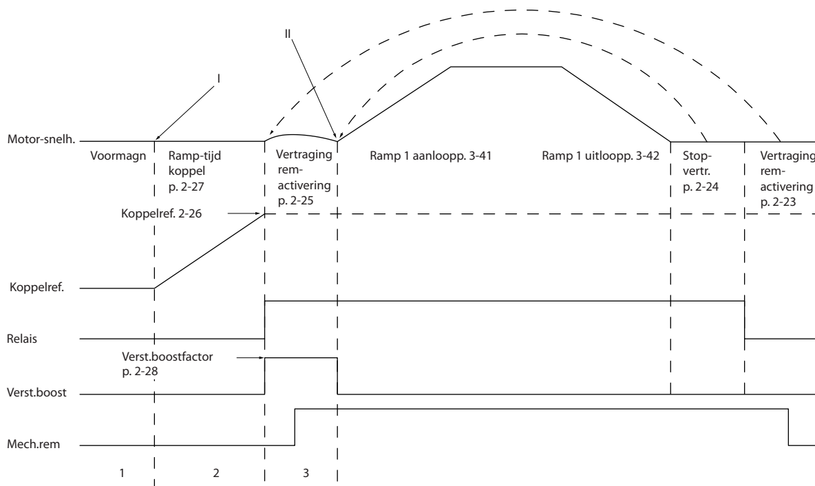
Afbeelding 3.20 Remvrijgaveprocedure voor mechanische rembesturing bij hijstoepassingen Dit type rembesturing is alleen beschikbaar bij een fluxregeling met motortrugkoppeling, beschikbaar voor asynchrone motoren en PM-motoren met niet-uitspringende magneten.
