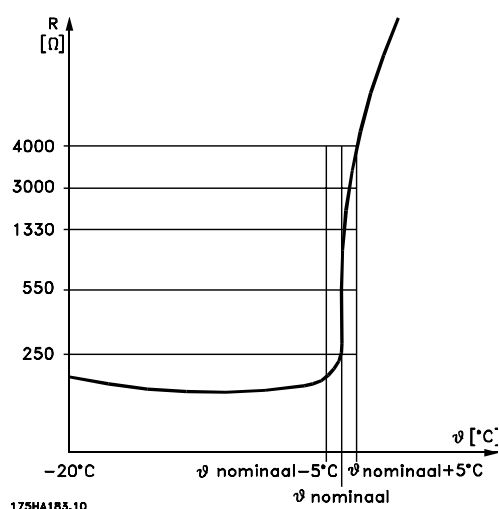
Afbeelding 3.12 PTC-profiel
