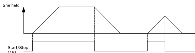
Afbeelding 1.6 Start/Stop
