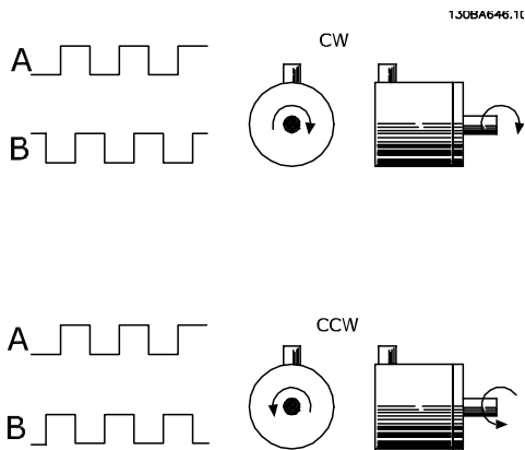
Afbeelding 3.40 Draairichting encoder
