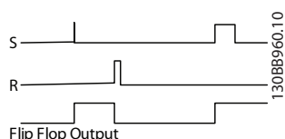
图 3.52 正反器输出
