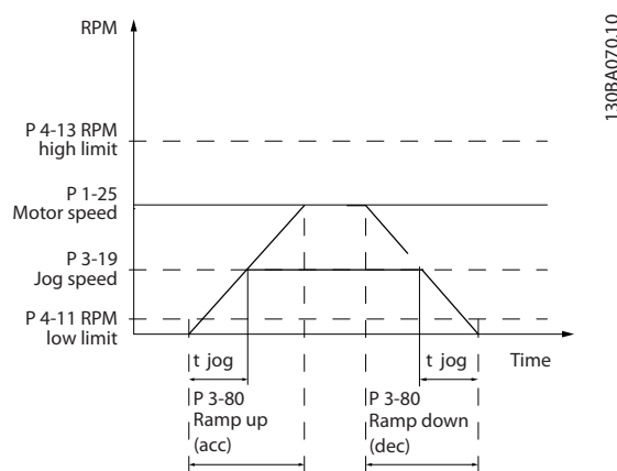
图 3.27 点动加斜坡时间
