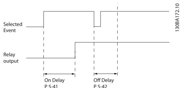
图 3.36 继电器关闭延迟
