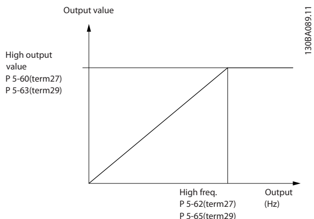
图 3.38 脉冲输出的配置
