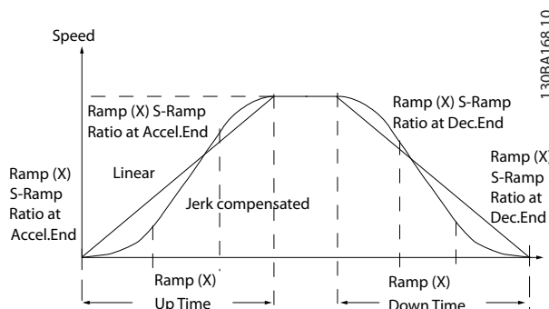
图 3.26 线性加减速时间
