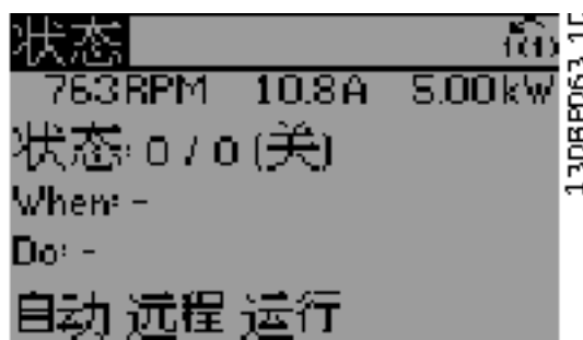
图 2.12 状态屏幕 III
