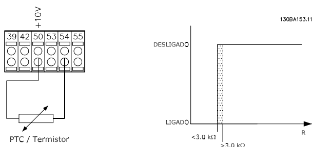
图 3.14 PTC 热敏电阻连接 - 模拟输入
