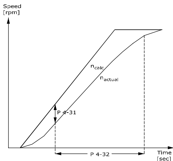
图 3.31 电机反馈速度错误
