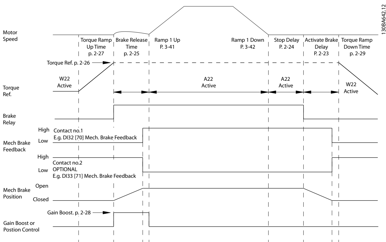
图 3.20 起重机械制动控制的抱闸释放过程 此制动控制仅在带电动机反馈的磁通矢量中可用，对于异步和非突出 PM 电动机可用。
