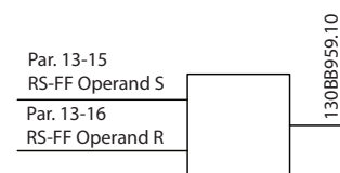
图 3.51 复位/设置触发器
