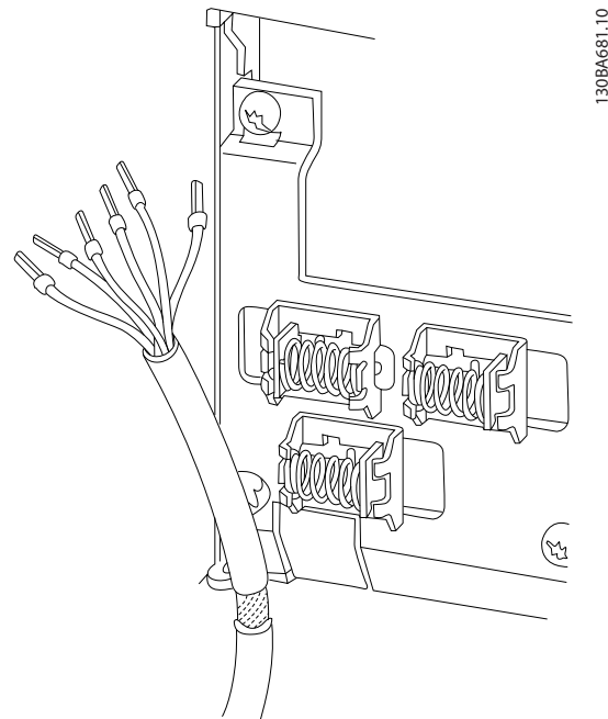
图 1.5 屏蔽/铠装控制电缆的接地
