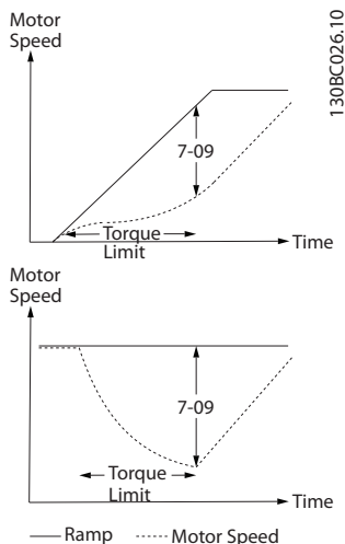
图 3.47 加减速和实际速度之间的速度误差
