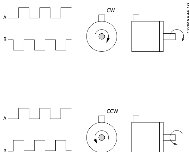
图 3.40 编码器旋转方向
