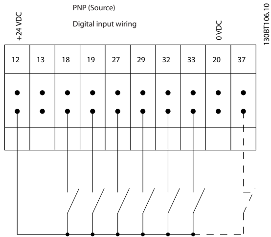
图 1.3 PNP (源型)
