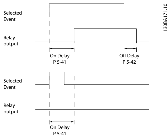
图 3.35 继电器打开延时
