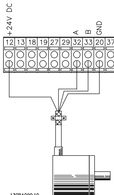
图 3.39 编码器连接
