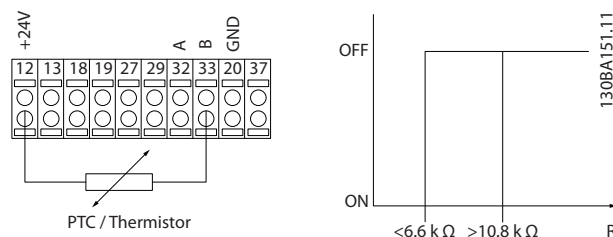
图 3.17 热敏电阻连接
