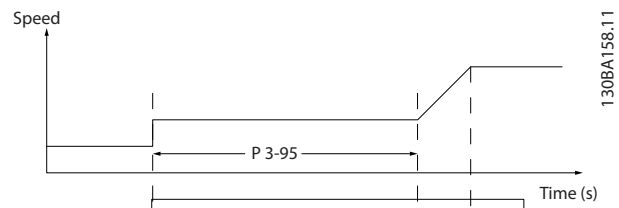
图 3.29 增加实际参考值
