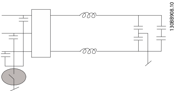
图 3.60 射频干扰滤波器
