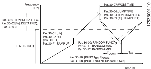
图 3.64 摆频功能
