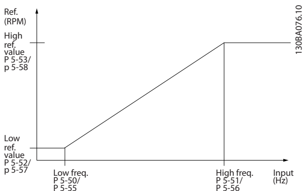
图 3.37 脉冲输入
