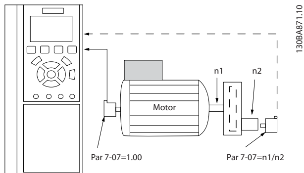
图 3.46 速度 PID 反馈传动比
