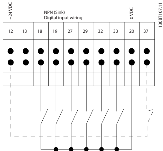
图 1.4 NPN (漏型)
