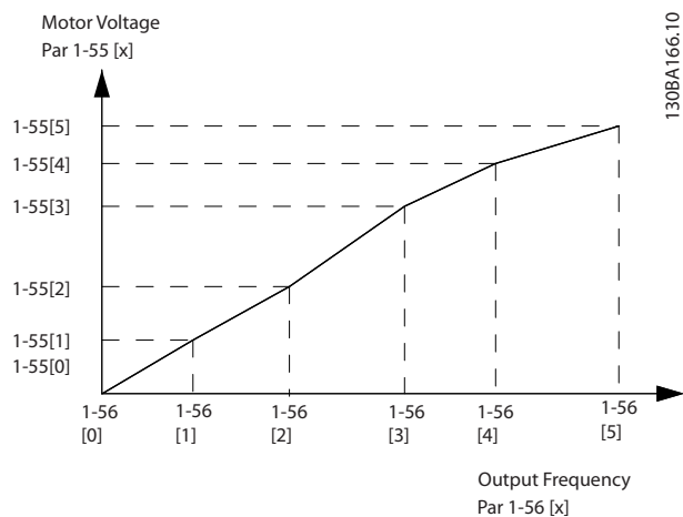
图 3.10 U/f 特性
