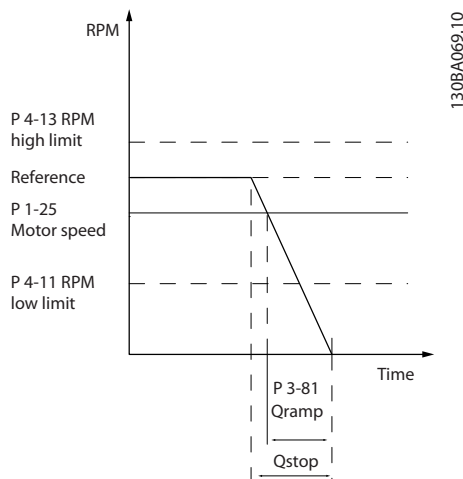
图 3.28 快速停止减速时间
