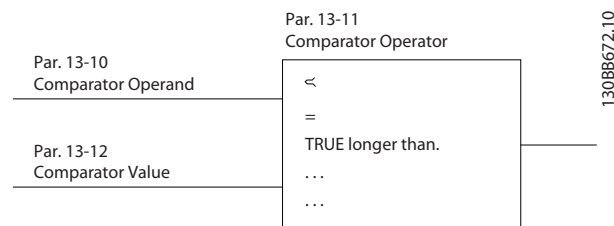
图 3.52 比较器
