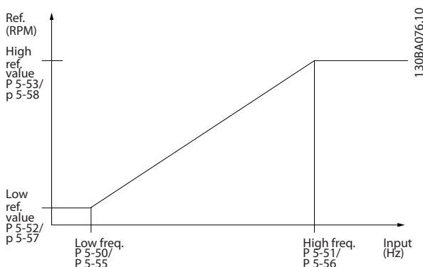
图 3.38 脉冲输入
