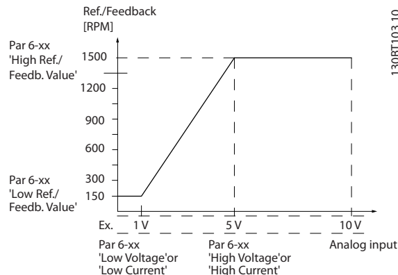
图 3.42 模拟输入 1
