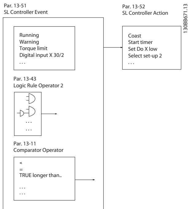
图 3.50 智能逻辑控制 (SLC)
