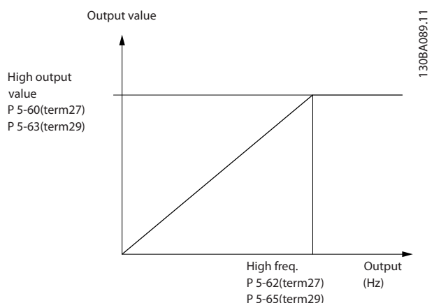
图 3.39 脉冲输出的配置
