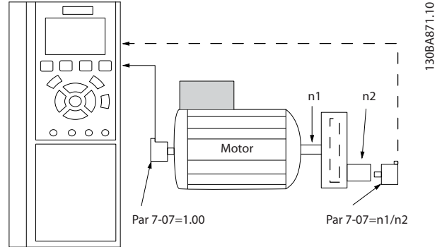
图 3.48 速度 PID 反馈传动比
