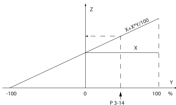
图 3.23 实际参考值
