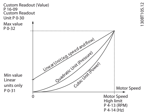
图 3.4 自定义读数
