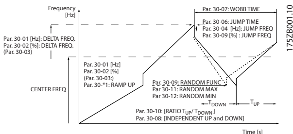
图 3.66 摆频功能
