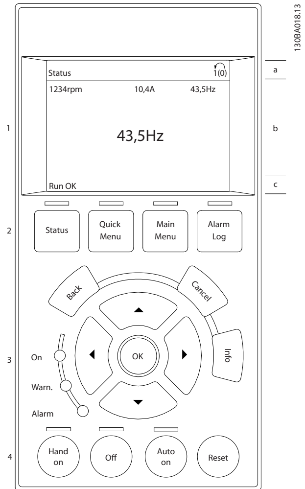
图 2.1 LCP
