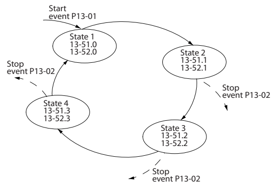
图 3.51 事件和操作
