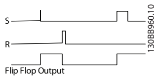
图 3.54 正反器输出
