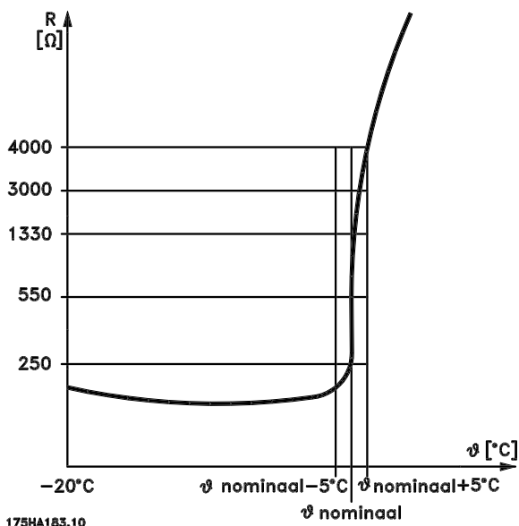
图 3.12 PTC 协议
