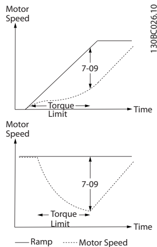
图 3.49 加减速和实际速度之间的速度误差
