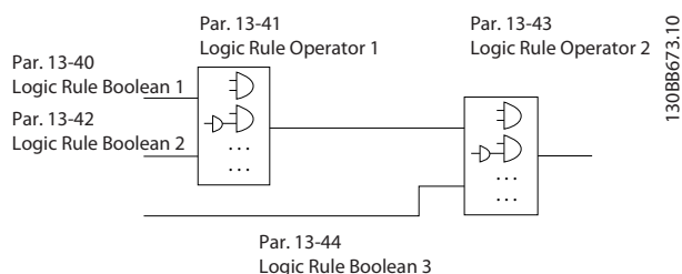
图 3.55 逻辑规则
