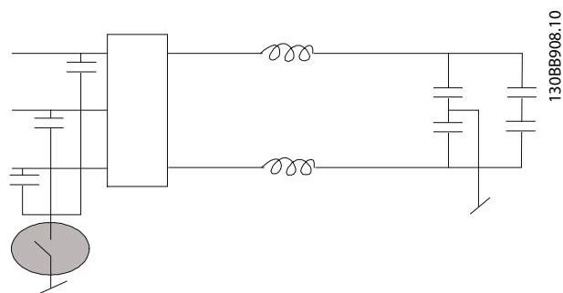
图 3.62 射频干扰滤波器
