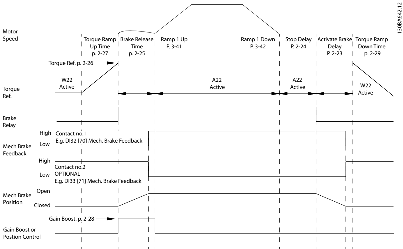
图 3.20 起重机械制动控制的抱闸释放过程 此制动控制仅在带反馈的磁通矢量控制原理或无传感器模式中可用，对于异步和非突出 PM 电动机可用。
