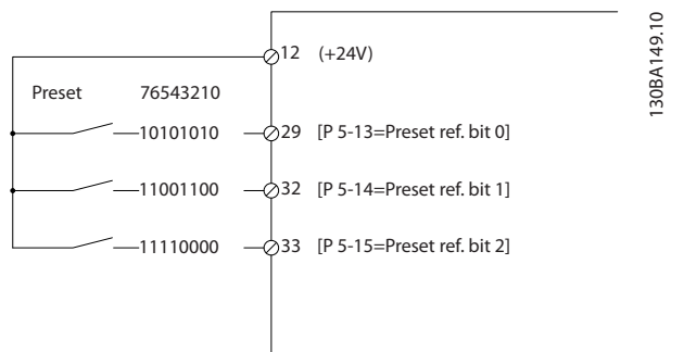
图 3.21 预置参考值
