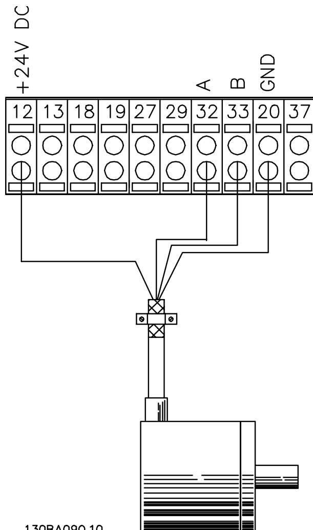
130BA090.10 图 3.40 编码器连接
