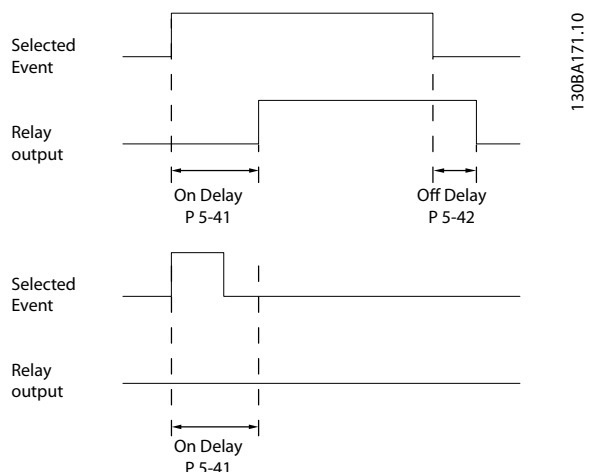
图 3.36 继电器打开延时
