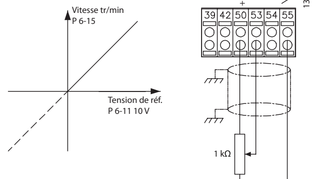
Illustration 1.9 Référence du potentiomètre
