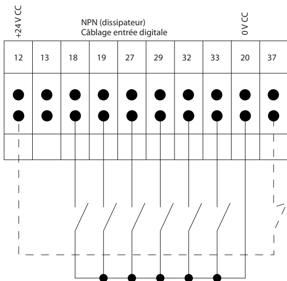
Illustration 1.4 NPN (dissipateur)
