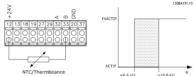
Illustration 3.17 Connexion de la thermistance
