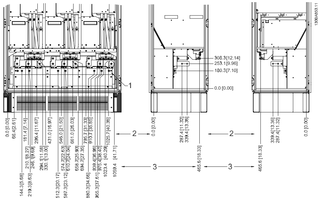
Kuva 3.23: Liitinten paikat - vaihtosuuntaajakaappi - F2 ja F4 (näkömää edestä, vasemmalta ja oikealta). Läpivientilevy on 42 mm .0-tason alapuolella.
