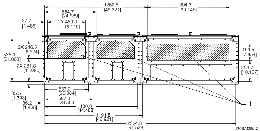
F1-F4: Kaapelin viennin taajuusmuuttajan pohjasta katsottuna - 1) Sijoitusputket merkittyihin kohtiin
