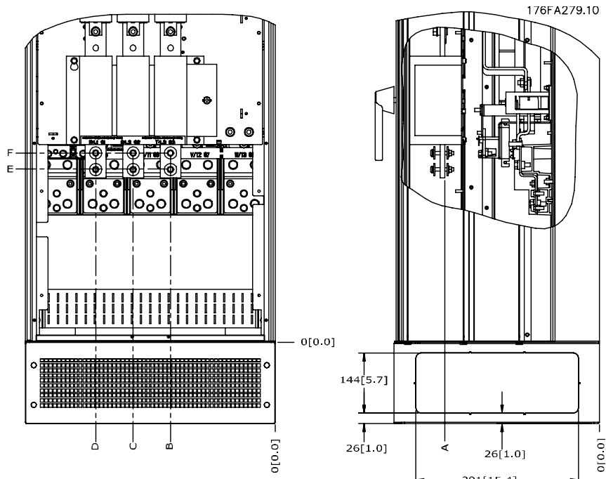
Kuva 3.17: IP21 (NEMA-tyyppi 1) ja IP54 (NEMA-tyyppi 12) -kotelo virtakytkennän katkaisimen paikka
