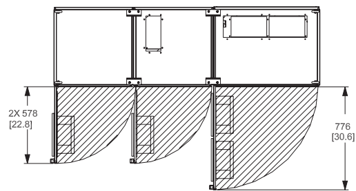
Kuva 3.10: Tila IP21/IP54-kotelointityyppien, kehyskoon F3
