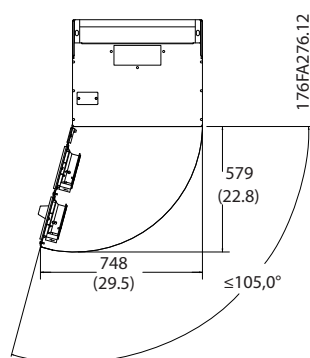
Slika 3.7 Prostor ispred kućišta IP21/IP54, veličina okvira E1.
