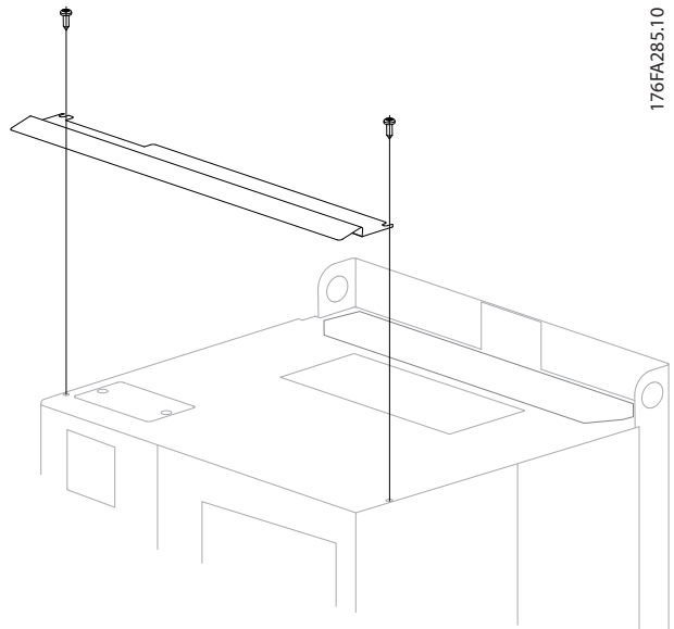
Slika 3.40 Instalacija štita kapanja.
