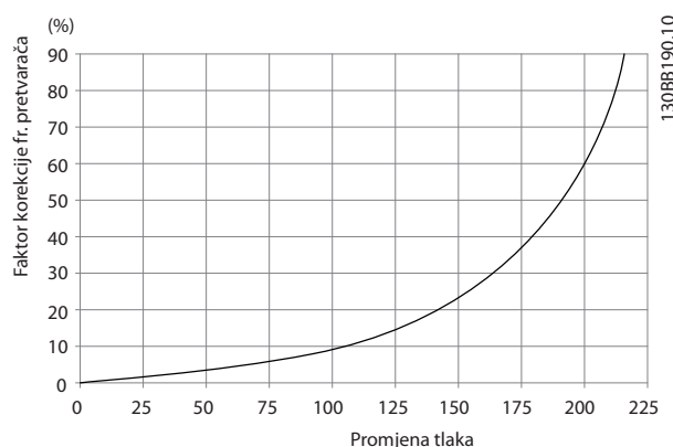
Slika 3.31 F1, F2, F3, F4 okvir Korekcija vs. Promjena tlaka Protok zraka frekvencijskog pretvarača: 580 cfm (985 m 3 /h)
