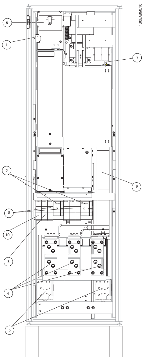
Slika 3.56 Ormarić ispravljača, veličina okvira F1, F2, F3 i F4
