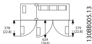
Slika 3.10 Prostor ispred kućišta IP21/IP54, veličina okvira F2
