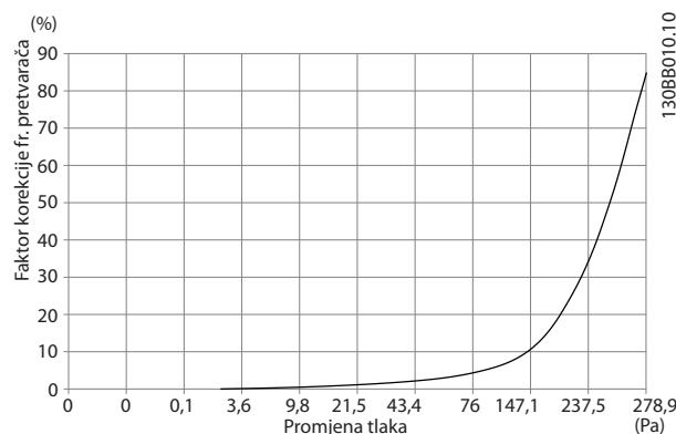
Slika 3.29 E okvir Korekcija vs. Promjena tlaka (Mali ventilator), P250T5 i P355T7-P400T7 Protok zraka frekvencijskog pretvarača: 650 cfm (1.105 m 3 /h)
