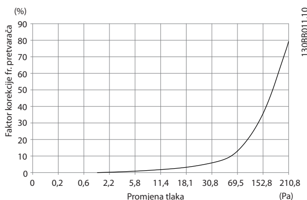
Slika 3.30 E okvir Korekcija vs. Promjena tlaka (Veliki ventilator), P315T5-P400T5 and P500T7-P560T7 Protok zraka frekvencijskog pretvarača: 850 cfm (1.445 m 3 /h)
