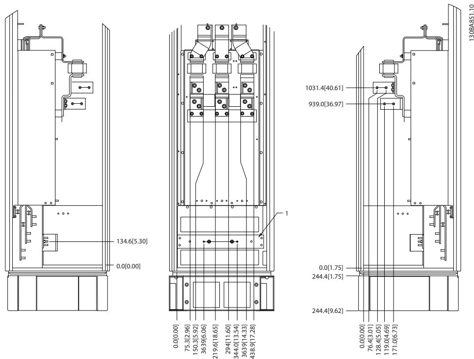
Slika 3.26 Lokacije stezaljki - opsijska kutija (pogled sprijeda, slijeva i zdesna). Ploča brtve je 42 mm ispod razine 0.
