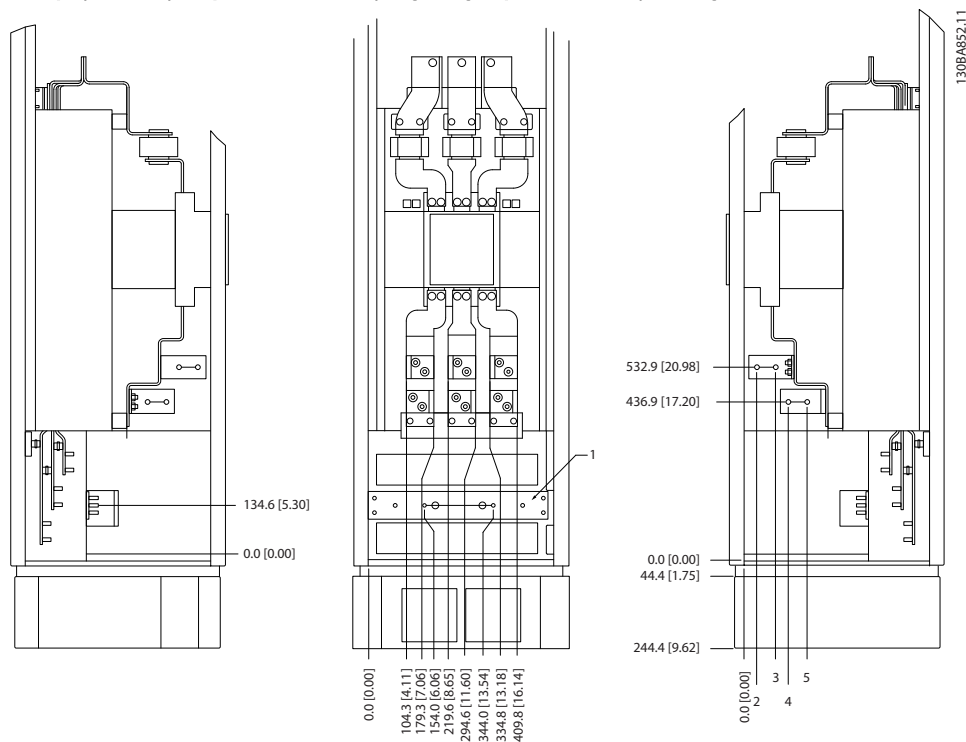
Slika 3.27 Lokacije stezaljki - Opcijska kutija s prekidačem strujnog kruga/ prekidačem lijevanog kućišta (pogled sprijeda, slijeva i zdesna). Ploča brtve je 42 mm ispod razine 0.
