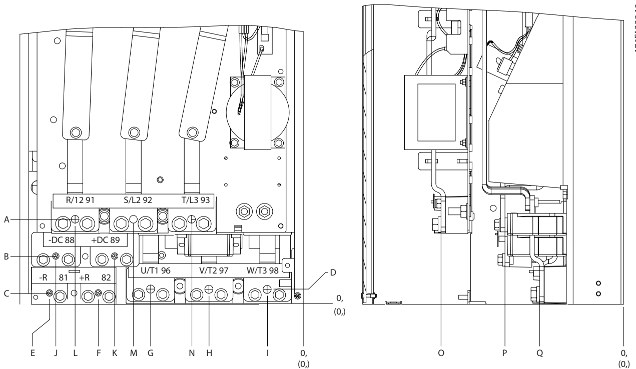
Slika 3.62 Položaji strujnih spojeva, veličina okvira D3 i D4
