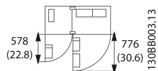
Slika 3.8 Prostor ispred kućišta IP21/IP54, veličina okvira F1
