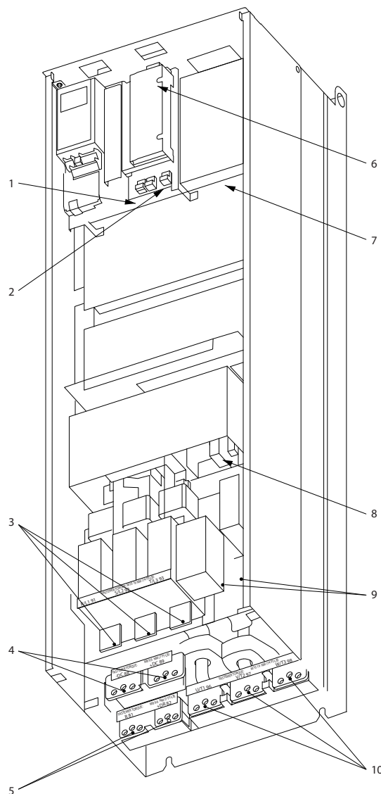
Slika 3.50 Compact IP 00 (Kućičte) s odspajanjem, osiguračem i RFI filtrom, veličina okvira D4
