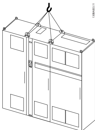
Slika 3.4 Preporučeni način podizanja, Veličina okvira F3 (460V, 600 do 900 HP, 575/690V, 900 do 1.150 HP).
