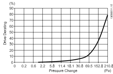
图 3.29: E 机架 的降容与 压力变化 (大风扇)、P315T5-P400T5 和 P500T7-P560T7 变频器气流: 850 cfm (1445 m 3 /h)
