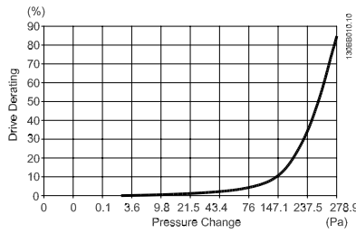
图 3.28: E 机架 的降容与 压力变化 (小风扇)、P250T5 和 P355T7-P400T7 变频器气流: 650 cfm (1105 m 3 /h)
