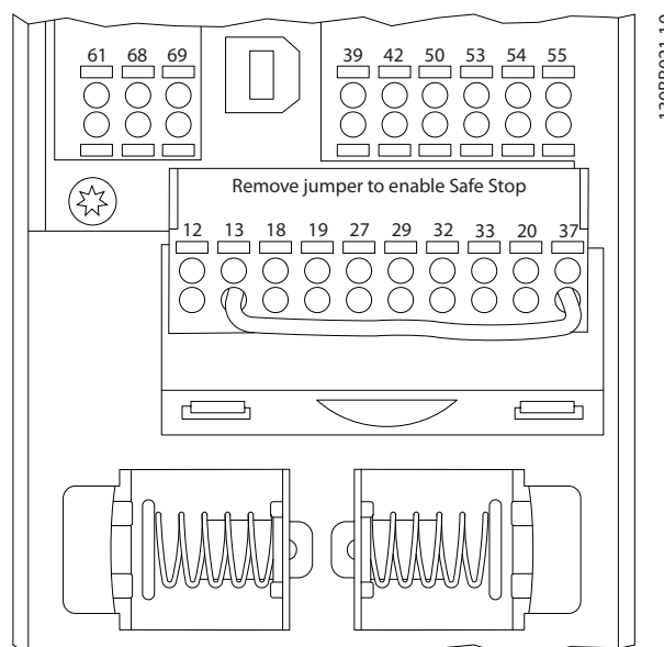
Afbeelding 7.1 Stuurkaartklemmen
