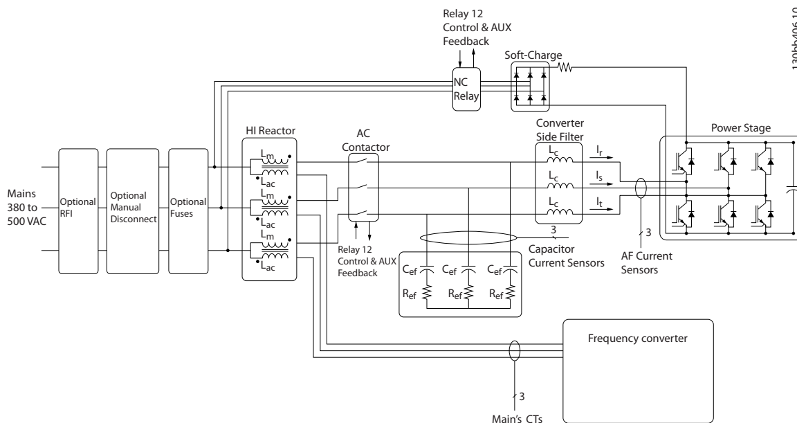
Afbeelding 3.1 Basislay-out voor de Low Harmonic Drive
