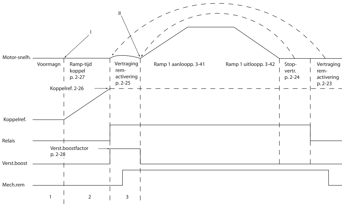
Afbeelding 6.4 Remvrijgaveprocedure voor mechanische rembesturing bij hijstoepassingen
