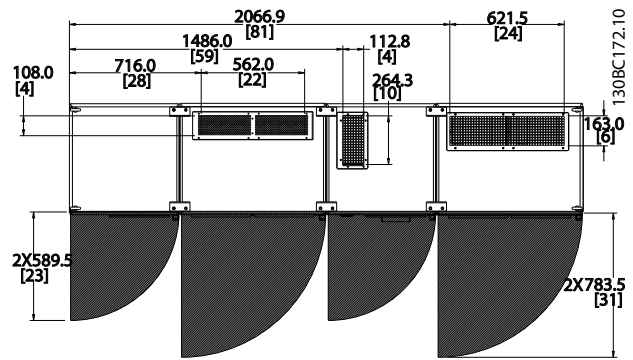
Afbeelding 4.12 Ruimte aan voorzijde van framegrootte F18 met IP 21/IP 54-behuizing.
