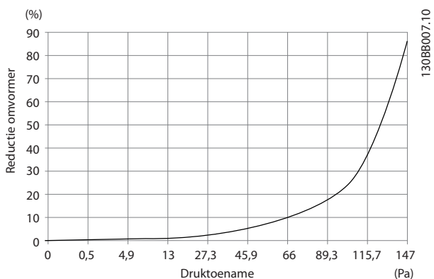
Afbeelding 4.21 Reductie framegrootte D t.o.v. drukverandering Luchtdoorstroming omvormer: 765 m 3 /u. (450 cfm)
