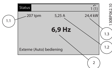
Afbeelding 5.3 Statusdisplay II – bedrijfsvariabelen
