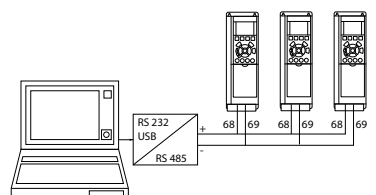
Afbeelding 5.8 Aansluitvoorbeeld.
