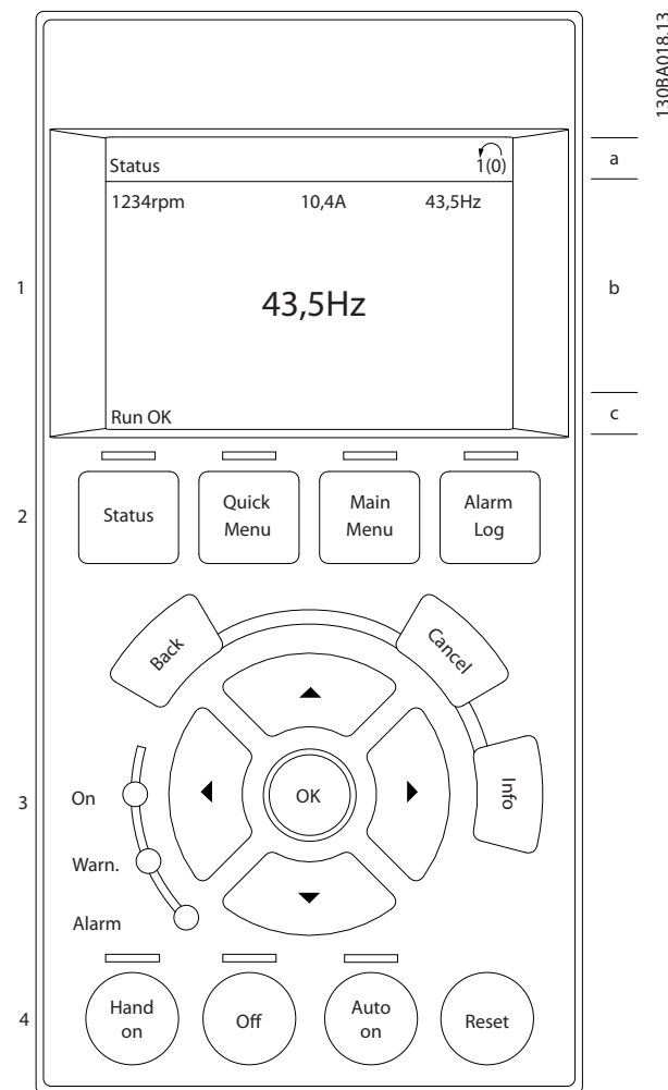
Afbeelding 5.1 LCP
