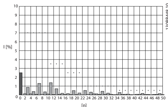
Afbeelding 3.2 Typisch frequentiespectrum van de harmonischen en THD-waarde bij de voedingsklemmen van de omvormer n = rangorde van de harmonischen ◆.....IEEE 519 ( I_{sc}/I_l > 20 ) limieten voor individuele harmonischen
