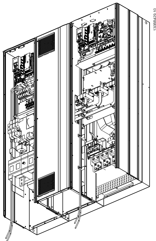
Afbeelding 4.39 Kabelroute voor stuurkaart, E9
