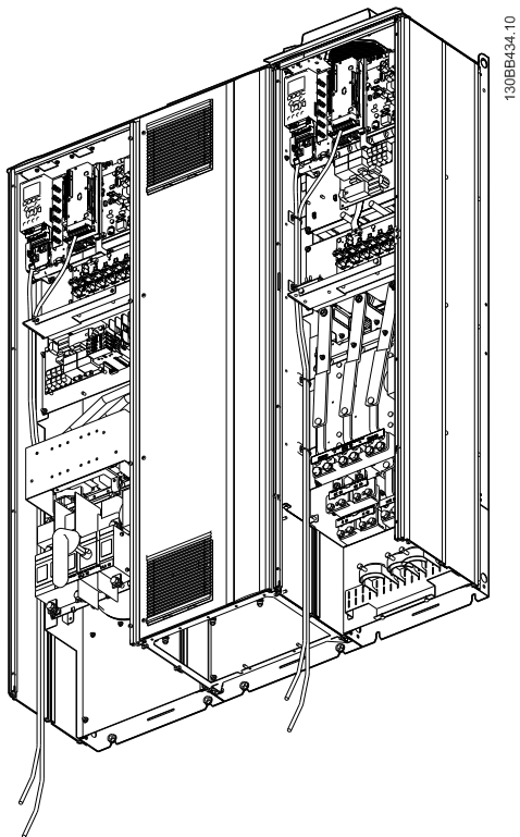
Afbeelding 4.38 Kabelroute voor stuurkaart, D13
