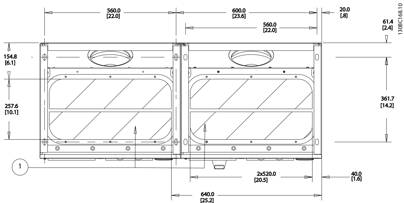
Afbeelding 4.27 Framegrootte E9
