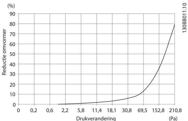
Afbeelding 4.23 Reductie framegrootte E t.o.v. drukverandering (grote ventilator), P355-P450 Luchtdoorstroming omvormer: 1445 m 3 /u. (850 cfm)
