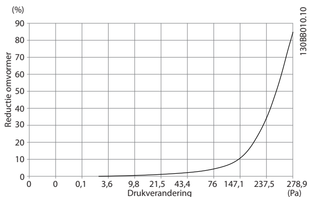
Afbeelding 4.22 Reductie framegrootte E t.o.v. drukverandering (kleine ventilator), P315 Luchtdoorstroming omvormer: 1105 m 3 /u. (650 cfm)
