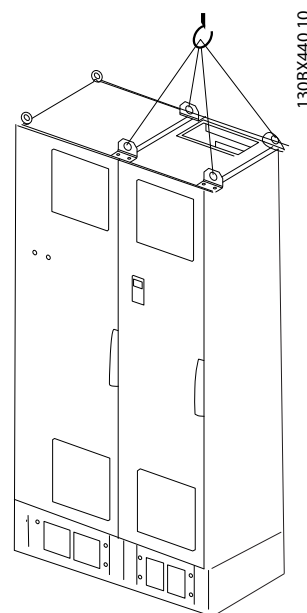
Afbeelding 4.4 Aanbevolen hijsmethode, framegrootte F18 – filterdeel
