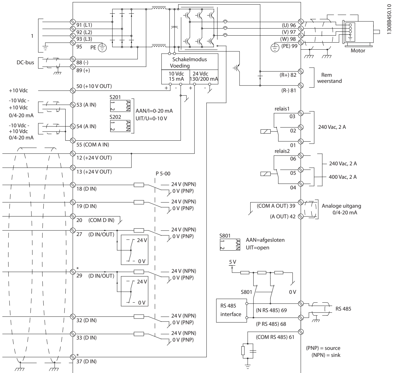
Afbeelding 4.40 Schema met alle elektrische klemmen zonder opties.
