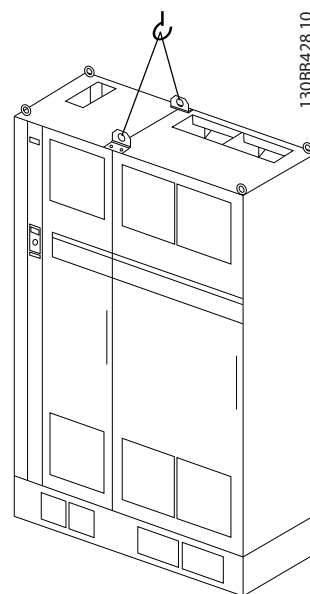
Afbeelding 4.5 Aanbevolen hijsmethode, framegrootte F18 – omvormerdeel
