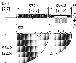
Afbeelding 4.10 Ruimte aan voorzijde van framegrootte D13 met IP 21/IP 54-behuizing.
