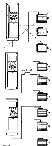
Afbeelding 4.41 Installaties met kabels die zijn aangesloten op een gezamenlijke verbinding
