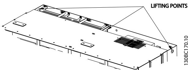
Afbeelding 4.3 Aanbevolen hijsmethode, framegrootte E9
