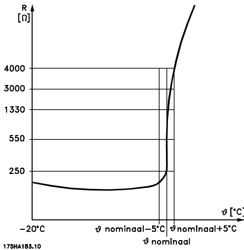
175HA183.10 Afbeelding 6.1 PTC-profiel
