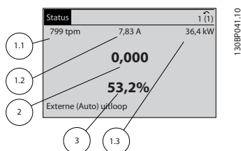
Afbeelding 5.2 Statusdisplay I – bedrijfsvariabelen
