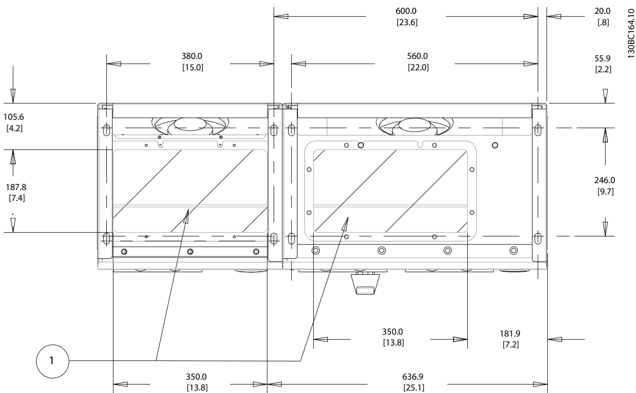
Afbeelding 4.26 Framegrootte D13
