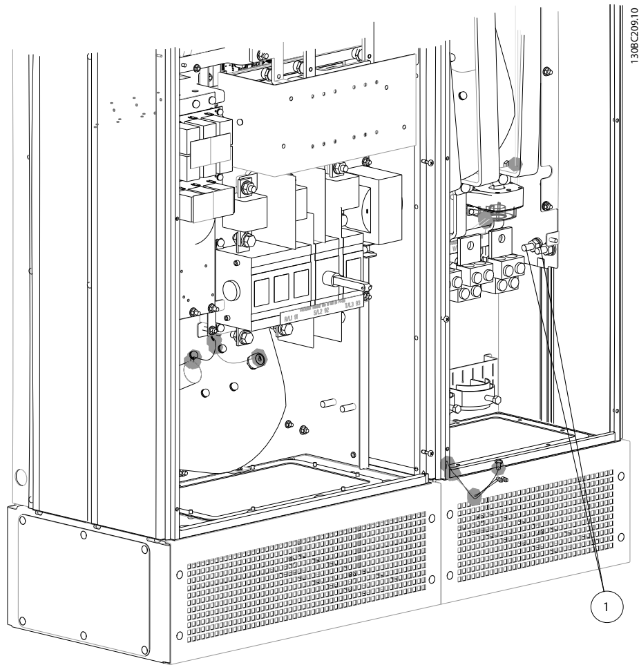
Afbeelding 4.31 Positie van aardklemmen
