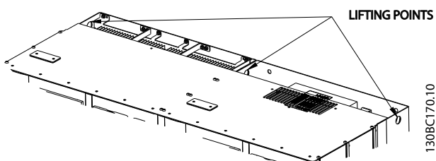
图 4.3 机架规格 E9 的建议起吊方法
