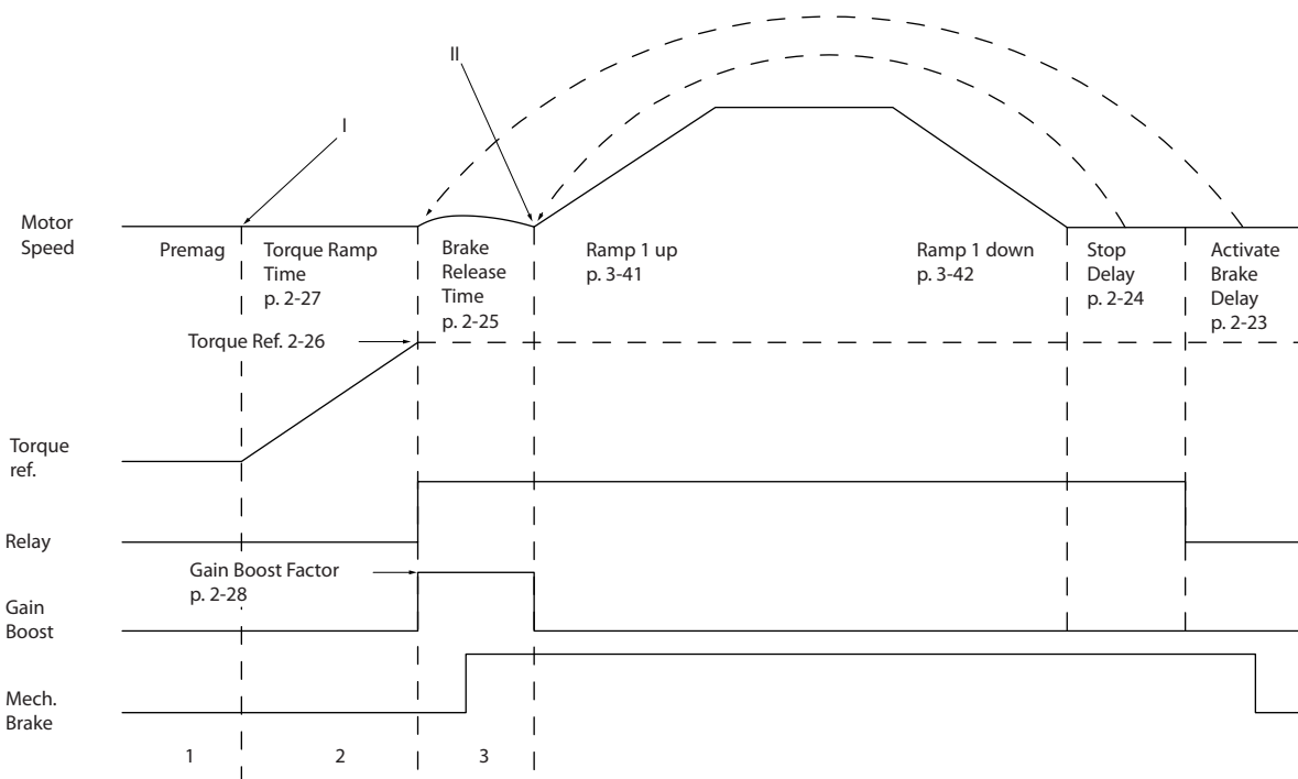
图 6.4 起重机械制动控制的抱闸释放过程
