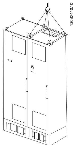
图 4.4 机架规格 F18 的建议起吊方法 - 滤波器单元。
