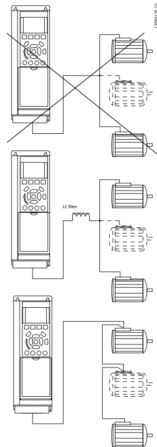
图 4.41 电缆连接到公共接点的系统
