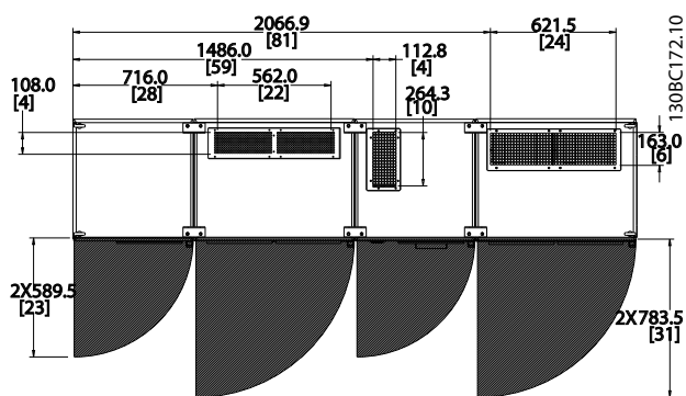
图 4.12 IP21/IP54 型机箱、F18 规格机架的前方空间。
