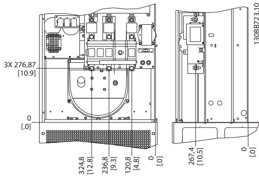
图 4.13 端子位置 - 主电源电缆
