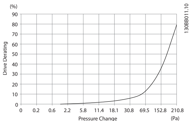
图 4.23 E 机架的降容与 压力变化 (大风扇) P355-P450 变频器气流: 850 cfm (1445 m 3 /h)
