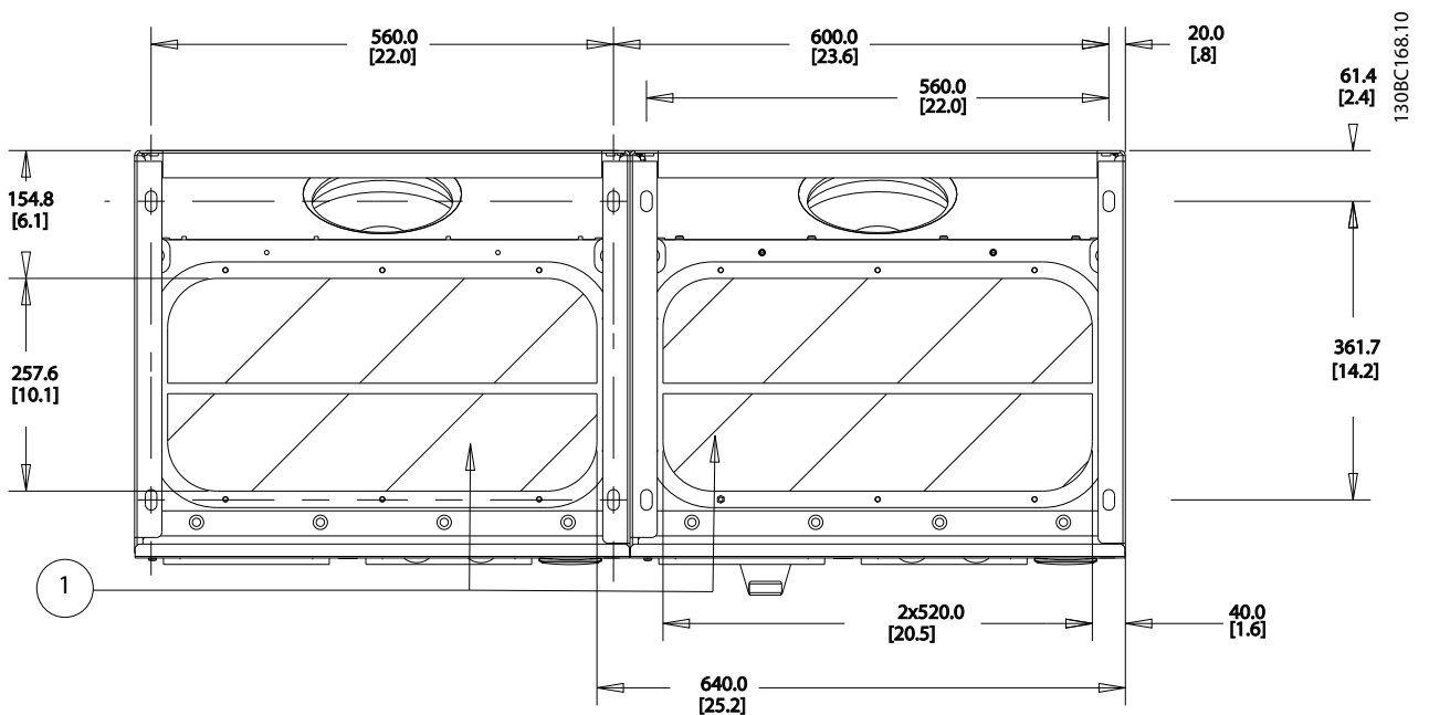
图 4.27 机架规格 E9
