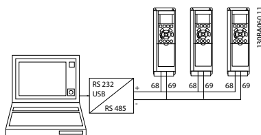
图 5.8 连接示例。
