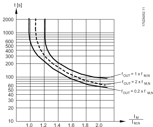
图 6.3 ETR 行规
