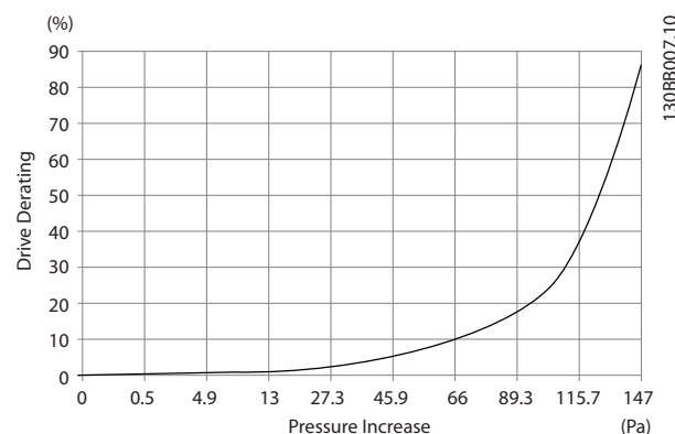
图 4.21 D 机架的降容与压力变化的关系
