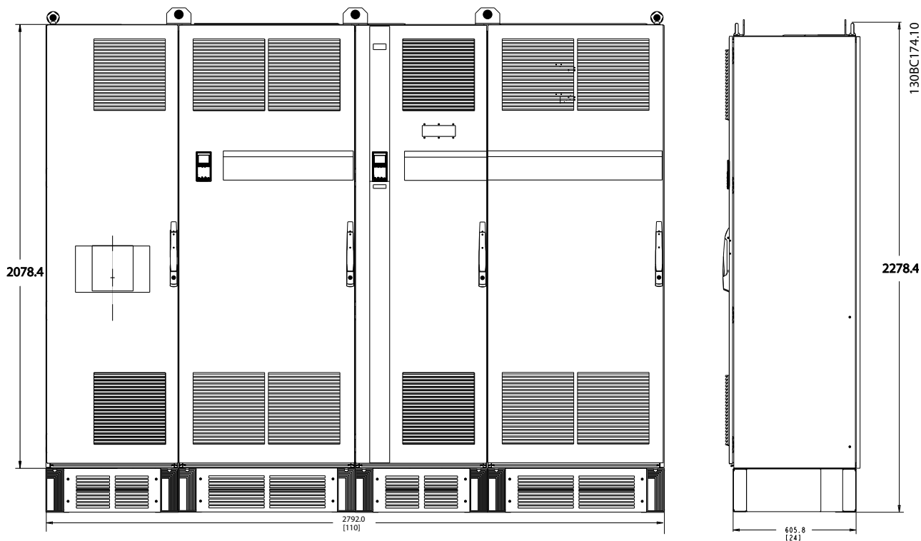
图 4.8 机架规格 F18 (正视图和侧视图)
