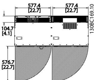
图 4.11 IP21/IP54 型机箱、E9 规格机架的前方空间。
