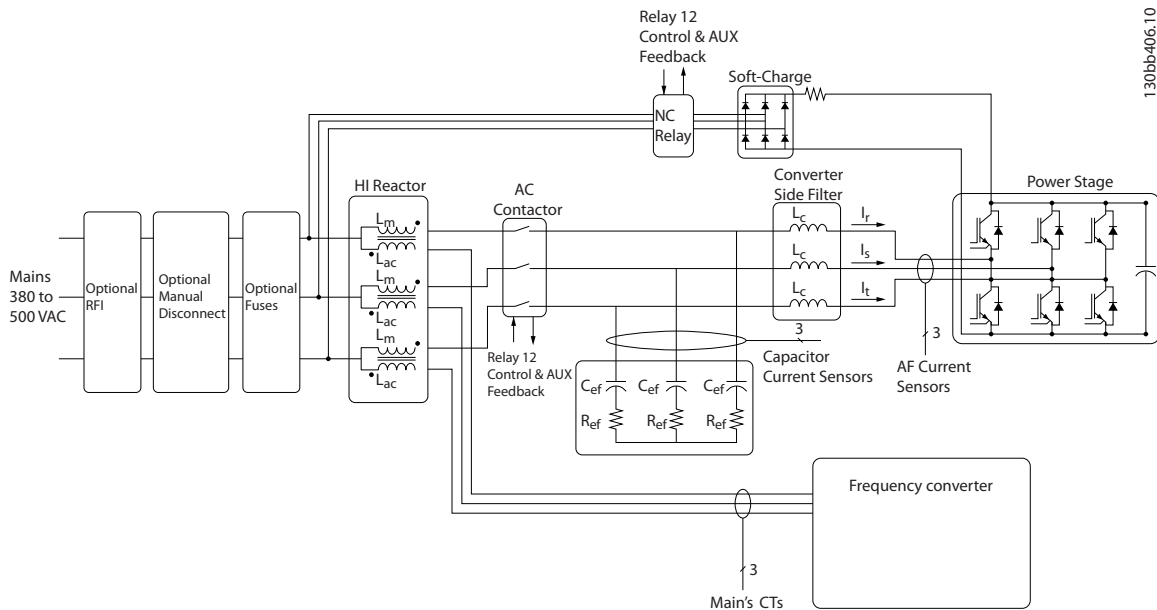
图 3.1 低谐波变频器的基本布局
