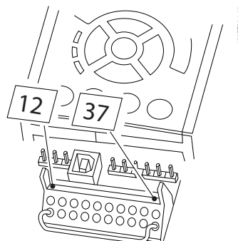
图 2.1 端子 37 和 24 V 直流之间的桥接跳线
