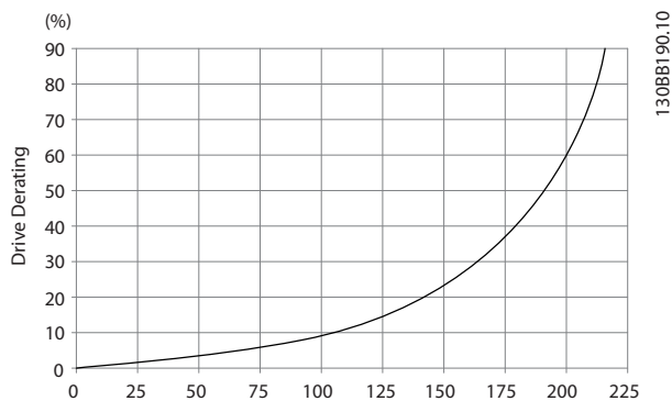
图 4.24 F 机架的降容与 降容 变频器气流: 580 cfm (985 m 3 /h)
