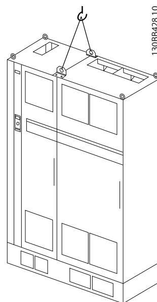
图 4.5 机架规格 F18 的建议起吊方法 - 变频器单元。
