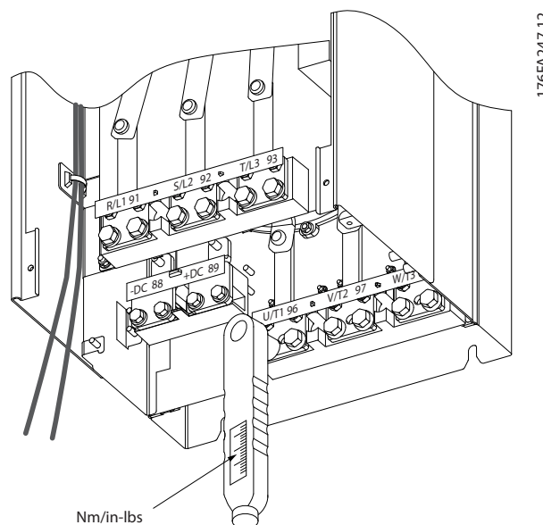
图 4.37 总是使用转矩扳手来拧紧螺栓。
