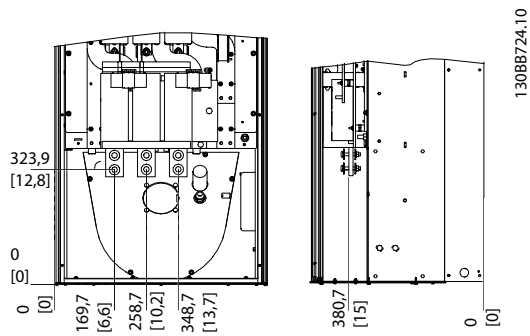
图 4.14 端子位置 E9 - 变频器
