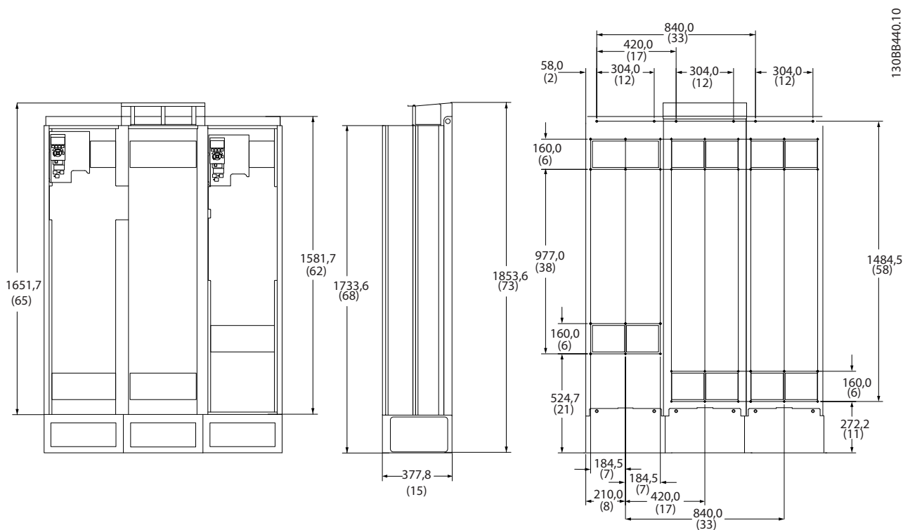
图 4.6 机架规格 D13
