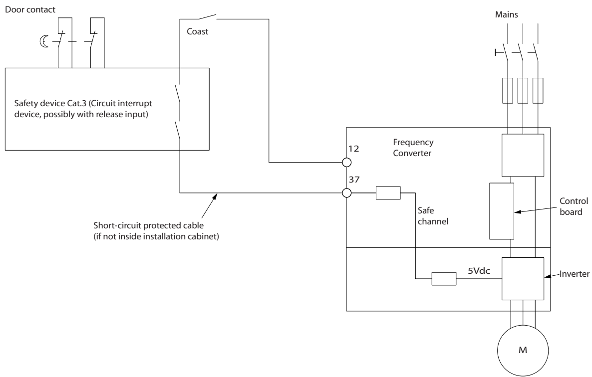
图 2.2 符合停止类别 0 (EN 60204-1) 及安全类别 3 (EN 954-1) 要求的安装要点图示。
