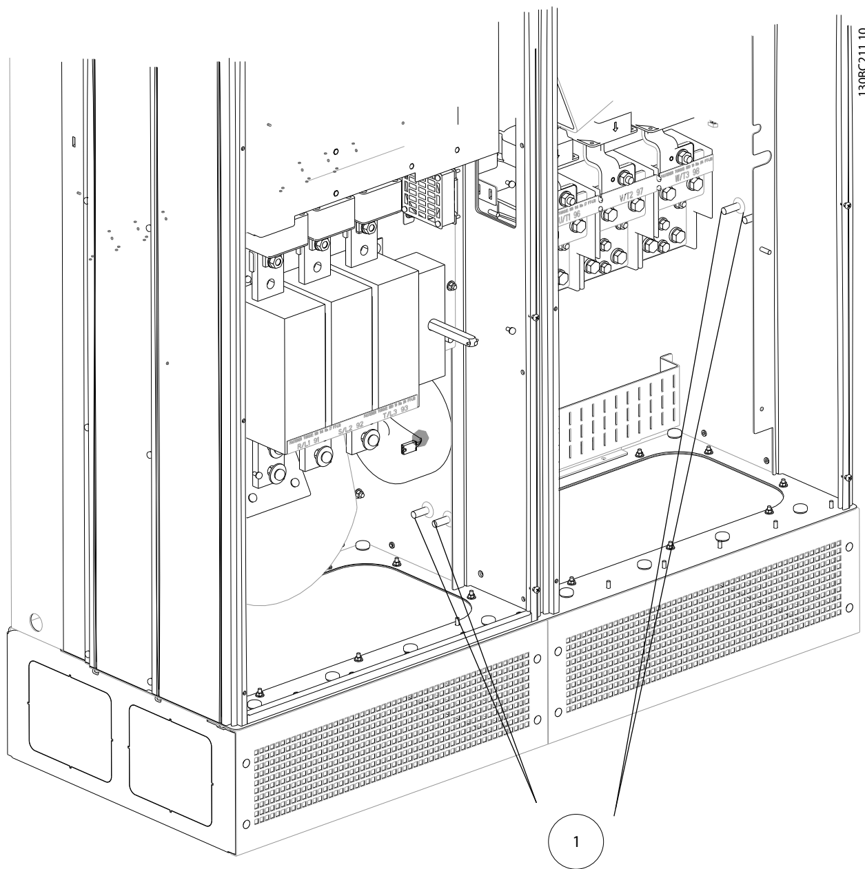
图 4.33 接地端子位置
