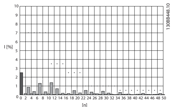
图 3.2 变频器主电源端子处的通常谐波频谱和 THD 值 n = 谐波次数 ◇.....IEEE519 ( I_{sc}/I_l > 20 ) 规定的单个谐波极限
