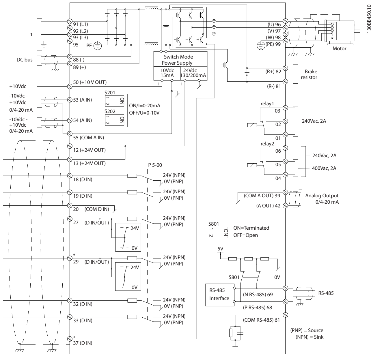
图 4.40 图中显示了不带选件时的所有电气端子。
