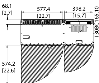
图 4.10 IP21/IP54 型机箱、D13 规格机架的前方空间。
