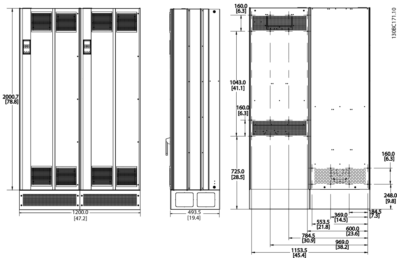
图 4.7 机架规格 E9
