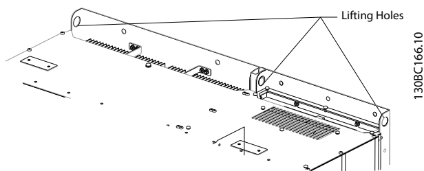
图 4.2 机架规格 D13 的建议起吊方法
