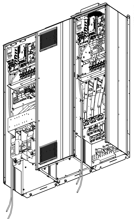
Ilustracja 4.38 Trasa okablowania karty sterującej dla D13
