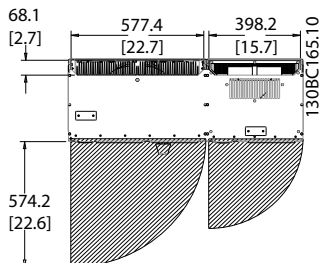
Ilustracja 4.10 Przestrzeń przed typem obudowy IP21/IP54, wymiar ramy D13.
