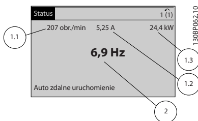
Ilustracja 5.3 Wyświetlacz statusu II - Zmienne parametry pracy
