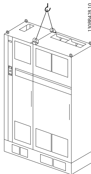
Ilustracja 4.5 Zalecana metoda podnoszenia, wymiar ramy F18 - sekcja przetwornicy.
