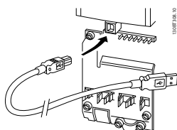
Ilustracja 5.9 Informacje o połączeniach przewodów sterowniczych, patrz 4.8.1 Instalacja elektryczna, przewody sterownicze .
