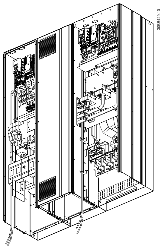
Ilustracja 4.39 Trasa okablowania karty sterującej dla E9
