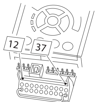
Ilustracja 2.1 Założyć mostek (zworkę) między zaciskami 37 i 24 V DC.
