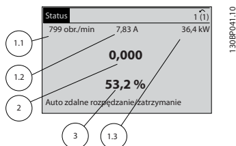
Ilustracja 5.2 Wyświetlacz statusu I - Zmienne parametry pracy
