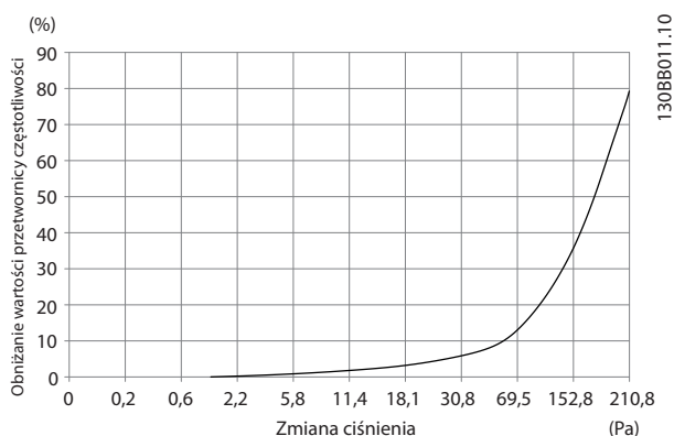
Ilustracja 4.23 Obniżanie wartości znamionowych ramy E w funkcji zmiany ciśnienia (duży wentylator), P355-P450 Przepływ powietrza przez przetwornicę: 1445 m 3 /h (850 cfm)
