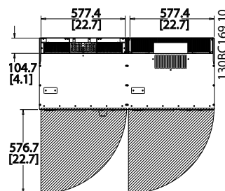
Ilustracja 4.11 Przestrzeń przed typem obudowy IP21/IP54, wymiar ramy E9.
