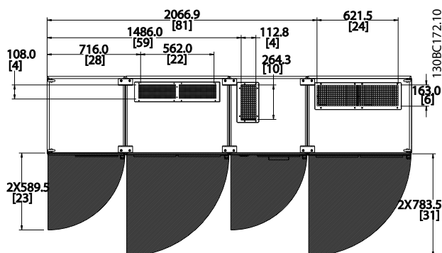
Ilustracja 4.12 Przestrzeń przed typem obudowy IP21/IP54, wymiar ramy F18.
