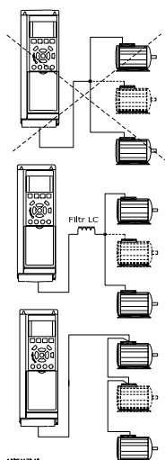
Ilustracja 4.41 Montaż z kablami podłączonymi wspólnie
