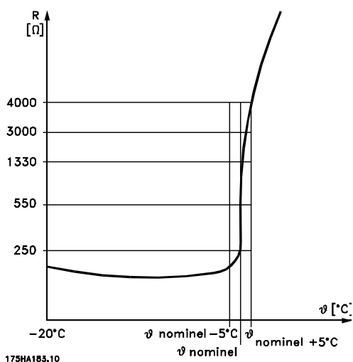
Ilustracja 6.1 Profil PTC
