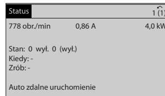
Ilustracja 5.4 Wyświetlacz statusu III - Zmienne parametry pracy
