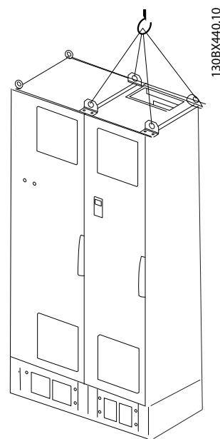
Ilustracja 4.4 Zalecana metoda podnoszenia, wymiar ramy F18 - sekcja filtra.
