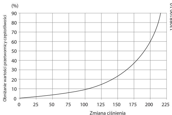
Ilustracja 4.24 Obniżanie wartości znamionowych ramy F w funkcji zmiany ciśnienia Przepływ powietrza przez przetwornicę: 985 m 3 /h (580 cfm)
