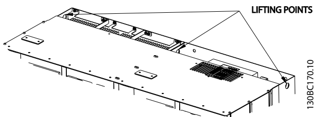
Ilustracja 4.3 Zalecana metoda podnoszenia, wymiar ramy E9.
