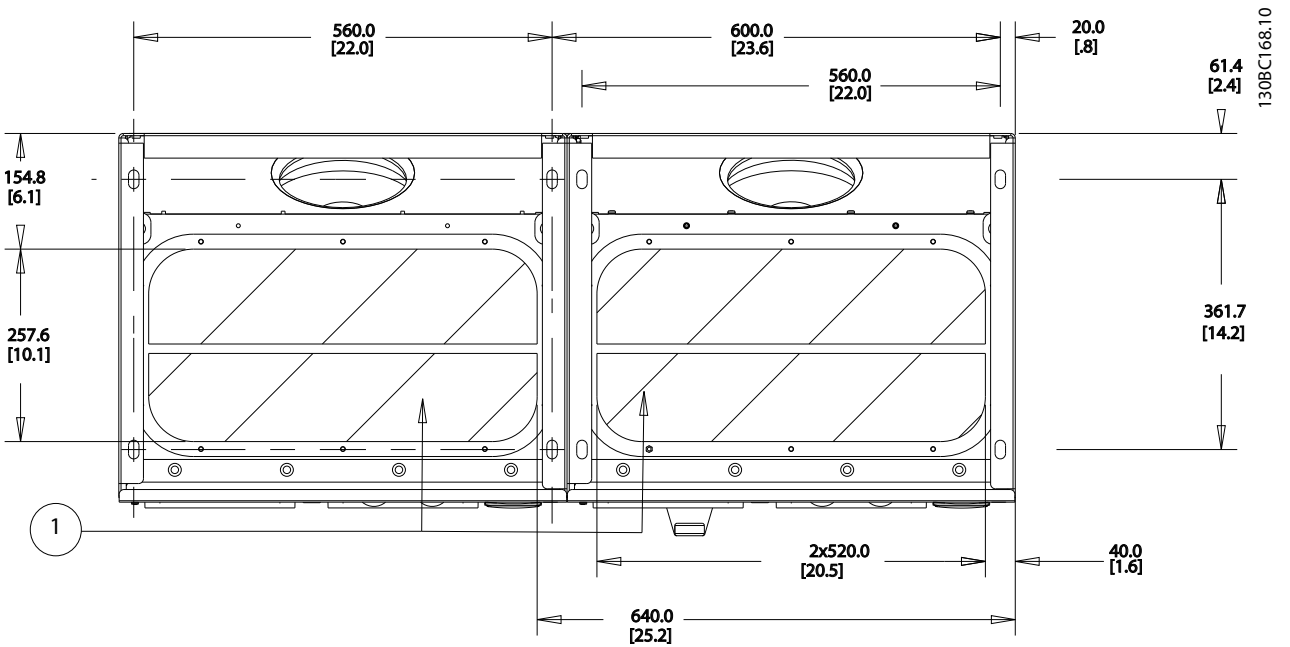
Ilustracja 4.27 Wymiar ramy E9
