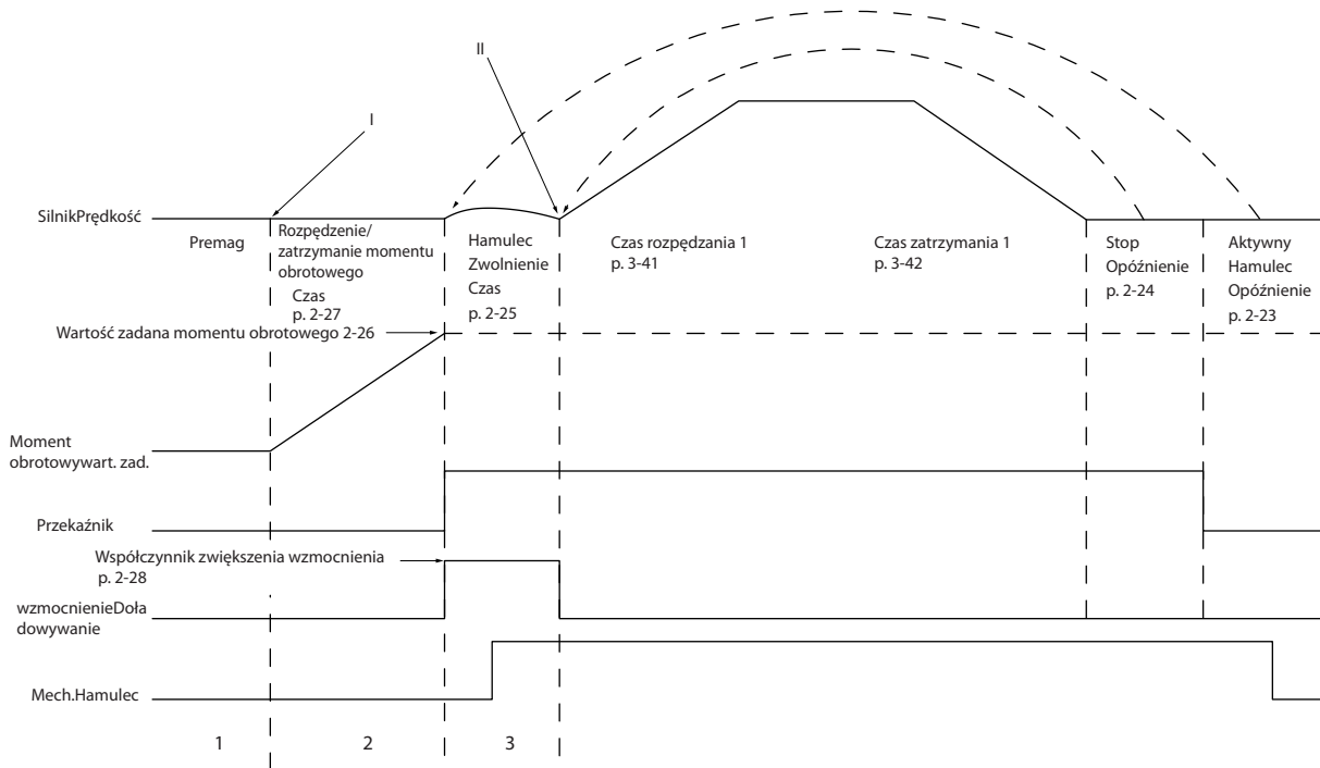
Ilustracja 6.4 Sekwencja zwolnienia hamulca dla sterowania hamulca mechanicznego
