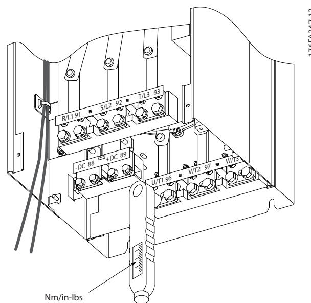
Ilustracja 4.37 Śruby należy zawsze dokręcać za pomocą klucza dynamometrycznego.
