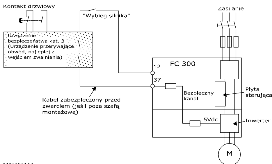
Ilustracja 2.2 Podstawowe aspekty instalacji, umożliwiające uzyskanie Kategorii zatrzymania 0 (EN 60204-1) z Kategorią bezpieczeństwa 3 (EN 954-1).
