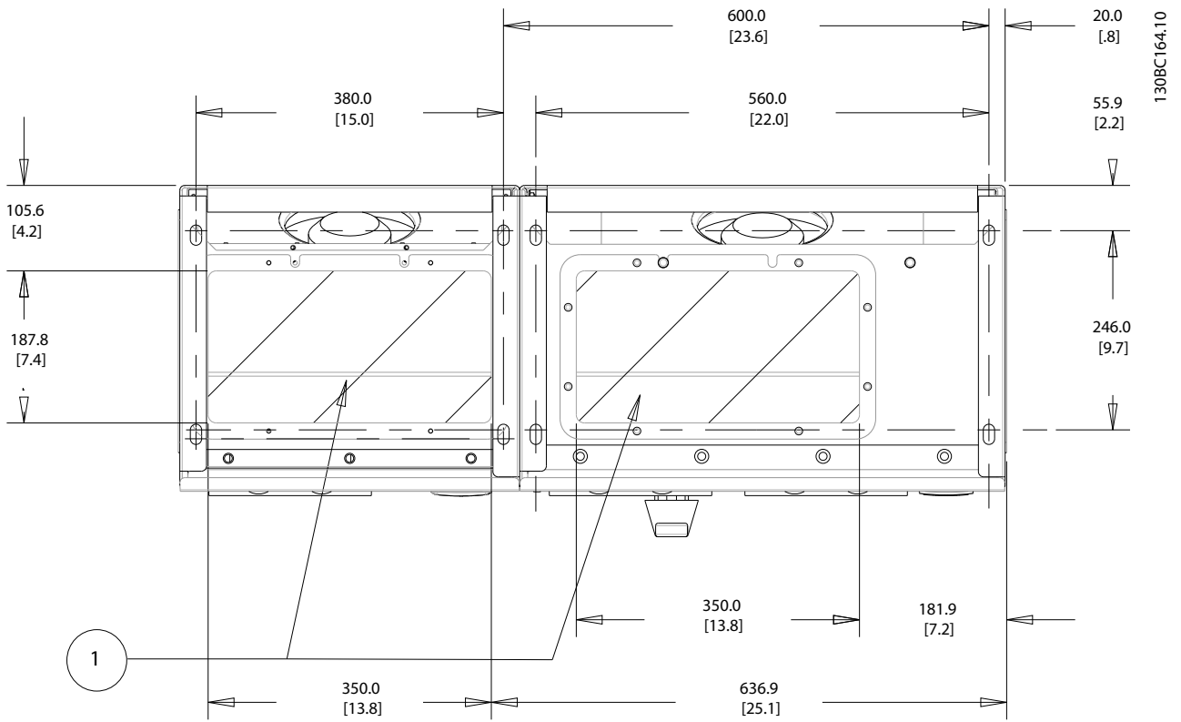
Ilustracja 4.26 Wymiar ramy D13
