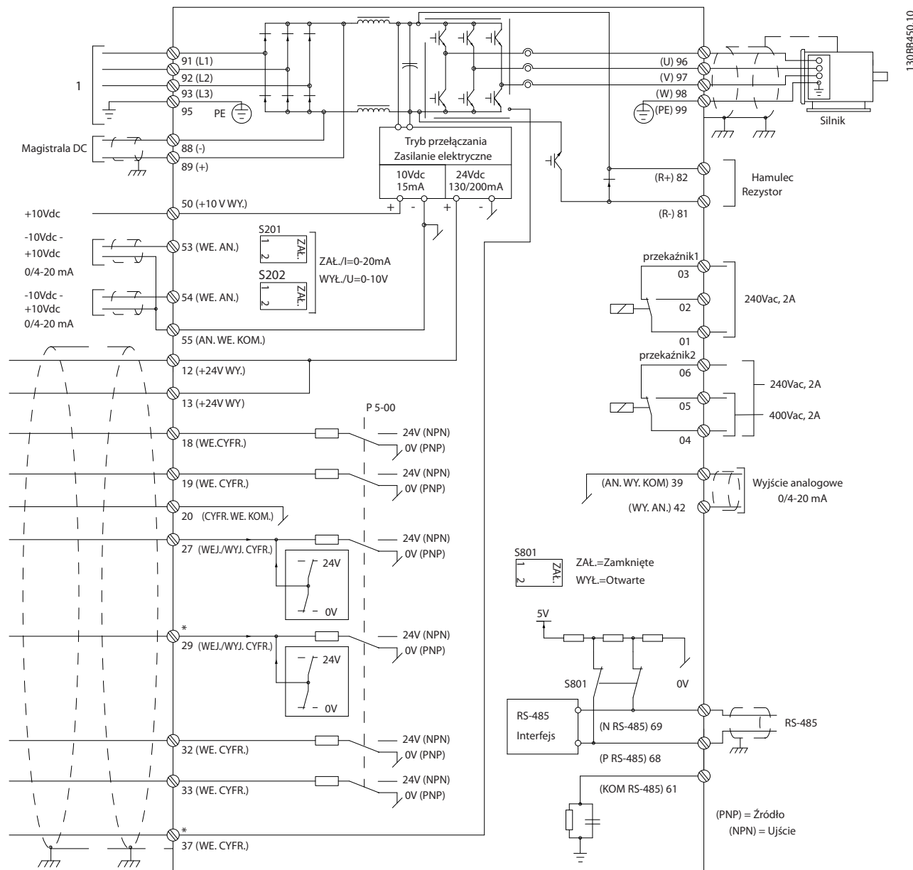
Ilustracja 4.40 Schemat wszystkich zacisków elektrycznych bez opcji.
