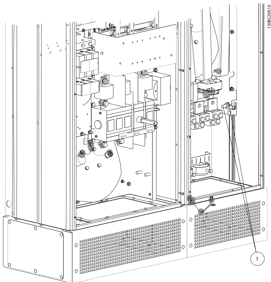
Ilustracja 4.31 Położenie zacisków uziemienia
