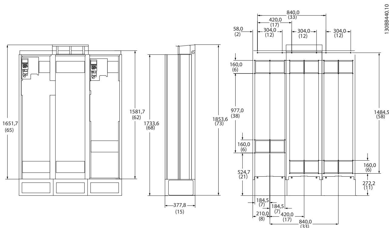
Ilustracja 4.6 Wymiar ramy D13
