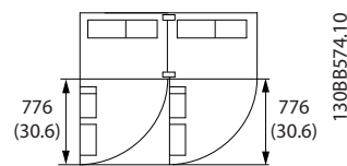
Рисунок 3.6 Пространство перед корпусом IP21/IP54, типоразмер F10
