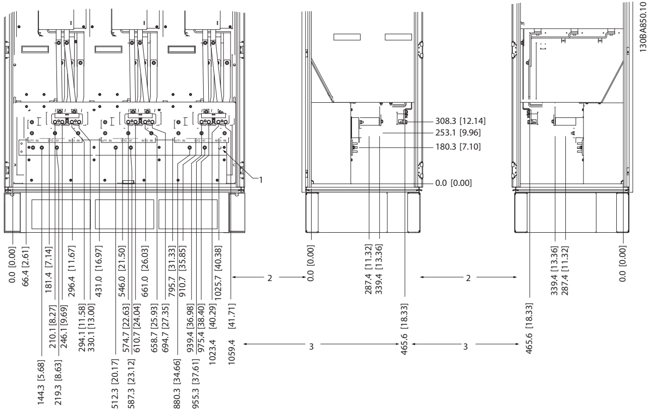
Рисунок 3.13 Расположение клемм — шкаф инвертора (вид спереди, слева и справа). Плата уплотнений расположена на 42 мм ниже уровня 0.
