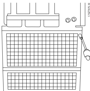
Рисунок 3.34 Монтаж экрана EMC (ЭМС).
