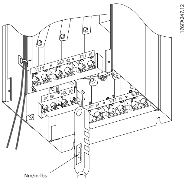
Рисунок 3.32 Для затягивания болтов всегда применяйте динамометрический ключ.
