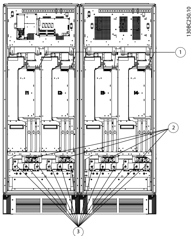
Рисунок 3.29 Шкаф инвертора, типоразмер F14
