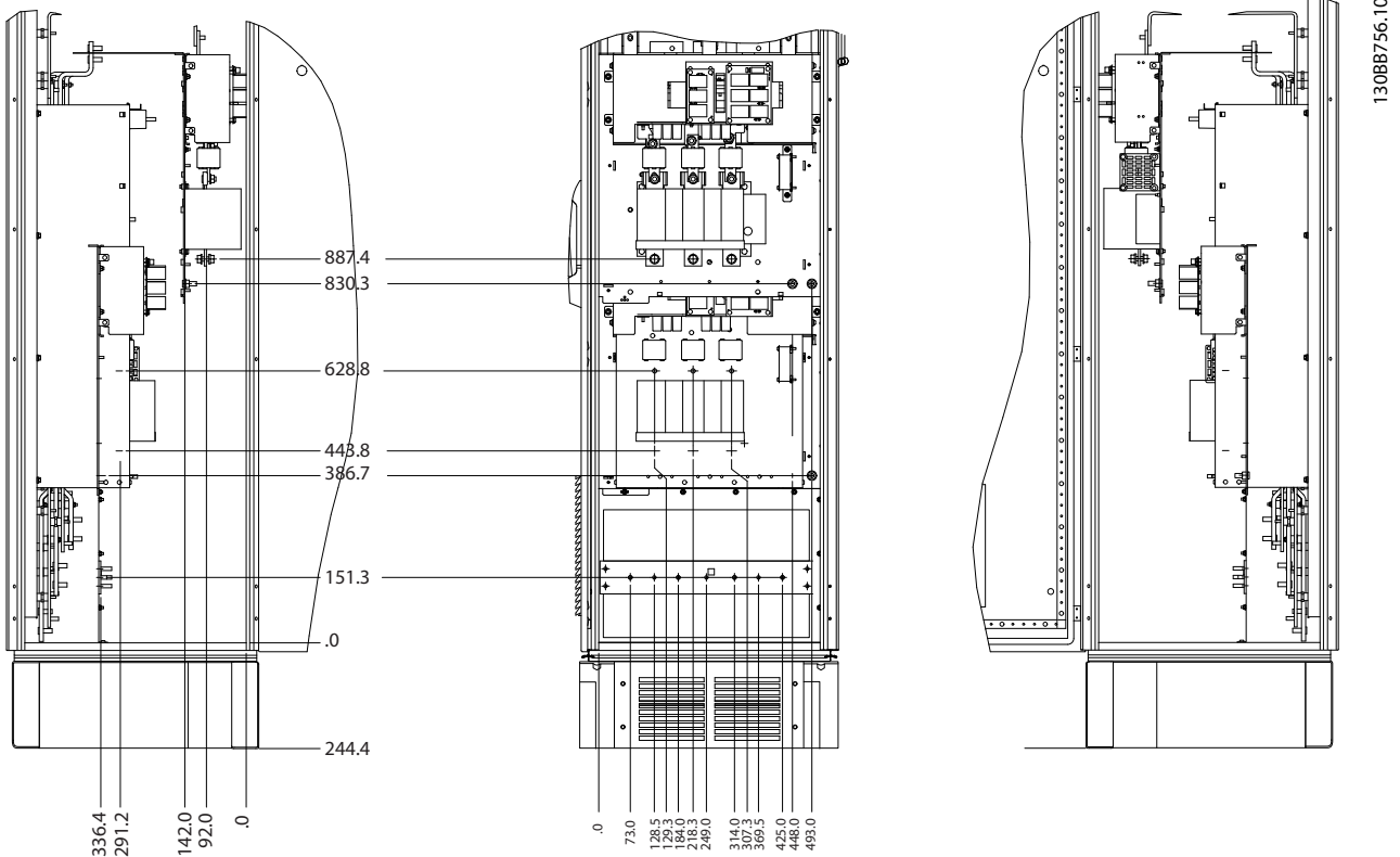
Рисунок 3.17 Расположение клемм — шкаф дополнительных устройств (вид слева, спереди и справа).
