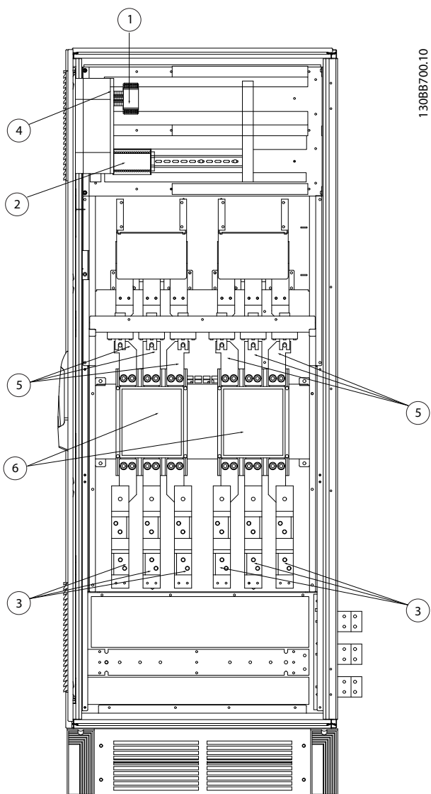
Рисунок 3.31 Дополнительный шкаф, типоразмеры F11 и F13
