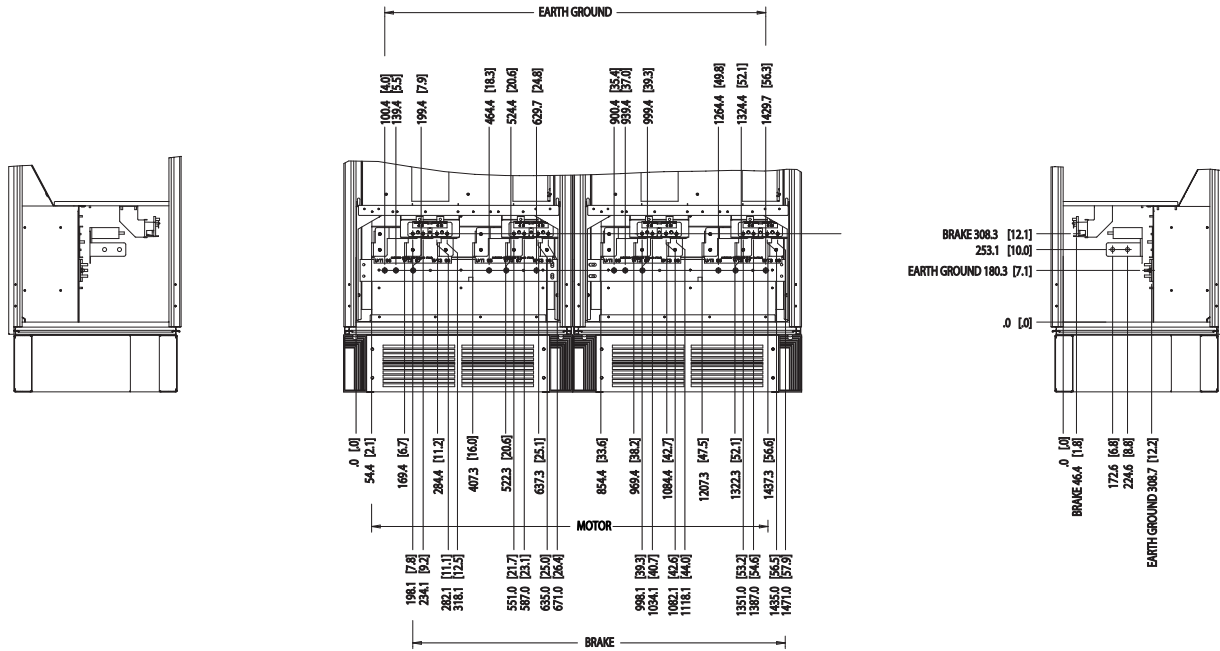
Рисунок 3.14 Расположение клемм — шкаф инвертора (вид спереди, слева и справа). Плата уплотнений расположена на 42 мм ниже уровня 0.
