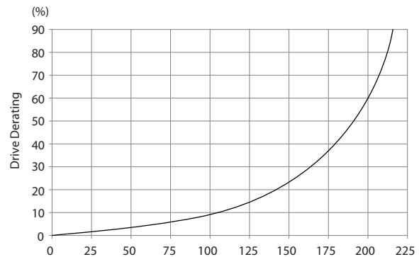
Рисунок 3.19 Корпус F: снижение номинальных параметров относительно изменения давления (Па)
