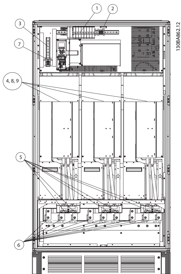
Рисунок 3.28 Шкаф инвертора, типоразмеры F12 и F13
