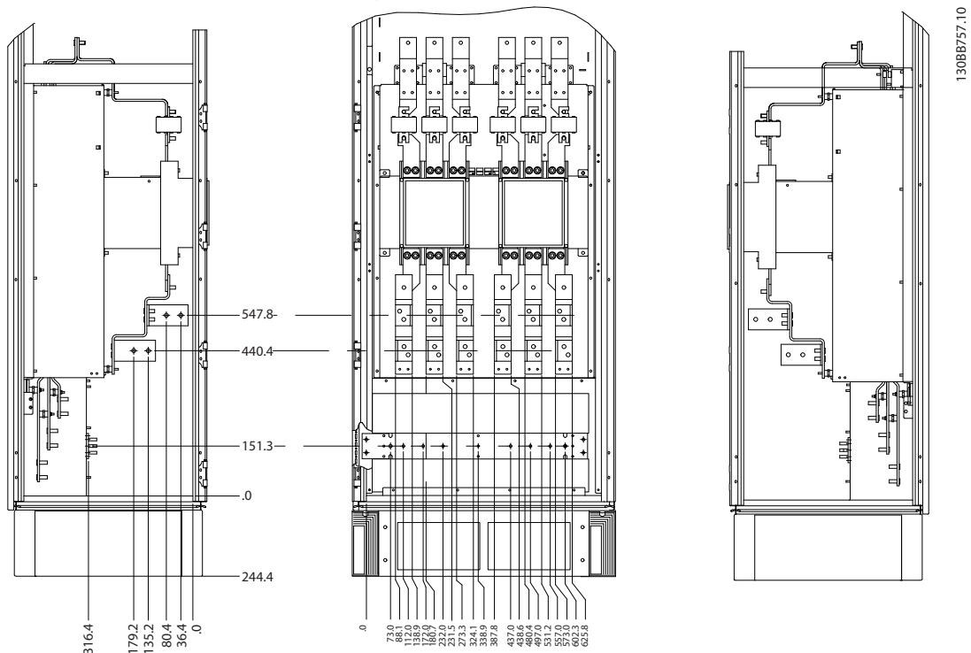
Рисунок 3.18 Расположение клемм — шкаф дополнительных устройств (вид слева, спереди и справа).
