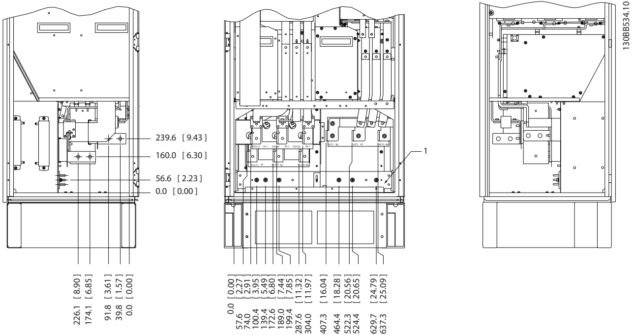
Рисунок 3.11 Расположение клемм — шкаф инвертора и выпрямителя — F8 и F9 (вид спереди, слева и справа). Плата уплотнений расположена на 42 мм ниже уровня 0.
