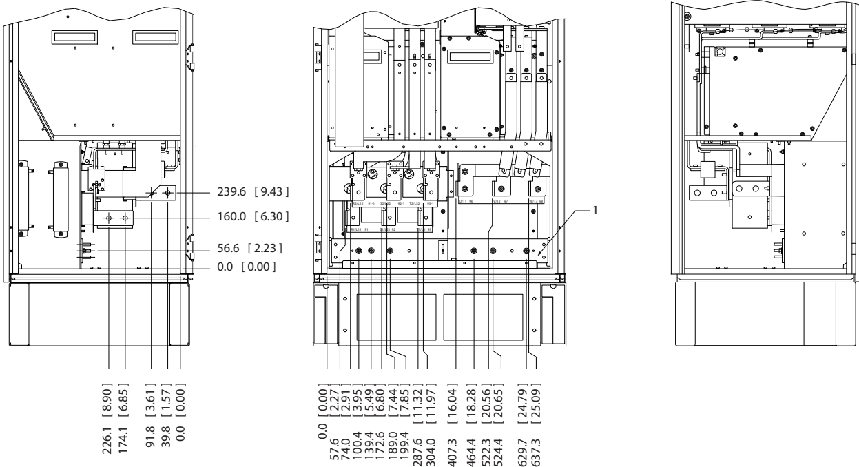
Рисунок 3.15 Расположение клемм — выпрямитель (вид слева, спереди и справа). Плата уплотнений расположена на 42 мм ниже уровня 0.
