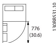
Рисунок 3.4 Пространство перед корпусом IP21/IP54, типоразмер F8
