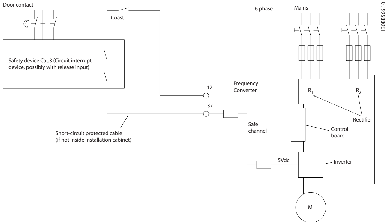
Рисунок 2.2 Основные особенности установки, необходимые для осуществления останова категории 0 (EN 60204-1), отвечающего требованиям категории безопасности 3 (EN 954-1).
