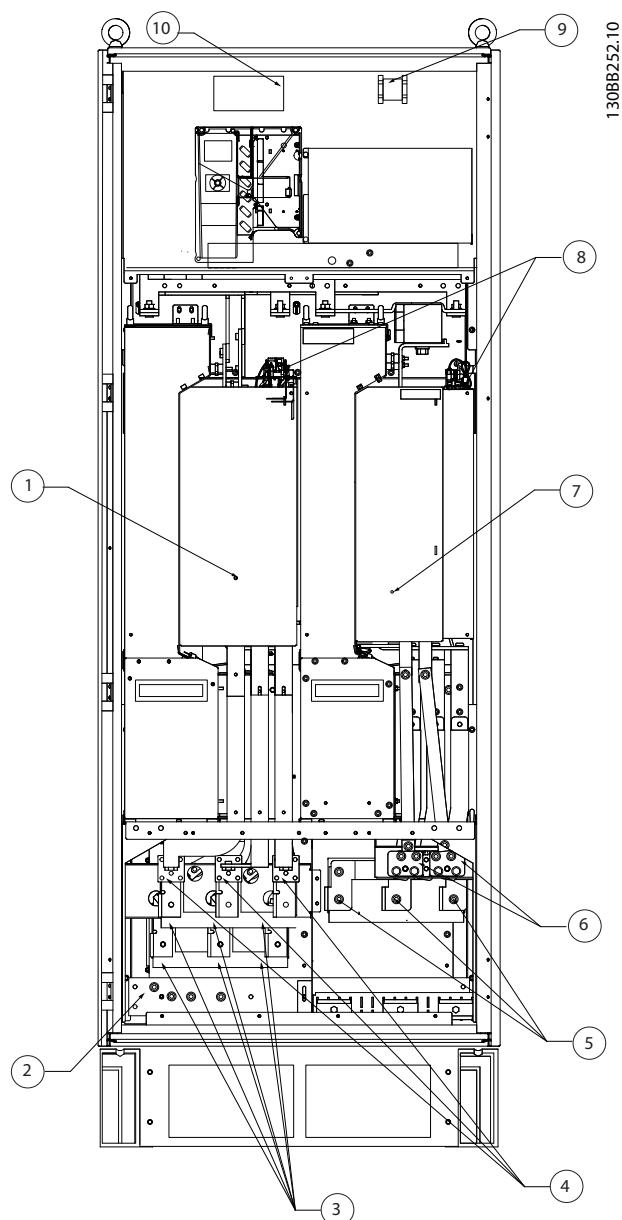
Рисунок 3.24 Шкаф выпрямителя и инвертора, типоразмеры F8 и F9
