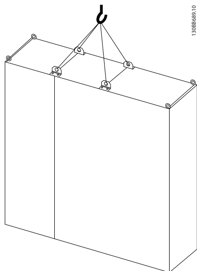
Рисунок 3.3 Рекомендуемый метод подъема, типоразмер F11/F12/F13/F14.
