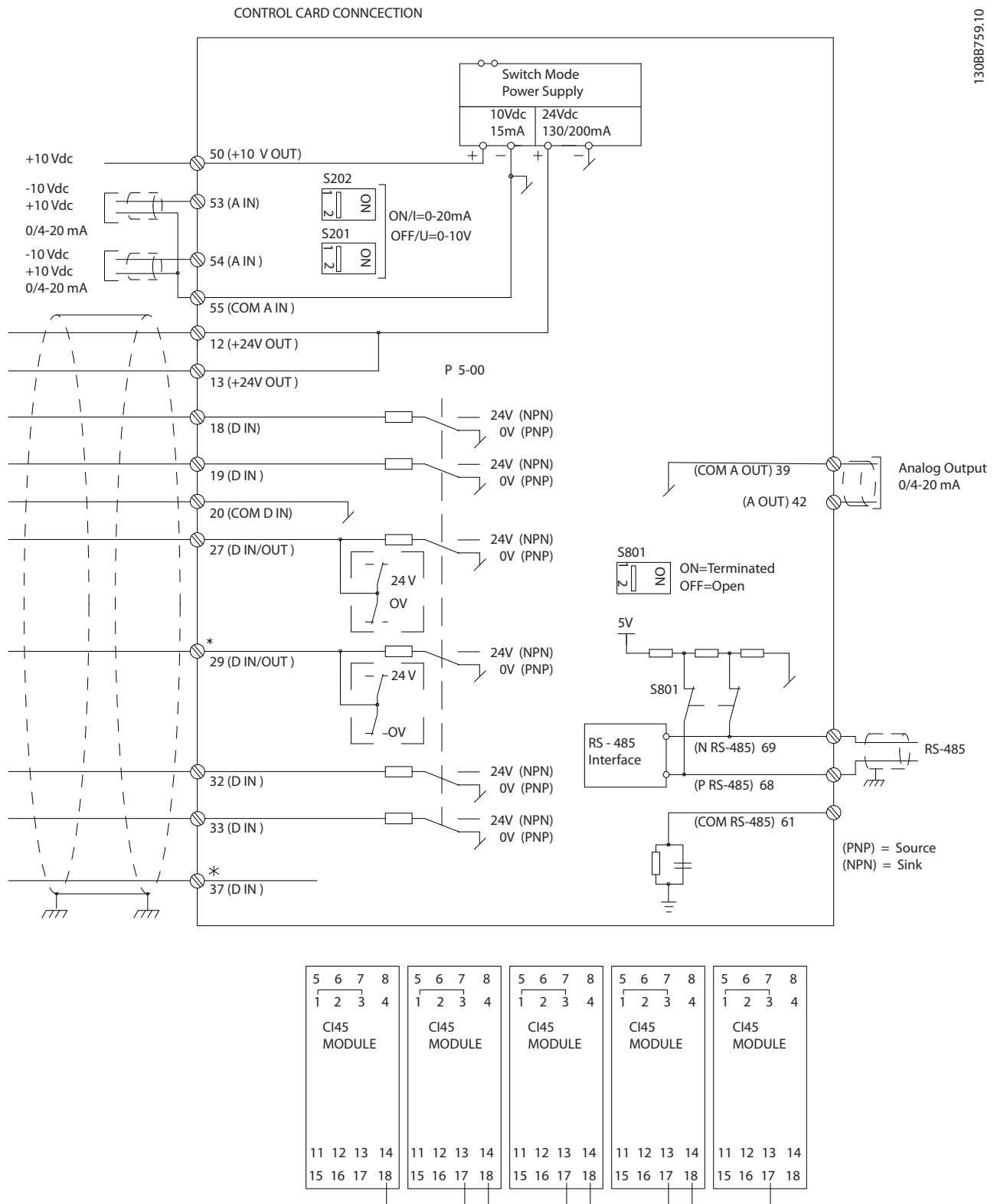
Bild 3.50 Kopplingschema
