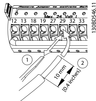
Kuva 3.49 Ohjaukkaapelin kytkentä
