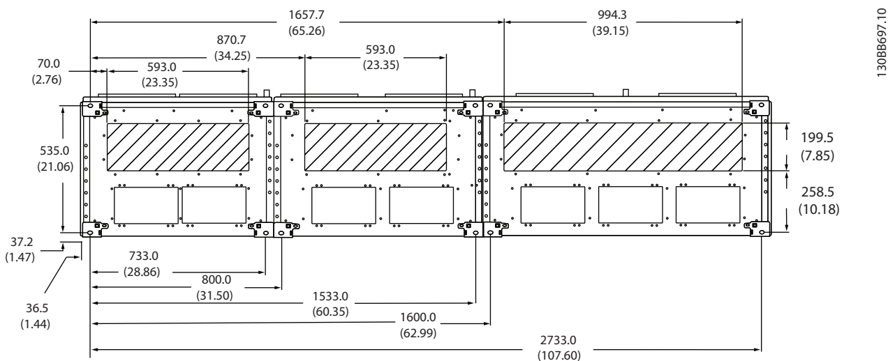
图 3.29 F13, 电缆入口 (从变频器底部看)
