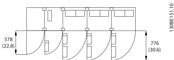
图 3.12 F15 机箱规格前方的空间
