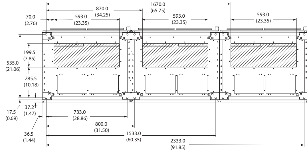
图 3.30 F14, 电缆入口 (从变频器底部看)
