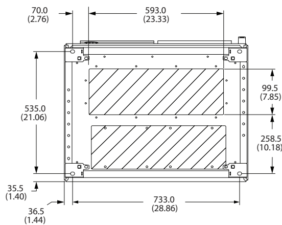
图 3.24 F8，电缆入口（从变频器底部看）
