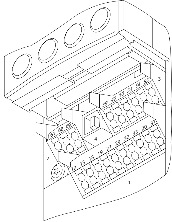
Çizim 2.29 Kontrol Terminali Yerleri
