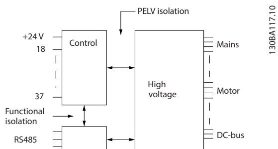
Εικόνα 10.1 Μόνωση PELV
