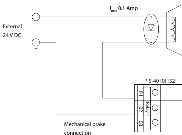
Slika 8.8 Konfiguracija ožičenja za ograničenje momenta i zaustavljanje
