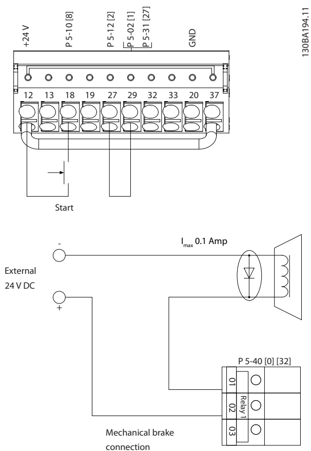
图 8.8 用于转矩和停止极限的接线配置
