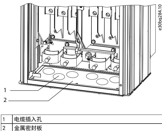
图 4.4 金属密封板中的电缆开口
