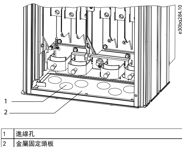
圖 4.4 金屬片固定頭板內的電纜線開口
