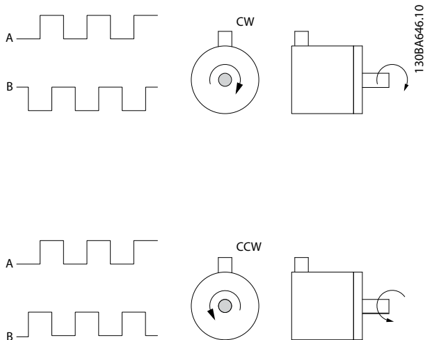
圖 8.6 決定編碼器轉向
