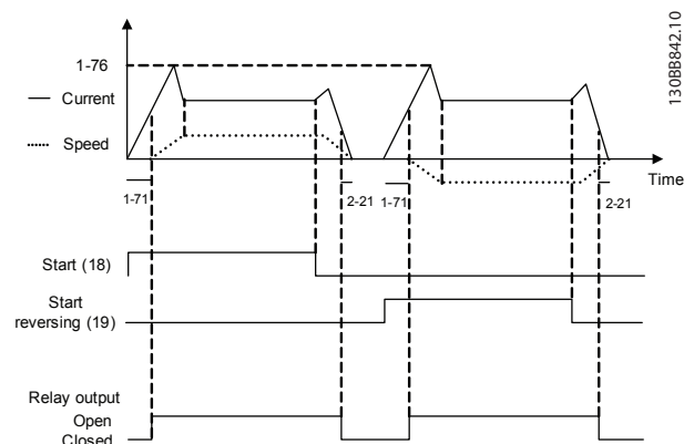
圖 8.5 機械煞車控制
