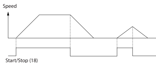
圖 8.2 啟動/停機指令 (含安全轉矩關閉功能)
