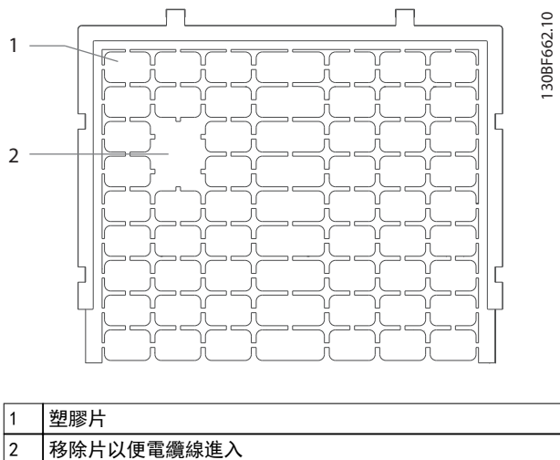
圖 4.5 塑膠製固定頭板內的電纜線開口
