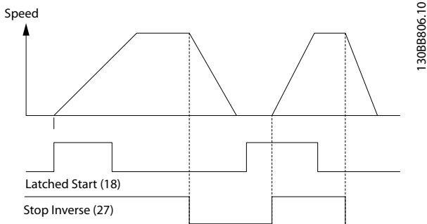
圖 8.3 脈衝啟動/停止反邏輯
