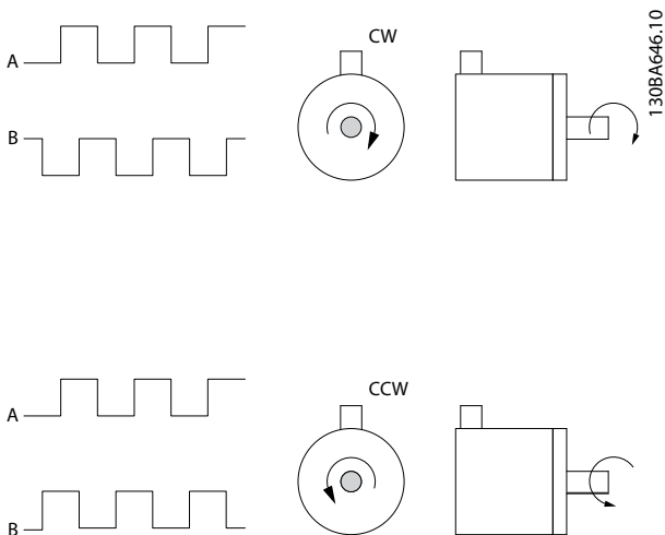
Ilustrația 8.6 Stabilirea direcției encoderului
