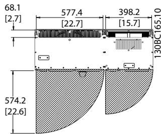
Illustration 4.10 Tila IP21/IP54-kotelointityypin edessä, D13-kehyskoko.
