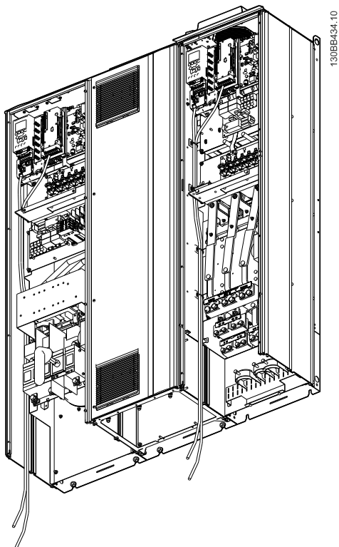
Illustration 4.32 Ohjaukkaapelin johdotusreitit mallille D13
